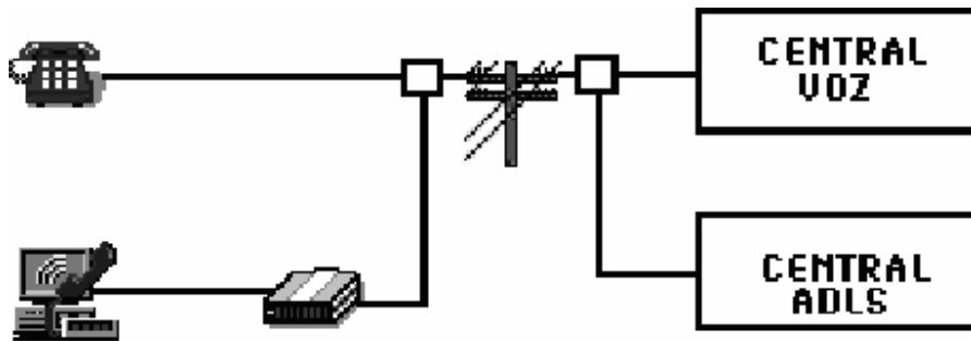
Figura 3.8 Filtros separadores.
