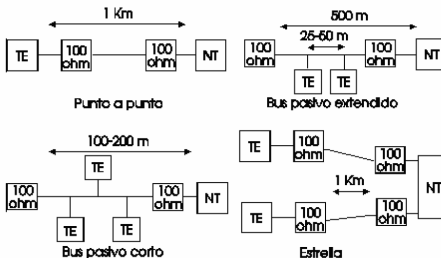
Figura 1.14 Configuraciones básicas de cableado.
