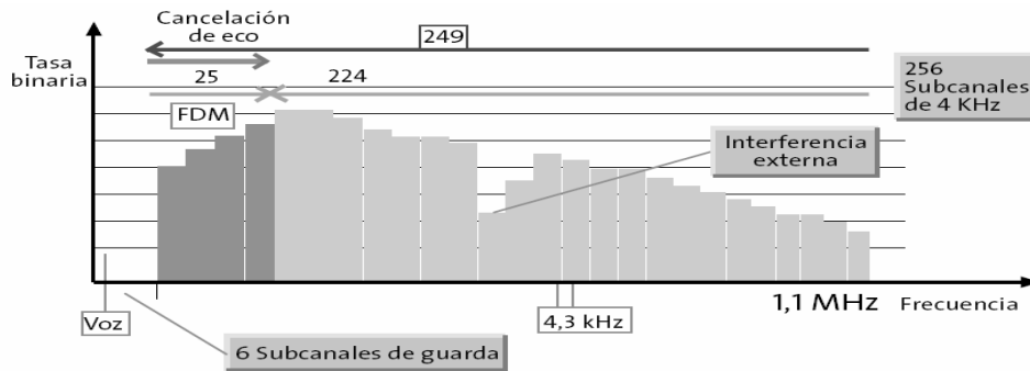
Figura 3.6 Espectro resultante de la modulación DTM.
