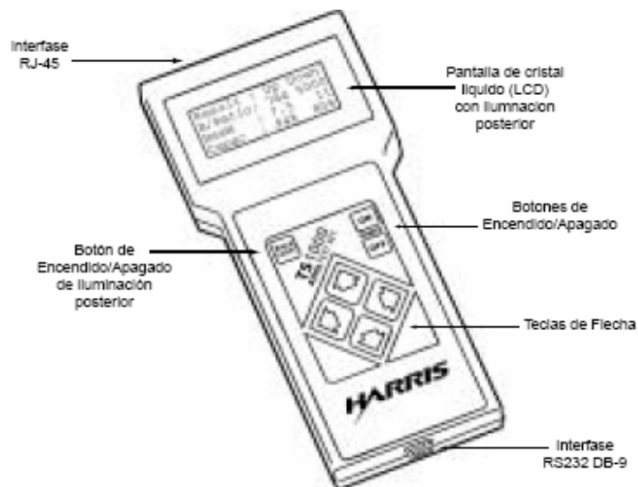
Figura 4.18 Equipo TS-1000
