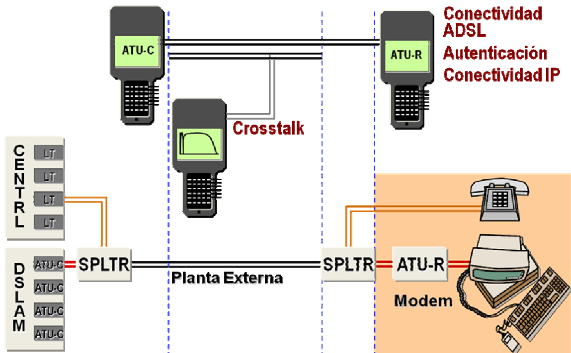
Figura 4.3 Emulación ADSL.
