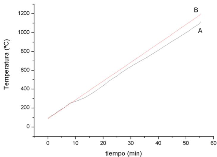
Figura 24. Perfil de temperatura de corridas directas en la muffla, a 60 min de calentamiento donde A es la temperatura del sensor y B es la temperatura del programa del horno.
