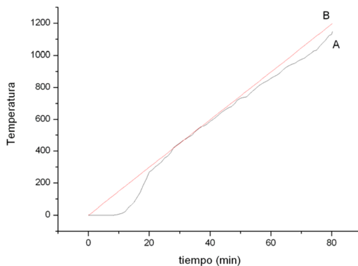
Figura 25. Perfil de temperatura de corridas directas en la muffla, a 90 min de calentamiento donde A es la temperatura del sensor y B es la temperatura del programa del horno.
