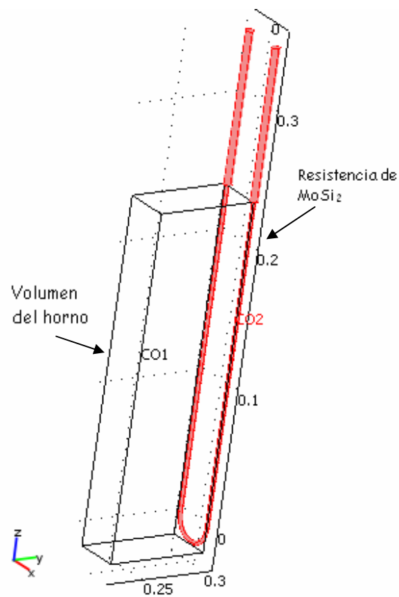
Figura 12. Vista tridimensional de la resistencia y volumen del horno
