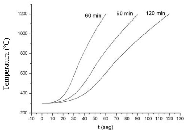
Figura 27. Predicción de distribución de Temperatura a 60, 90 y 120 min en horno muffle, COMSOL 3.2.
