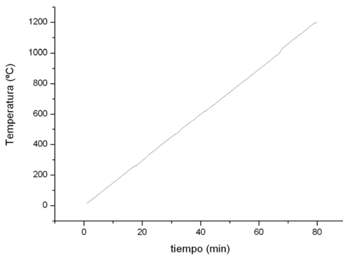
Figura 32. Predicción de distribución de Temperatura 90 min de calentamiento en horno muffle, Programa en Visual Basic.
