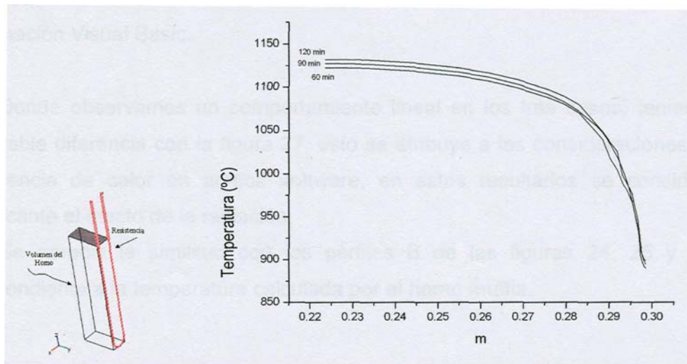
Figura 29. Corridas en COMSOL3.2, perfiles de temperatura respecto a la longitud superior del horno a los tiempo de 60, 90 y 120 min de calentamiento.
