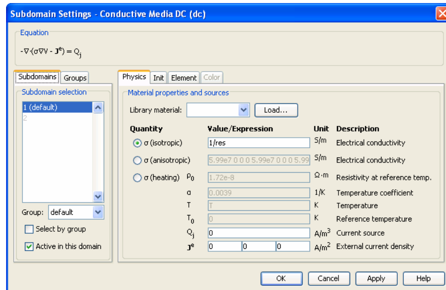
Figura 15. Propiedad eléctrica de la resistencia.
