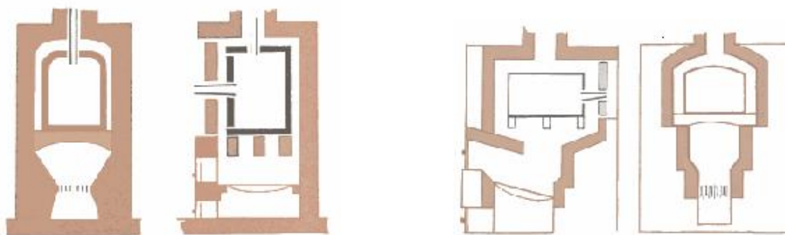
Figura 7. Paredes de los hornos muffla.
