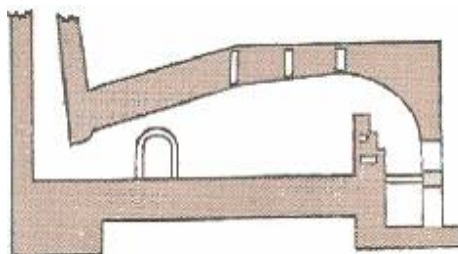
Figura 5. Horno Kasseler
