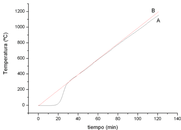
Figura 26. Perfil de temperatura de corridas directas en la muflla, a 120 min de calentamiento donde A es la temperatura del sensor y B es la temperatura del programa del horno.
