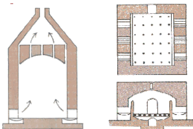
Figura 6. Hornos de cámara de dos pisos
