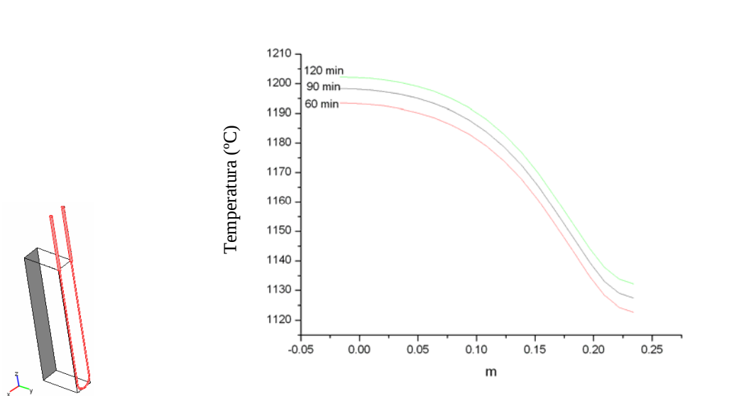
Figura 30. Corridas en COMSOL3.2, perfiles de temperatura respecto a la longitud superior del horno a los tiempo de 60, 90 y 120 min de calentamiento.
