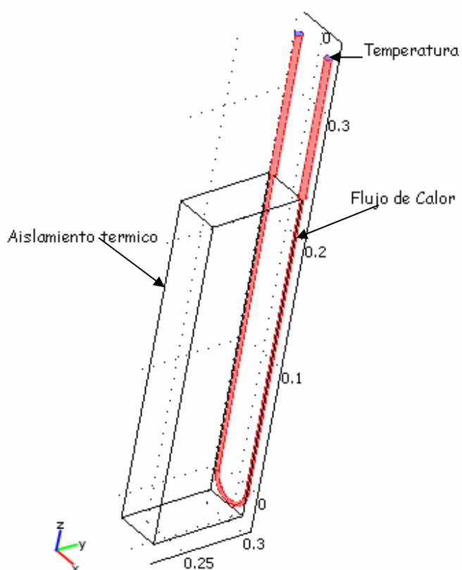
Figura 17. Condiciones límite de la resistencia y volumen de horno (aire), modulo Heat Transfer by Conduction
