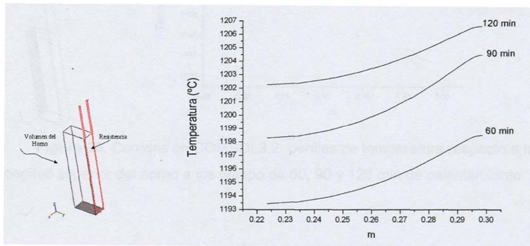
Figura 28. Corridas en COMSOL3.2, perfiles de temperatura respecto a la longitud inferior del horno a los tiempo de 60, 90 y 120 min de calentamiento.
