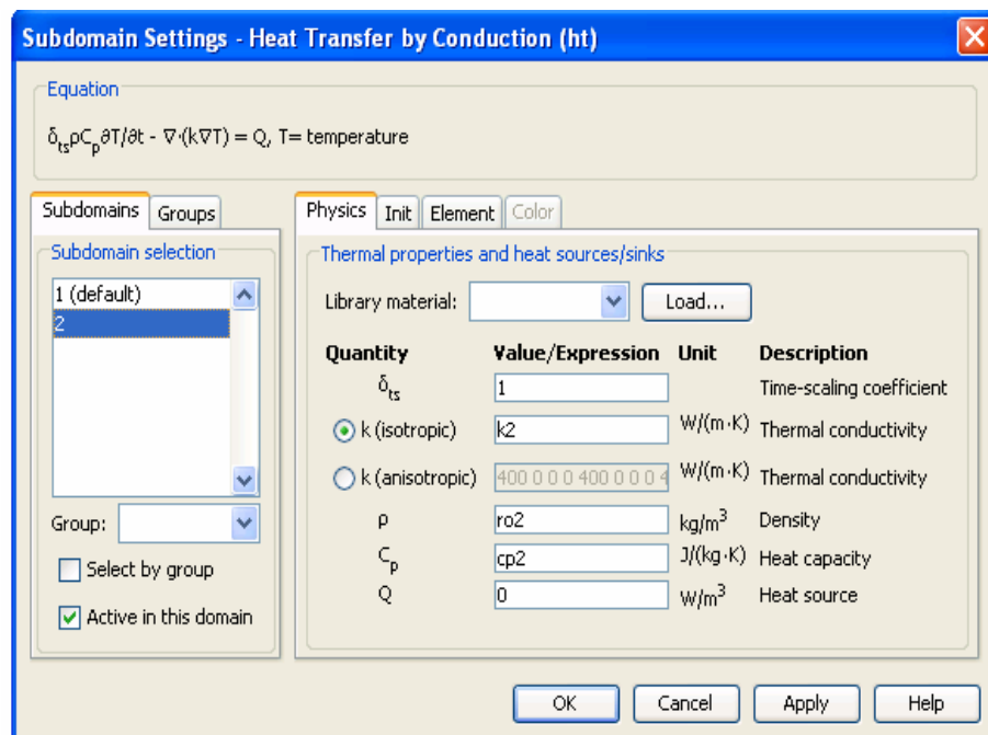
Figura 14. Propiedades físicas del volumen del horno (aire).
