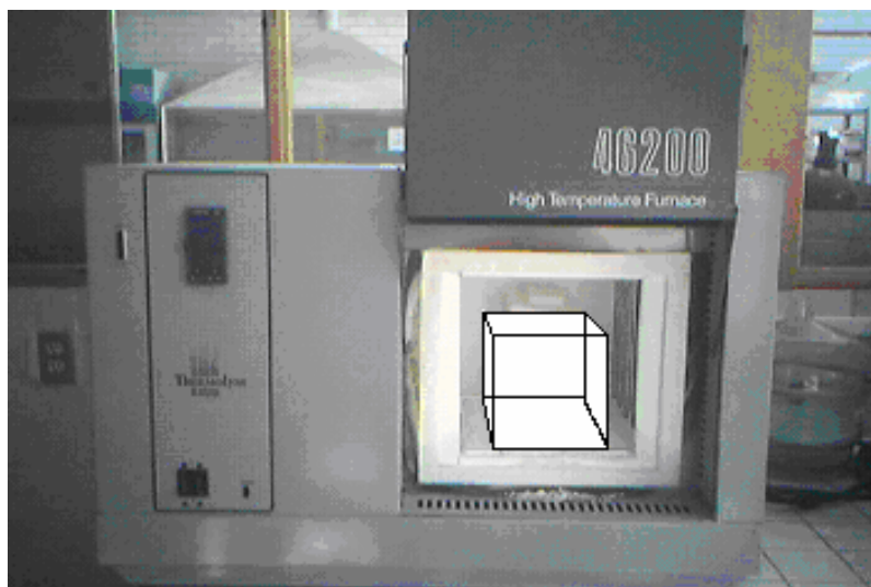
Figura 35. Volumen con temperatura constante para la sinterización de material cerámico muffle thermolyne 46000.
