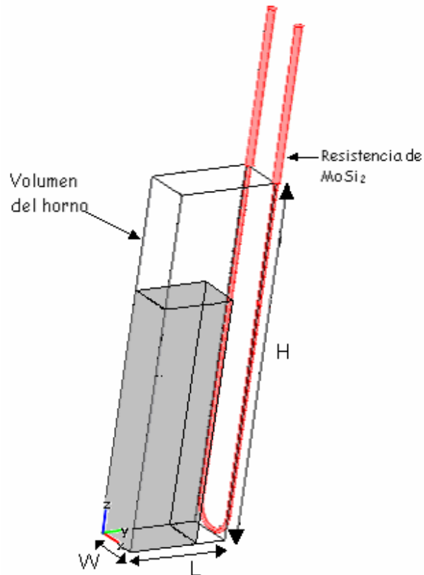
Figura 34. Volumen donde la temperatura es constante
