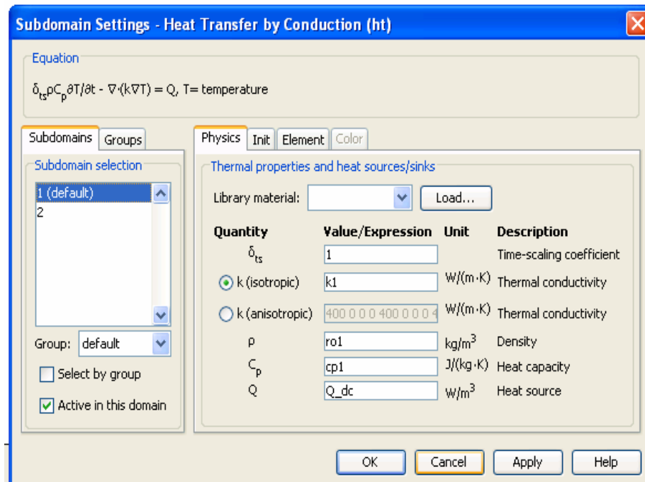
Figura 13. Condiciones físicas de la resistencia.
