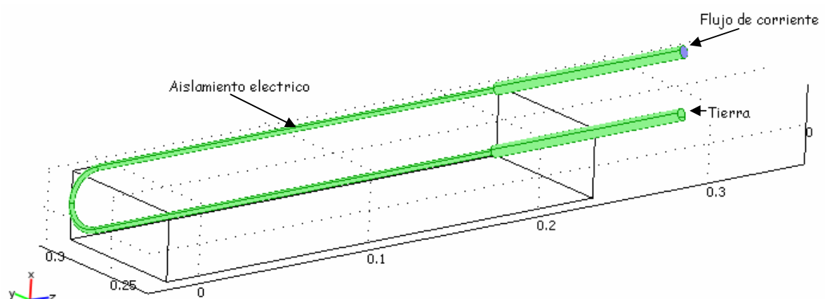
Figura 16. Condiciones límite de la resistencia para el modulo Electro Therma- Joule Heating
