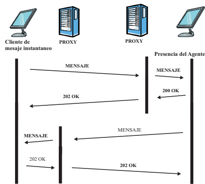
Figura 4.7: Mensajería instantánea SIP
