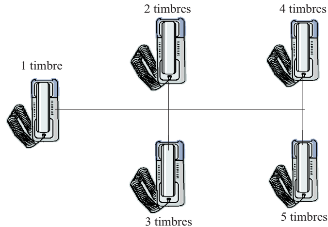
Figura 2.2: Intercomunicador en paralelo
