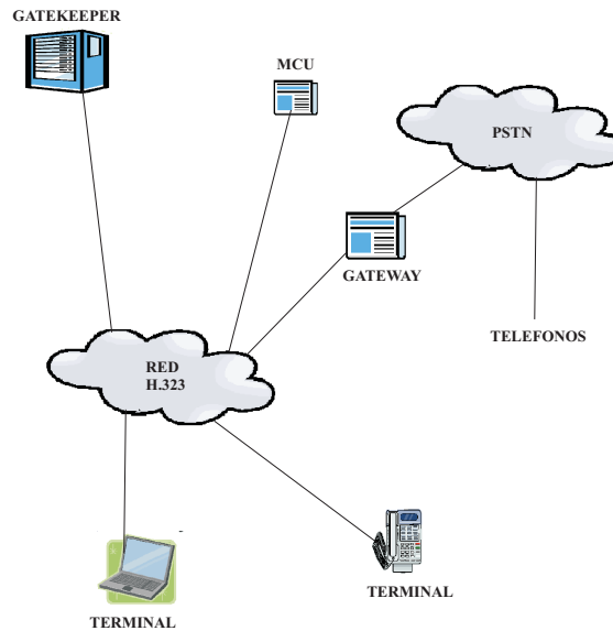
Figura 4.12: Elementos principales de una red H.323
