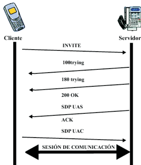
Figura 4.4: INVITE con cuerpo de mensaje
