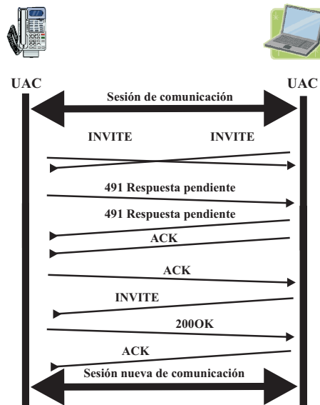
Figura 4.11: Resolución de re-INVITE simultáneas
