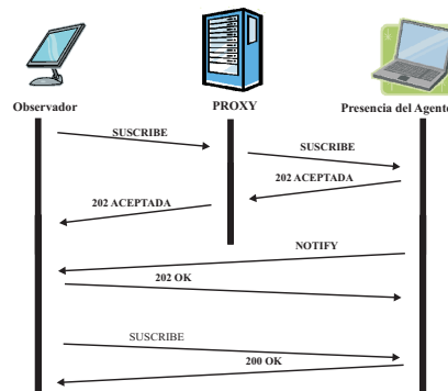
Figura 4.6: Llamada de un SUSCRIBE y NOTIFY
