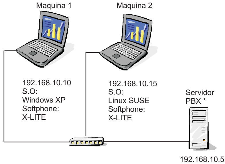
Figura 5.2: Interconexion de clientes SIP Y PBX asterisk en una red local
