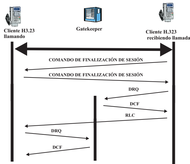
Figura 4.14: Secuencia de terminación de llamada H.323
