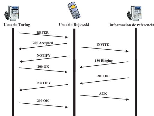
Figura 4.5: Flujo de llamada para una REFER (referencia)
