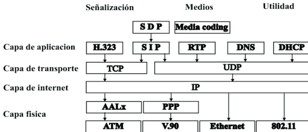
Figura 4.1: Línea de protocolos multimedia de Internet
