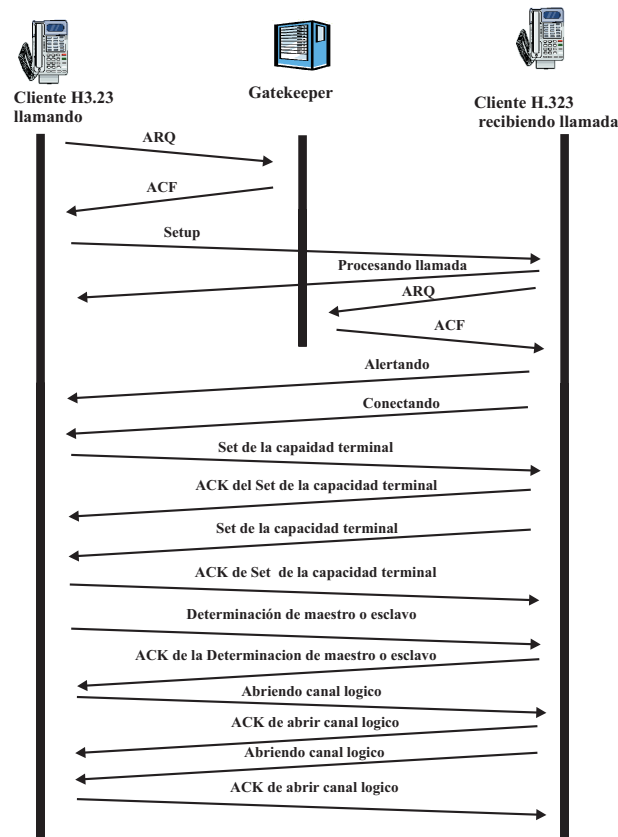
Figura 4.13: Flujo de llamada H.323
