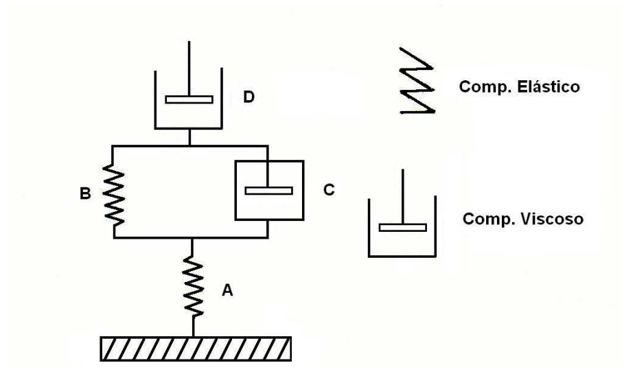
Figura 1. Modelo mecánico para el comportamiento reológico de la masa (Pomeranz, 1977).
