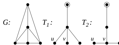
Figura 4.3: Gráfica G junto con dos árboles generadores, uno de los cuales es primero en profundidad.
