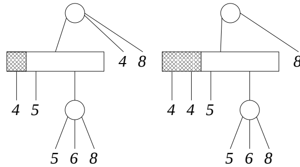
Figura 5.19: Procedimiento para checar planaridad de G (Figura 5.15). Fase 7 y 8.
