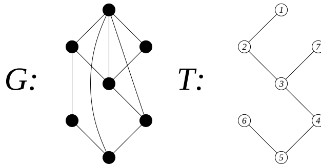
Figura 4.5: Gráficas G y T del ejemplo.
