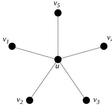
Figura 6.2: El vértice v_i tiene el color c_i
