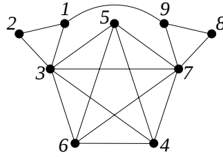
Figura 4.2: Numeración st de una gráfica.
