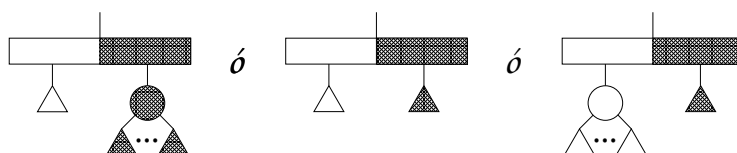
Figura 5.7: Reemplazos alternativos para la plantilla P_3
