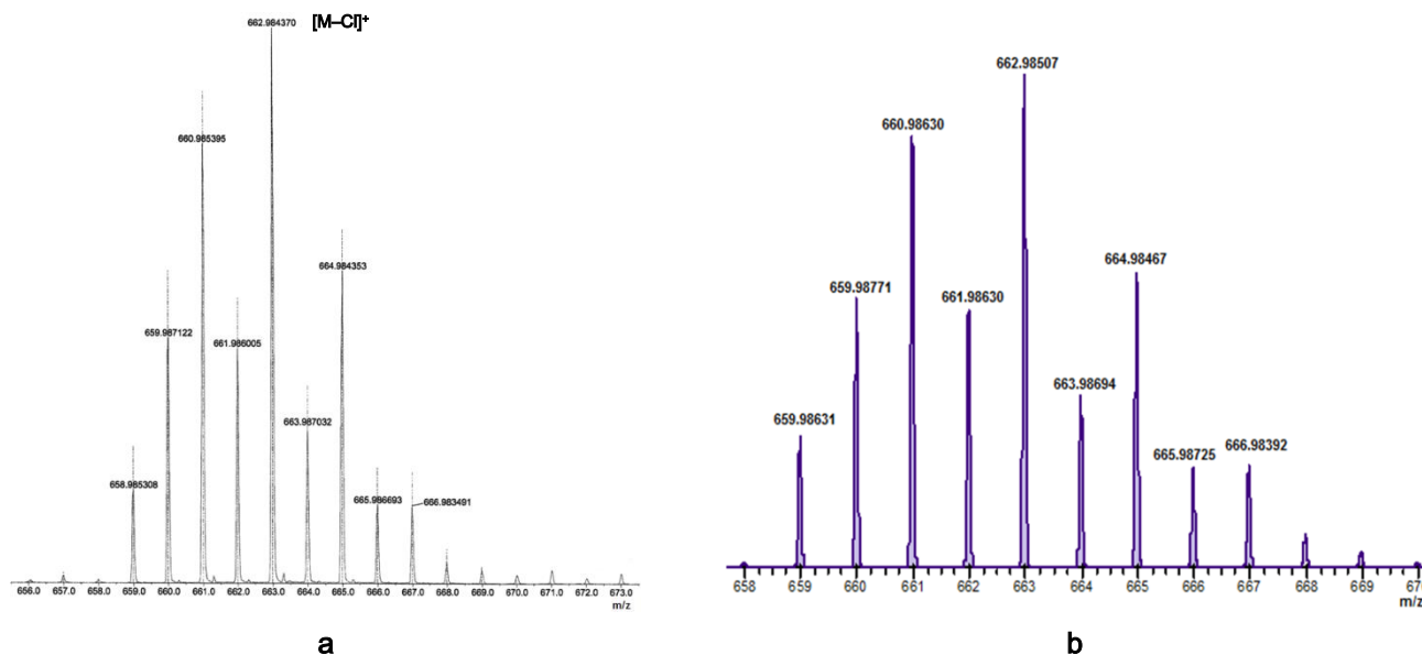
Figura 3.18. Comparación de los picos de masas observado (a) y calculado (b) para el fragmento [M-CI]^+ para el metalomacrocielo 23.
