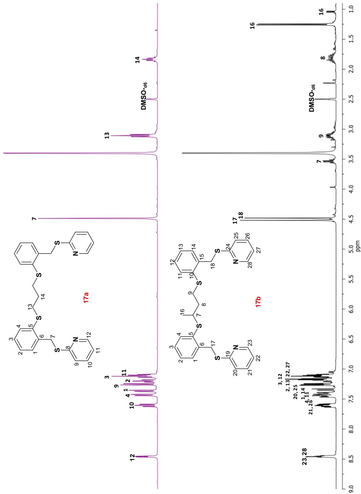
Figura 2.8. Espectros de 1 H a 400 MHz del de los ligantes 17a y 17b en DMSO-d 6 .
