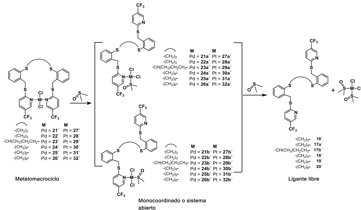
Esquema 3.5. Ruta propuesta para el proceso de desensamble de los metalomacrociclos 21' – 32' .
