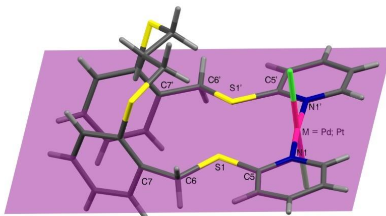
Figura 3.12. Perspectiva del segmento plano presente en el anillo de 18 miembros de los metalomacrociclos 22 y 28 .
