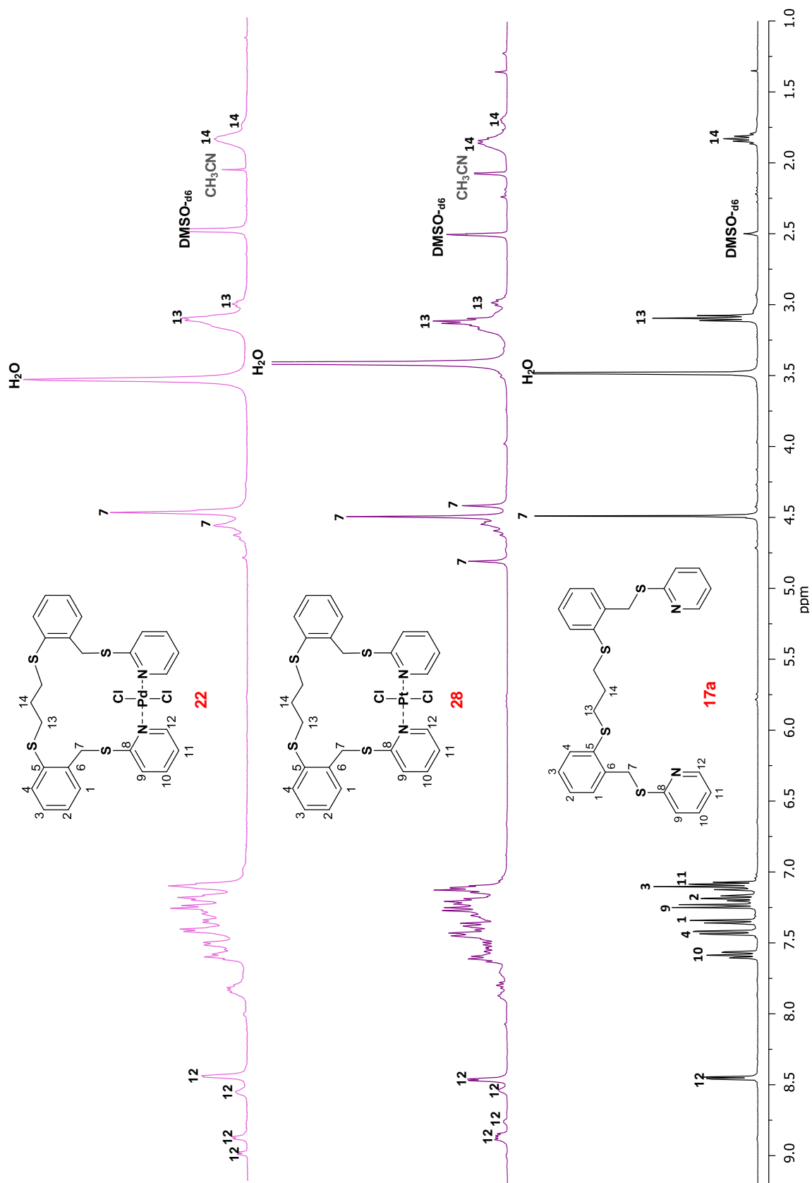
Figura 3.3. Comparación de los espectros de 1 H a 400 MHz de los metalomacrocielos 22 y 28 y el ligante libre 17a , a una conc. 0.05 M a 25 °C,
