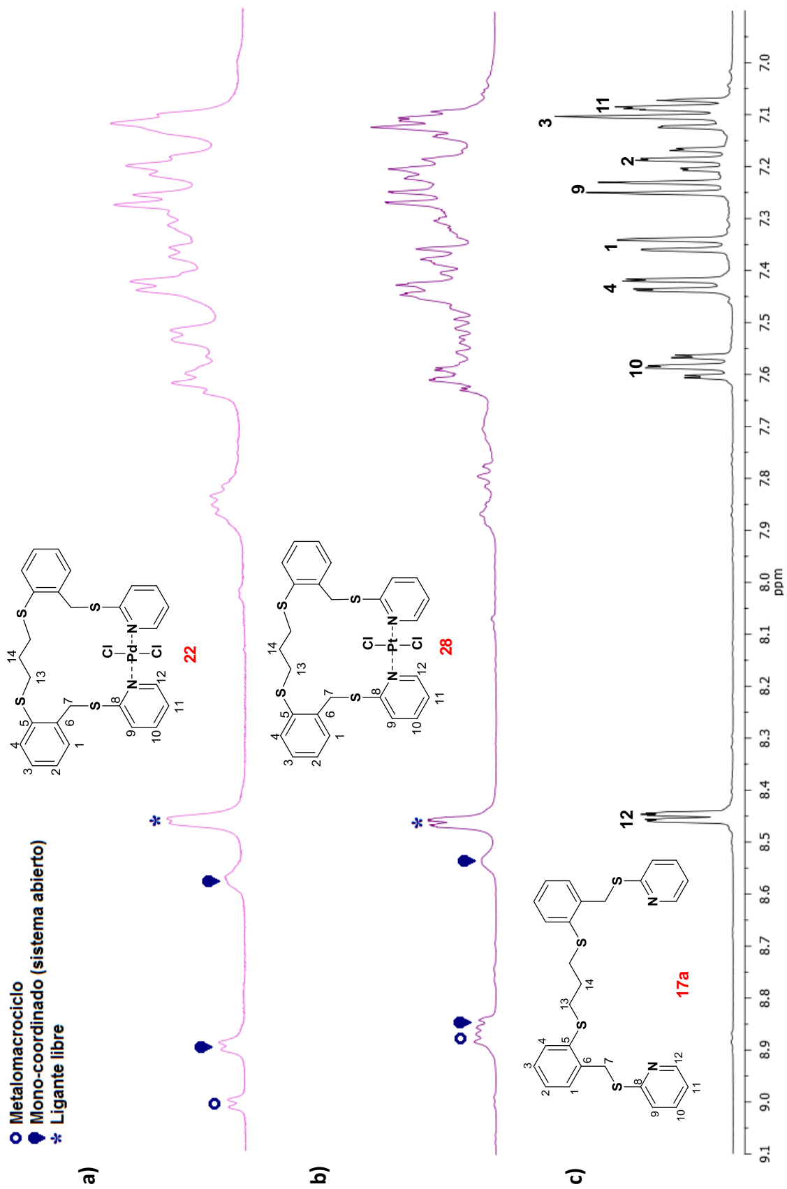
Figura 3.4. Espectro parcial de 1 H (400 MHz, DMSO- d 6 , conc. 0.05 M, 25 °C), espectros; (a) metalomacrocielo 22 , (b) metalomacrocielo 28 , (c) ligante libre 17a .
