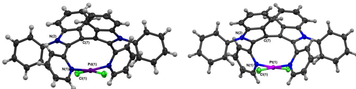
Figura 1.6. Estructura molecular de los complejos de Pd(II) y Pt(II) derivados de la orto -piridina.
