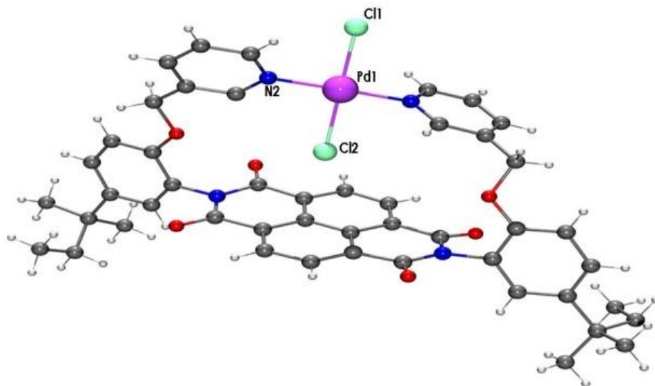
Figura 10. Estructura molecular de un metalomacrocielo de 22 miembros de Pd(II) derivado de la meta -piridina.
