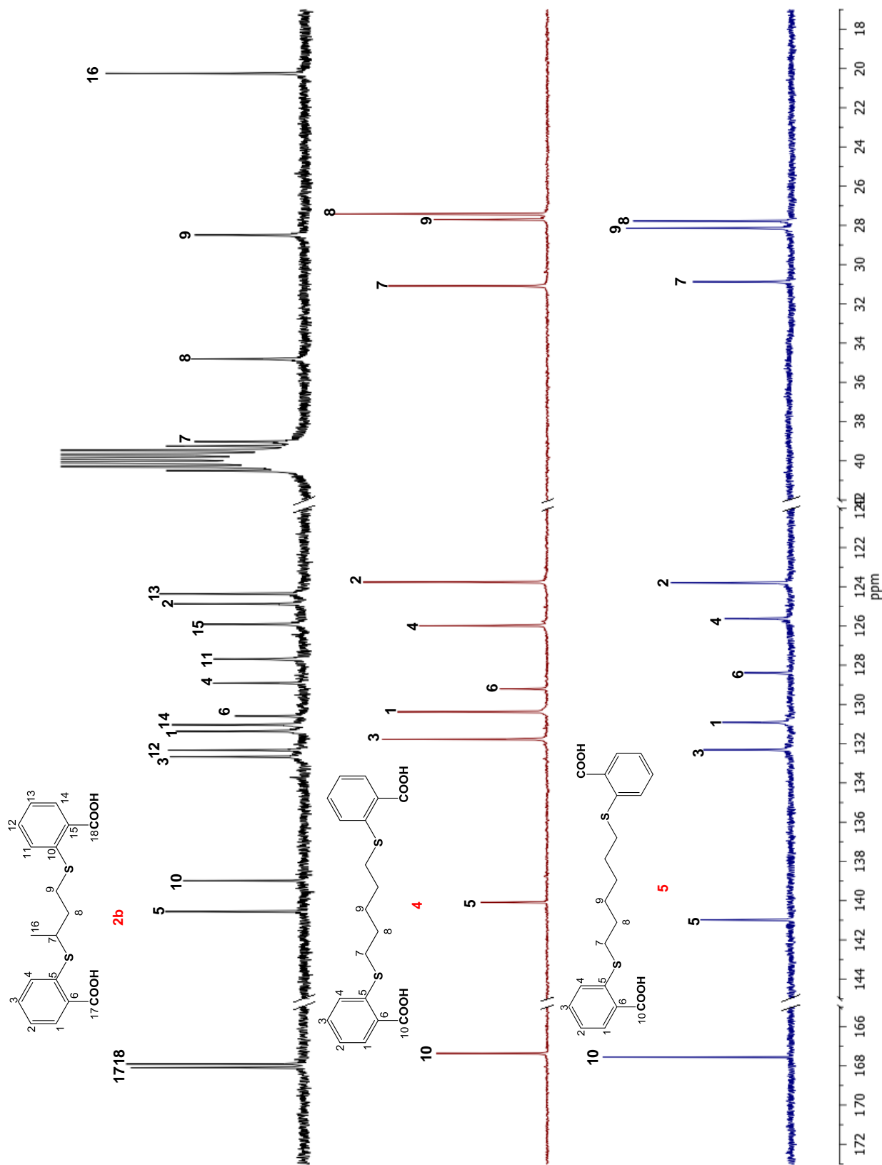
Figura 2.2. Espectros de ^{13}\text{C}\{^1\text{H}\} a 100 MHz de los compuestos 2b, 4 y 5 en DMSO- d_6 .
