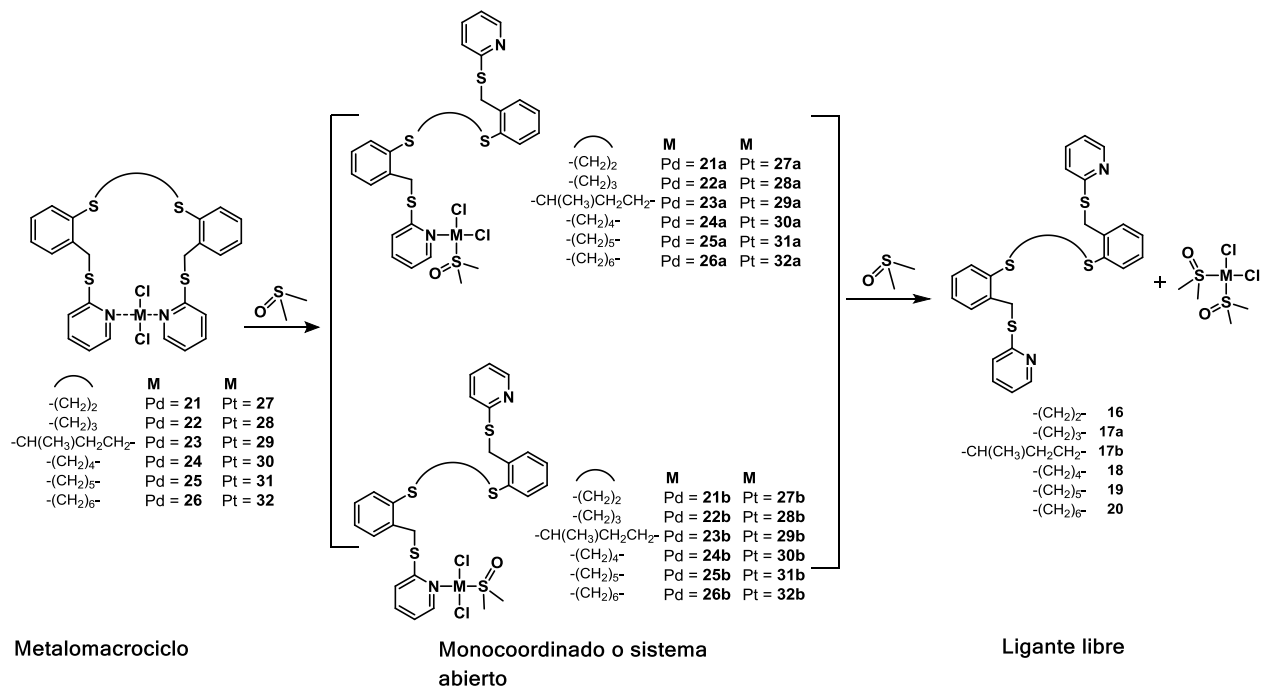
Esquema 3.3. Ruta propuesta para el proceso de desensamble de los metalomacrociclos 21 – 32 .
