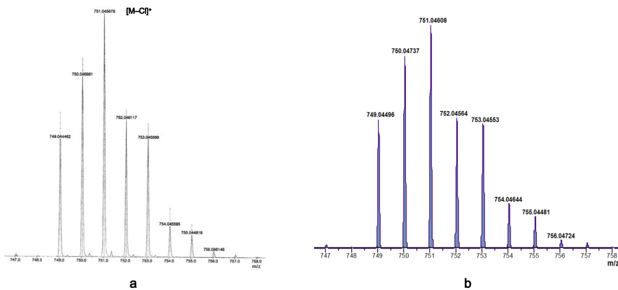
Figura 3.19. Comparación de los picos de masas observado (a) y calculado (b) para el fragmento [M-CI]^+ para el metalomacrocielo 29
