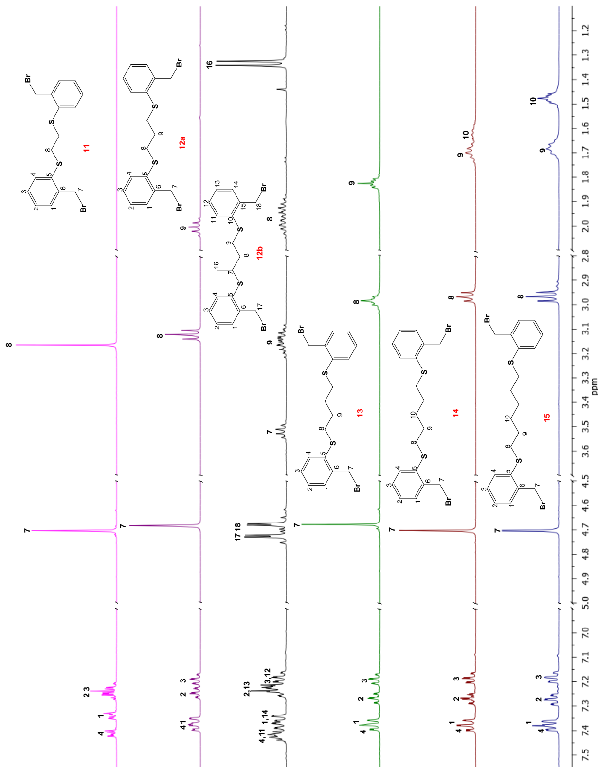
Figura 2.5. Espectros de 1 H a 400 MHz de los compuestos 11 – 15 en CDCl 3 .
