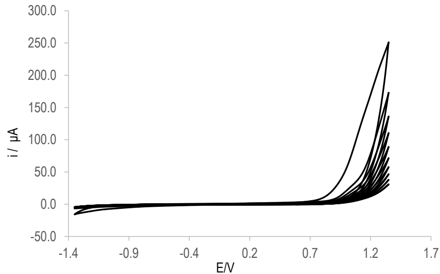
Figura 12. Voltamperogramas cíclicos (se realizaron 10 barridos) obtenidos con el electrodo de barra de grafito para el sistema Ppy-Ibuprofenato. Se realizó en una ventana de potencial de -1.3 a 1.3 V utilizando una velocidad de barrido 0.05 \text{ V s}^{-1} .
