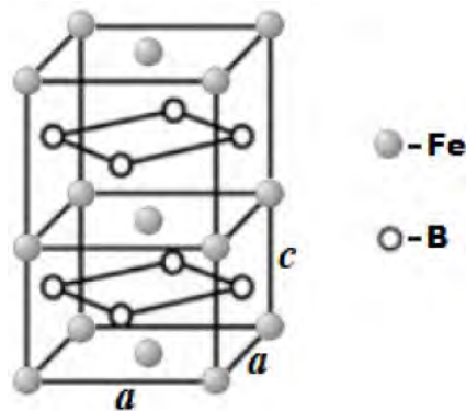
Figura IV.13. Estructura cristalina tetragonal centrada en el cuerpo de la fase \text{Fe}_2\text{B} , donde \alpha = \beta = \gamma = 90^\circ y a = b (\neq c) , con a = 0.5109 \text{ nm} y c = 0.4249 \text{ nm} . Fuente: Ortiz Domínguez, M., 2015.
