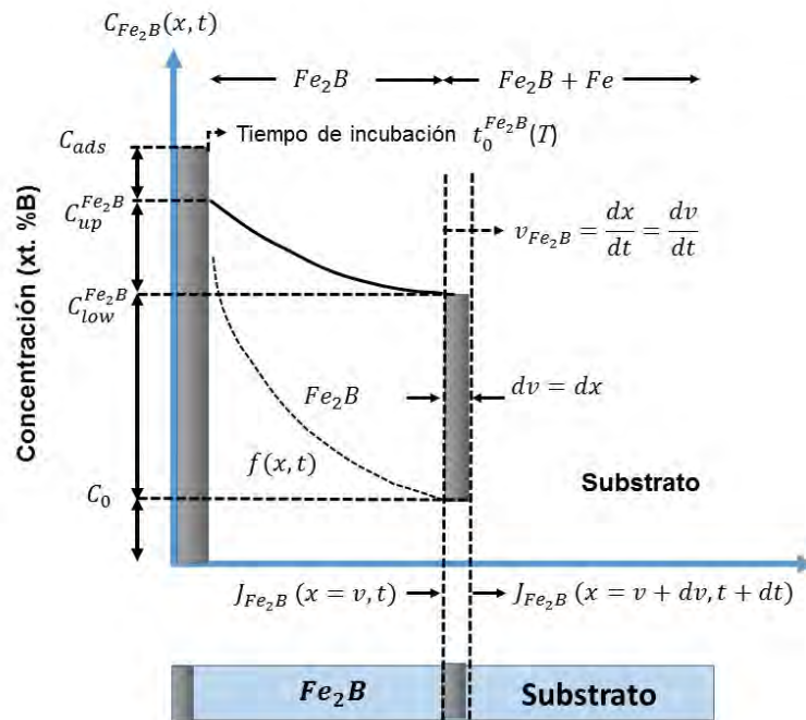
Figura III.1. Perfil de concentración de boro en la capa Fe_2B . Fuente: Autoría propia.
