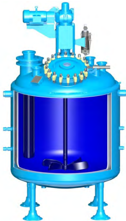
Figura I.4. Reactor criogénico. Fuente: Pfaudler, 2018.
