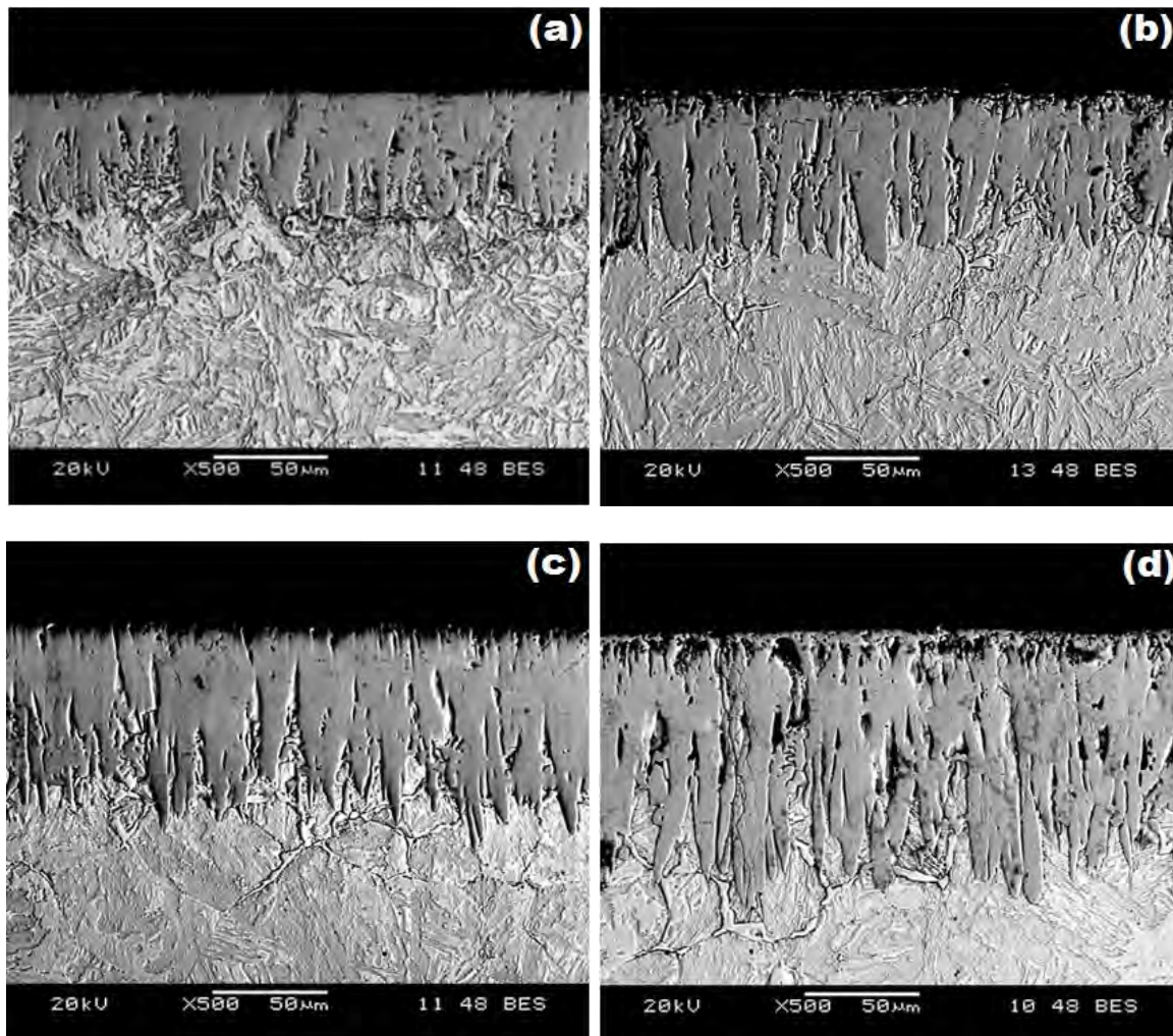
Figura V.17. Microfotografías obtenidas con microscopía electrónica de barrido de las secciones transversales de las muestras boruradas del acero AISI P20, con una temperatura de tratamiento de 1198 K durante diferentes tiempos de exposición: (a) 2 h, (b) 4 h, (c) 6 h y (d) 8 h. Fuente: Autoría propia.
