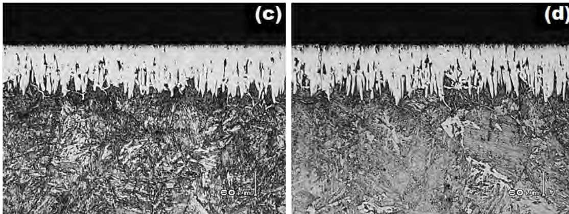
Figura V.13. Microfotografías Ópticas de las secciones transversales de las muestras boruradas del acero AISI P20, con una temperatura de tratamiento de 1223 K durante diferentes tiempos de exposición: (a) 2 h, (b) 4 h, (c) 6 h y (d) 8 h. Fuente: Autoría propia.
