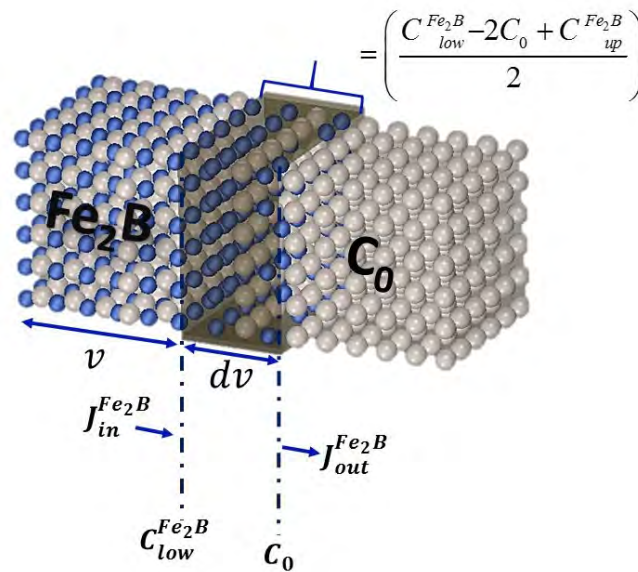
Figura III.4. Balance de masa en la interfase de crecimiento \text{Fe}_2\text{B} /substrato. Fuente: Autoría propia.
