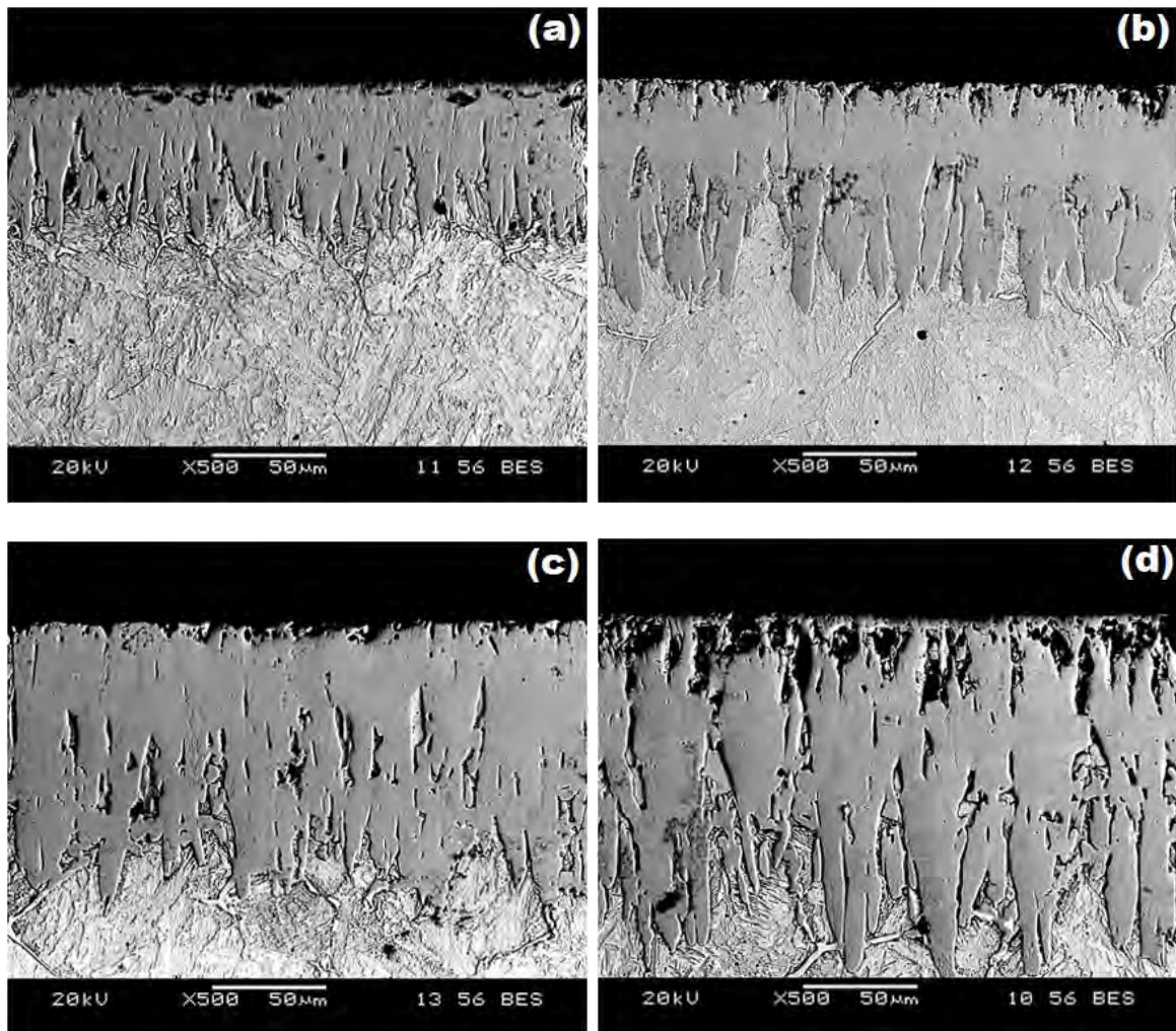
Figura V.18. Microfotografías obtenidas con microscopía electrónica de barrido de las secciones transversales de las muestras boruradas del acero AISI P20, con una temperatura de tratamiento de 1223 K durante diferentes tiempos de exposición: (a) 2 h, (b) 4 h, (c) 6 h y (d) 8 h. Fuente: Autoría propia.
