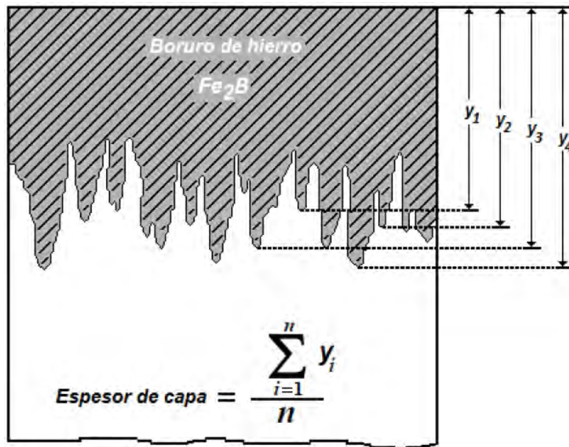
Figura IV.14. Medición de capas boruradas. Fuente: Elías Espinosa, M., Ortiz Domínguez, M., Keddam, M., Flores Rentería, M. A., Damián Mejía O. & Zuno Silva J., 2015.
