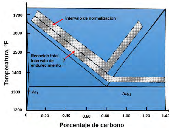
Figura I.1. Intervalo de recocido, normalizado y endurecimiento para aceros al carbono. Fuente: Autoría propia.
