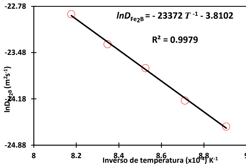
Figura V.22. Relación de Arrhenius para el coeficiente de difusión de boro ( D_{Fe_2B} ) a través de la capa de Fe_2B . Fuente: Autoría propia.
