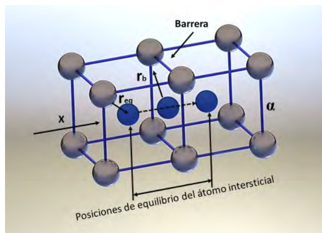
Figura II.7. Consideración de un átomo intersticial en una celda cúbica cristalina. Fuente: Autoría propia.
