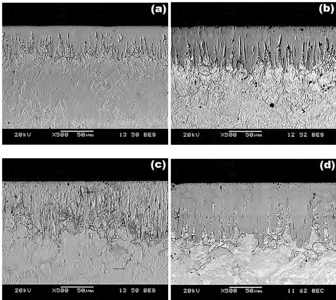
Figura V.16. Microfotografías obtenidas con microscopía electrónica de barrido de las secciones transversales de las muestras boruradas del acero AISI P20, con una temperatura de tratamiento de 1173 K durante diferentes tiempos de exposición: (a) 2 h, (b) 4 h, (c) 6 h y (d) 8 h. Fuente: Autoría propia.
