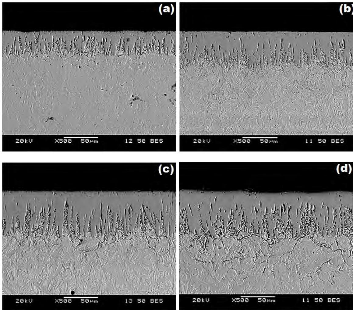
Figura V.15. Microfotografías obtenidas con microscopía electrónica de barrido de las secciones transversales de las muestras boruradas del acero AISI P20, con una temperatura de tratamiento de 1198 K durante diferentes tiempos de exposición: (a) 2 h, (b) 4 h, (c) 6 h y (d) 8 h. Fuente: Autoría propia.
