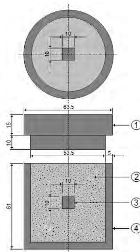
Figura IV.2. Vista esquemática del contenedor de acero AISI 304L empleado para el tratamiento termoquímico de borurización (1: tapa; 2: medio borurante ( B_4C + KBF_4 + SiC ); 3: muestra; 4: contenedor) (escala en milímetros). Fuente: Elias Espinosa, M., Ortiz Domínguez, M., Keddam, M., Flores Rentería, M. A., Damián Mejía O. & Zuno Silva J.,2015.
