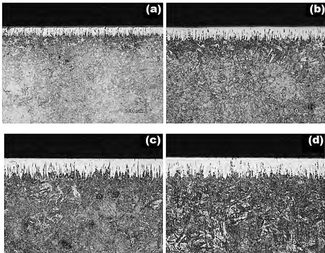
Figura V.11. Microfotografías Ópticas de las secciones transversales de las muestras boruradas del acero AISI P20, con una temperatura de tratamiento de 1173 K durante diferentes tiempos de exposición: (a) 2 h, (b) 4 h, (c) 6 h y (d) 8 h. Fuente: Autoría propia.
