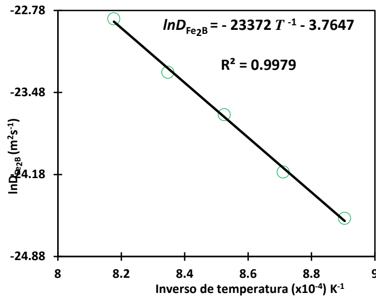
Figura V.21. Relación de Arrhenius para el coeficiente de difusión de boro ( D_{Fe_2B} ) a través de la capa de Fe 2 B. Fuente: Autoría propia.
