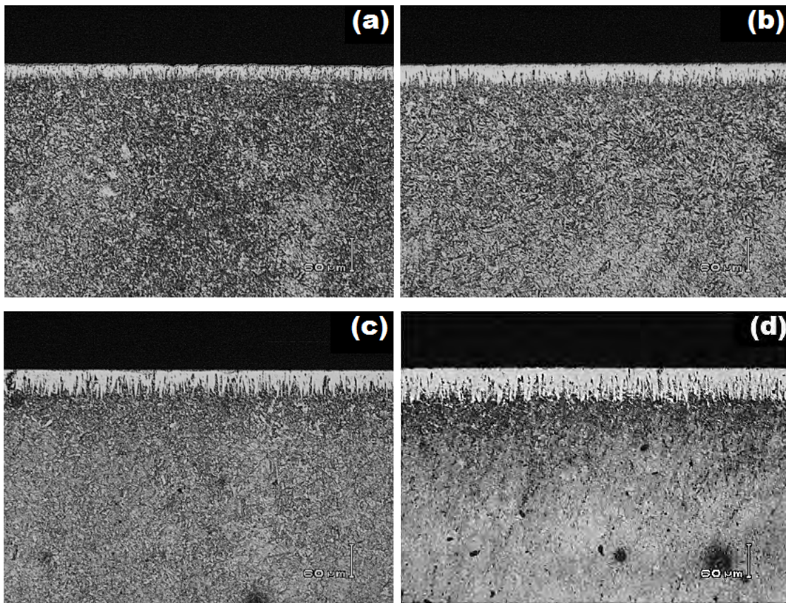
Figura V.9. Microfotografías Ópticas de las secciones transversales de las muestras boruradas del acero AISI P20, con una temperatura de tratamiento de 1123 K durante diferentes tiempos de exposición: (a) 2 h, (b) 4 h, (c) 6 h y (d) 8 h. Fuente: Autoría propia.
