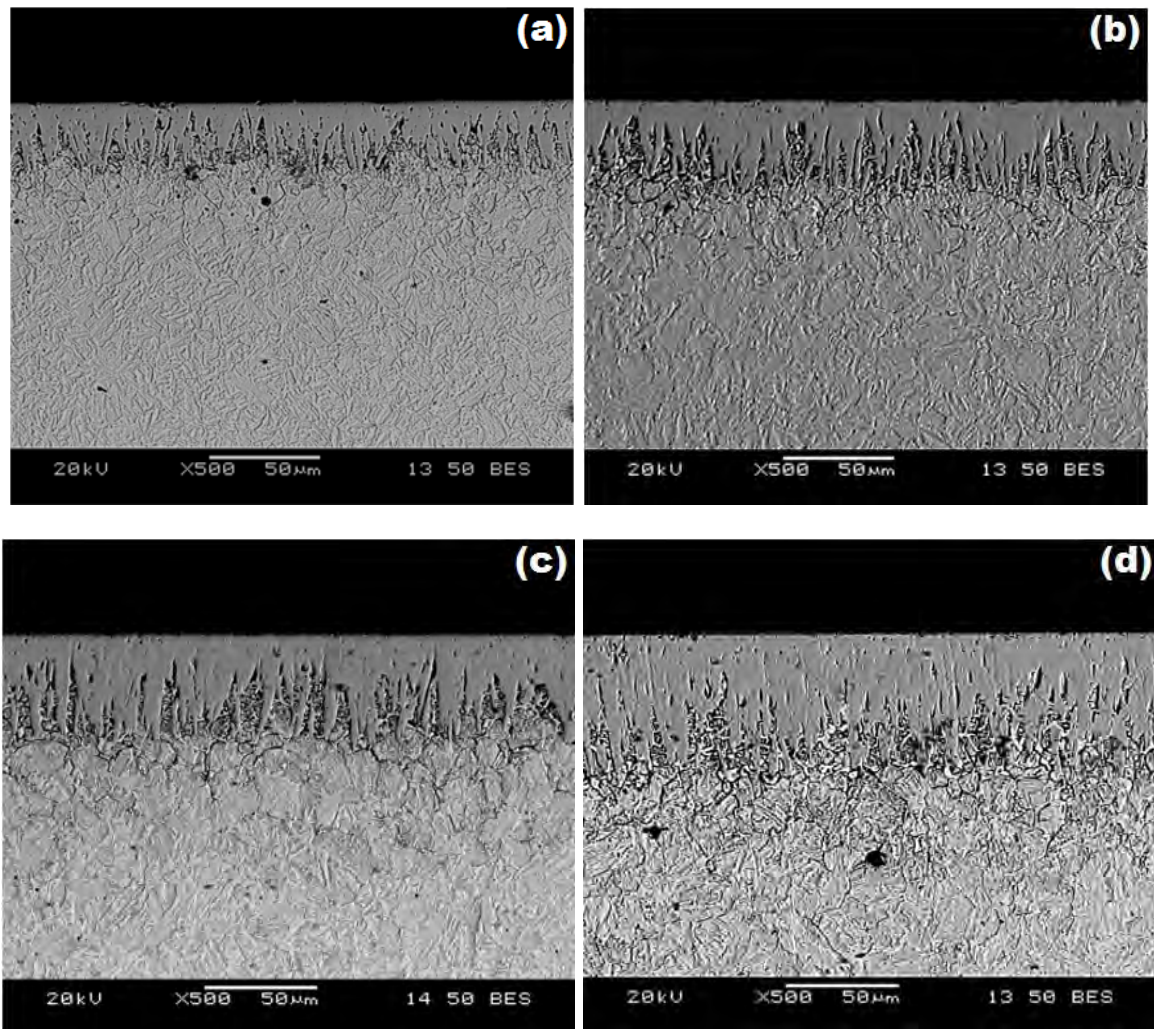
Figura V.14. Microfotografías obtenidas con microscopía electrónica de barrido de las secciones transversales de las muestras boruradas del acero AISI P20, con una temperatura de tratamiento de 1198 K durante diferentes tiempos de exposición: (a) 2 h, (b) 4 h, (c) 6 h y (d) 8 h. Fuente: Autoría propia.
