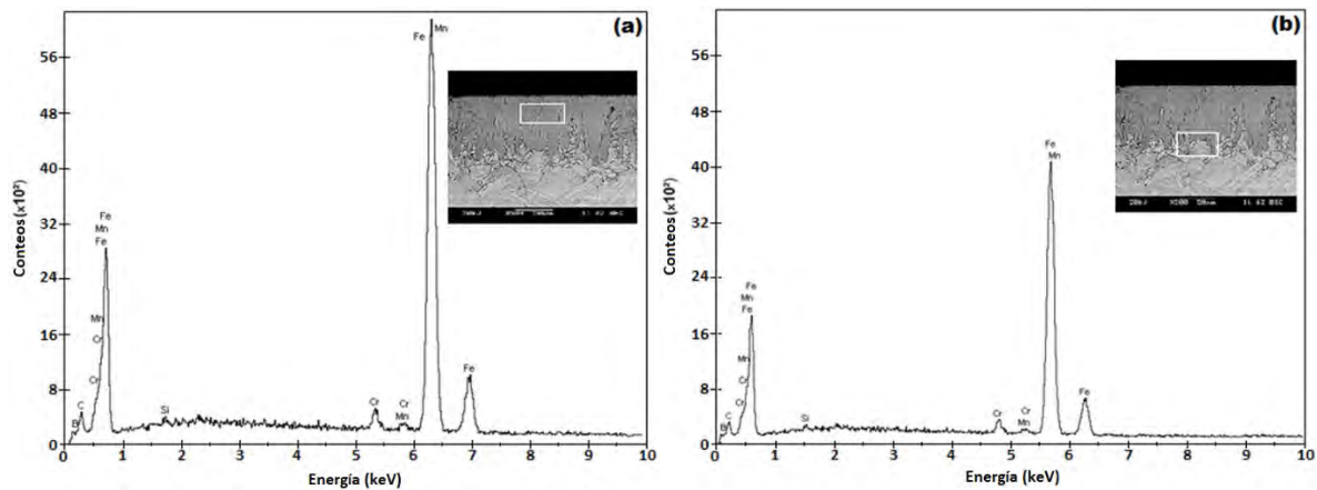
Figura V.19. Una micrografía (SEM) de las secciones transversales de la imagen de la micrografía del acero endurecido AISI P20 obtenida a la temperatura de 1173 K con un tiempo de exposición de 6 h, (a) y (b) espectro EDS de la muestra borurada. Fuente: Autoría propia.
