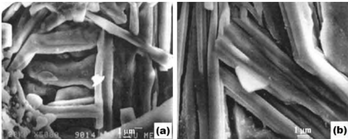
Figura V.6. Micrografías con la técnica de Microscopía Electrónica de Barrido (SEM) de cristales Fe_2B creciendo en la superficie del metal, donde (a) detenido, o (b) forzado a cambiar de dirección como consecuencia de estar en contacto con cristales adyacentes. Fuente: C. Martini, G. Palombarini, & M. Carbucicchio, 2004.
