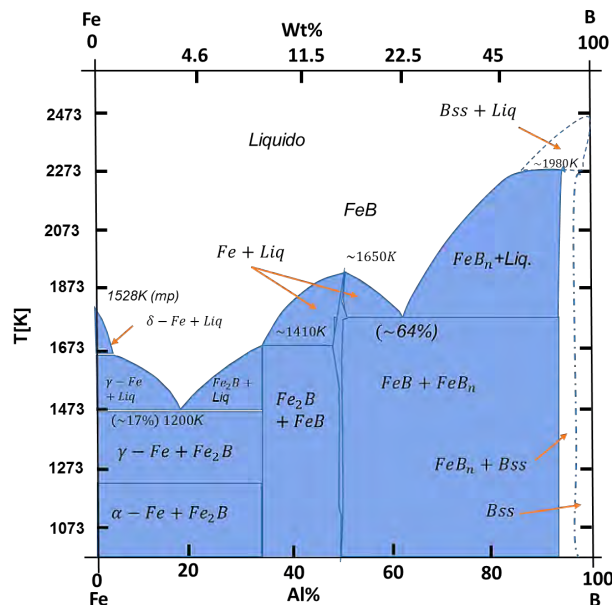
Figura I.5. Diagrama de fases del sistema binario Fe-B. Fuente: Autoría propia.
