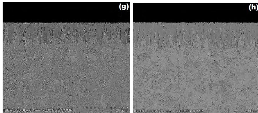
Figura I.8. Efectos de los elementos de aleación en las morfologías de las capas boruradas, sobre diferentes aceros borurados. a) y b) Acero AISI 4150; c) y d) AISI 1025, e) y f) AISI 1026; g) y h) AISI 1518. Fuente: Autoría propia.
