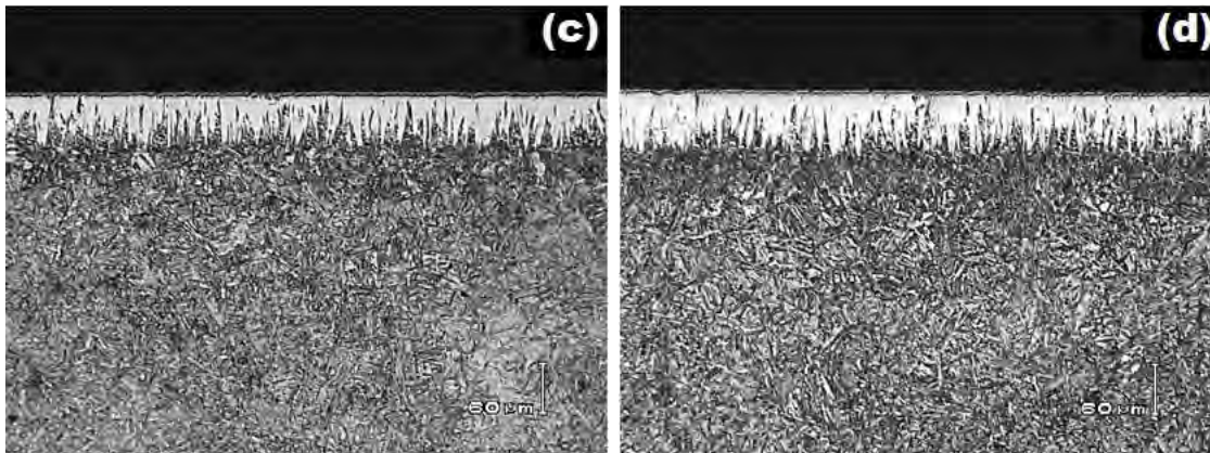
Figura V.10. Microfotografías Ópticas de las secciones transversales de las muestras boruradas del acero AISI P20, con una temperatura de tratamiento de 1148 K durante diferentes tiempos de exposición: (a) 2 h, (b) 4 h, (c) 6 h y (d) 8 h. Fuente: Autoría propia.
