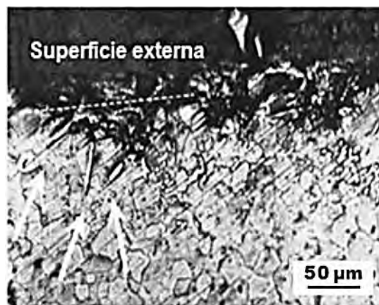
Figura V.4. Metalografía de una sección transversal de una muestra de hierro puro donde se puede apreciar cavidades en la superficie debido al crecimiento de cristales Fe_2B dentro del sustrato. Fuente: C. Martini, G. Palombarini, & M. Carbuicchio, 2004.
