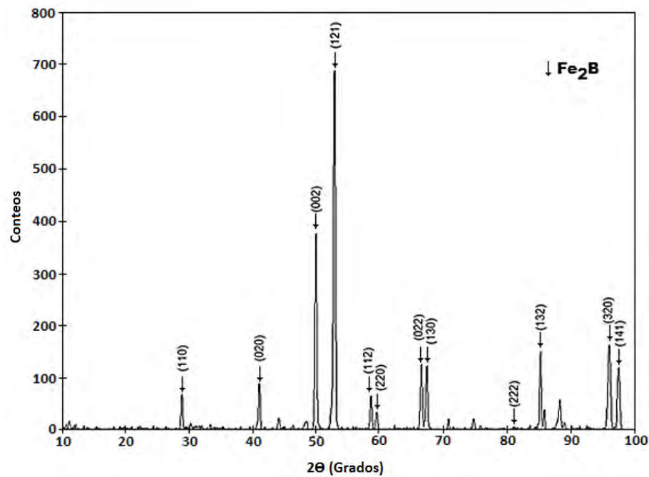
Figura IV.11. Difractograma obtenido en la superficie del acero borurado AISI P20. La temperatura de borurización es de 1223 K con 4 h de tratamiento. Fuente: Autoría propia.
