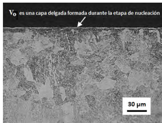
Figura V.8. Microfotografía óptica de la sección transversal de una muestra borurada del acero AISI P20 con un tiempo de tratamiento de durante la temperatura de borurización de 1123 K. Fuente: Autoría propia.
