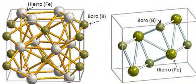
Figura I.6. Representación esquemática de las celdas unitarias de los boruros de hierro a) tipo Fe_2B , b) tipo FeB . Fuente: Autoría propia.
