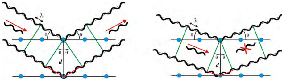
Figura IV.12. De acuerdo al ángulo de desviación ( 2\theta ), el cambio de fase de las ondas produce interferencia constructiva (Figura izquierda) o destructiva (Figura derecha). Fuente: Xtal, 2019.
