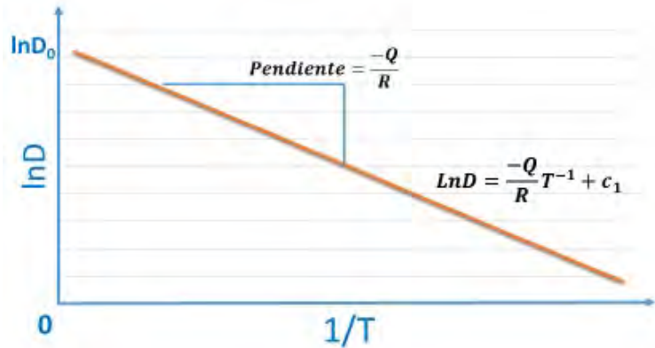
Figura II.8. Gráfica de pendiente de \ln D vs 1/T . Fuente: Autoría propia.
