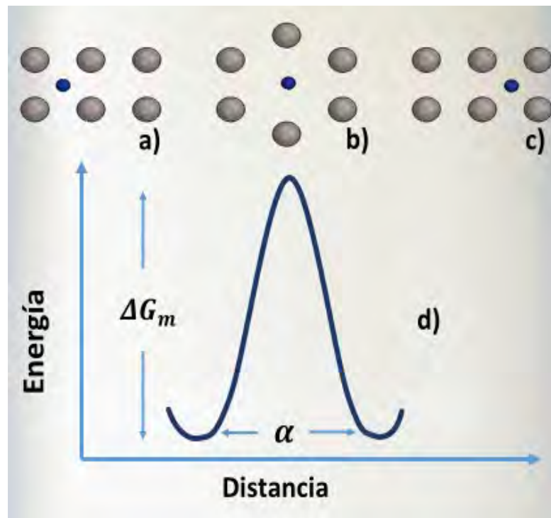
Figura II.5. (d) Representación de la energía libre de red al momento de que un átomo se mueva de (a) a (c). Fuente: Autoría propia.
