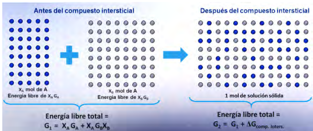
Figura II.2. Energía libre del compuesto intersticial. Fuente: Autoría propia.
