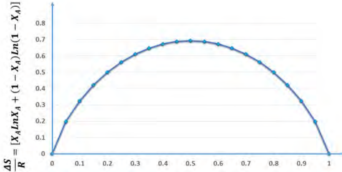
Figura II.4. \Delta S_{\text{comp.inters.}} es la entropía del compuesto intersticial que aumenta al formar un mol de solución. Fuente: Autoría propia.
