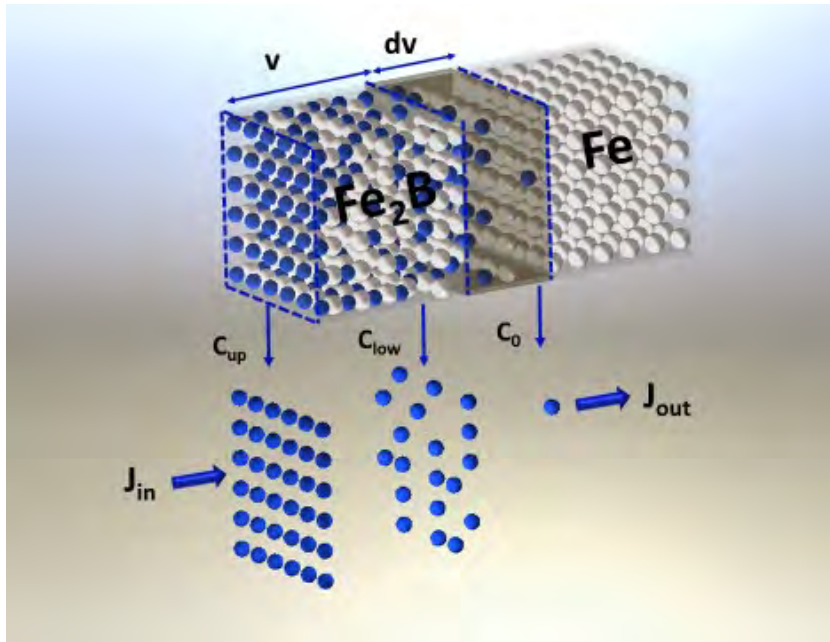
Figura III.3. Flujo de átomos de boro en la interface. Fuente: Autoría propia.
