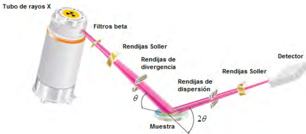
Figura IV.10. Esquematización del funcionamiento de un difractómetro de rayos X. Fuente: Xtal, 2015.
