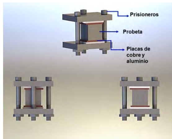
Figura IV.4. Dispositivo empleado para el desbaste de las probetas endurecidas. Fuente: Autoría propia.
