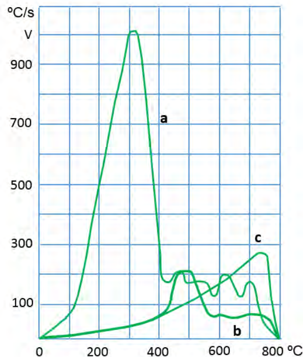
Figura 1.2. Representación esquemática de la velocidad de enfriamiento V en función de la temperatura instantánea, para una esfera de plata de 20 mm de diámetro, templada desde 800°C en: (a) agua a 40°C; (b) aceite mineral a 40°C; (c) baño de sal a 200°C. Fuente: Autoría propia.
