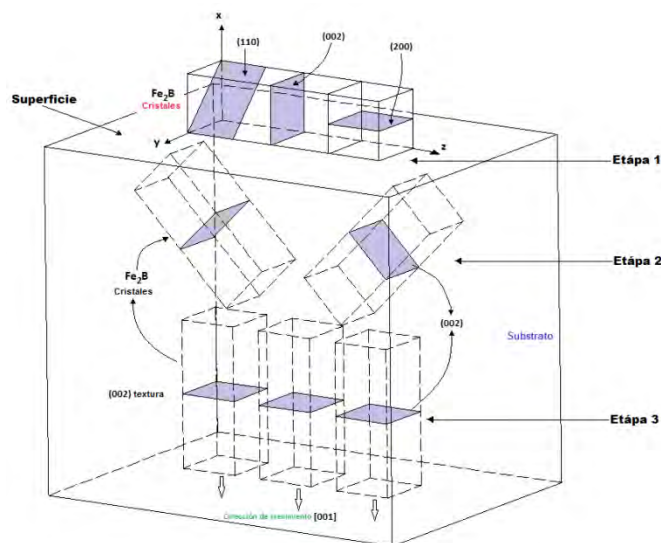
Figura V.5. Representación esquemática de las etapas del crecimiento termoquímico de los cristales \text{Fe}_2\text{B} : etapa 1, crecimiento sobre la superficie del material; etapa 2, crecimiento en el interior del material; etapa 3, el crecimiento profundo conduce a una fuerte orientación preferencial (002). Fuente: Autoría propia.
