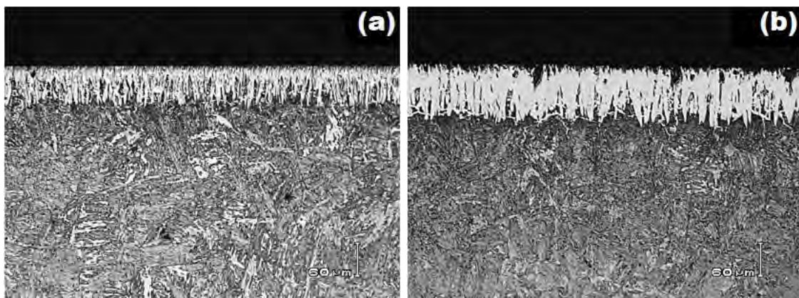
Figura V.12. Microfotografías Ópticas de las secciones transversales de las muestras boruradas del acero AISI P20, con una temperatura de tratamiento de 1198 K durante diferentes tiempos de exposición: (a) 2 h, (b) 4 h, (c) 6 h y (d) 8 h. Fuente: Autoría propia.
