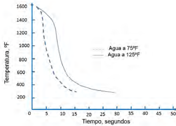
Figura I.3. Curvas de enfriamiento obtenidas en el centro de muestras templadas en agua a temperaturas de 75°F (24°C) y 125°F (52°C) sin agitación.
