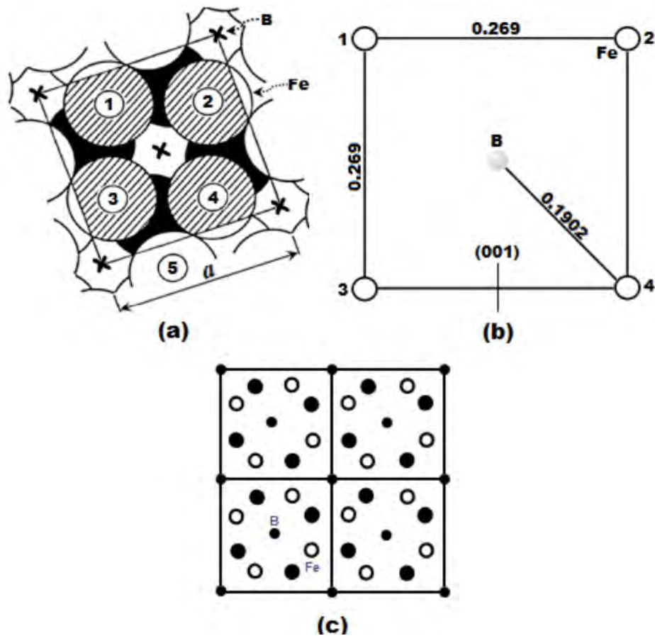
Figura V.3. Proyección de los átomos de hierro Fe sobre el plano perpendicular (001) en el cual un salto atómico de B lleva a cabo en la fase Fe_2B . Los puntos centrales de los átomos eclosionados están en un plano a una distancia de 3c/4 por encima del plano de proyección; los puntos centrales de los átomos oscuros están en un plano a una distancia de c/4 por encima del plano de proyección. Los radios atómicos de Fe han sido tomados igual a la mitad de la distancia más corta en la estructura Fe-Fe: 0.120 nm (por ejemplo, el par de átomos 4-5 en (a)). Los átomos de B no han sido dibujados, pero las proyecciones de los átomos de B coinciden con las cruces que se indican en (a). En (b) se representa la configuración del átomo de Fe alrededor del átomo de B para la fase Fe_2B en el momento de máximo acercamiento durante un salto atómico de B perpendicular a (001); y finalmente en (c) representa la misma estructura de la fase Fe_2B proyectada sobre el plano (001) con la colocación de los átomos en la estructura cristalina tetragonal = átomo de Fe en 1/4 c ; \bullet = átomo de Fe en 3/4 c ; \circ = 3 átomos de B en 0, 1/2, 1c . Fuente: Brakman, C. M., Gommers, A. W. J. & Mittemeijer, E. J., 1989.
