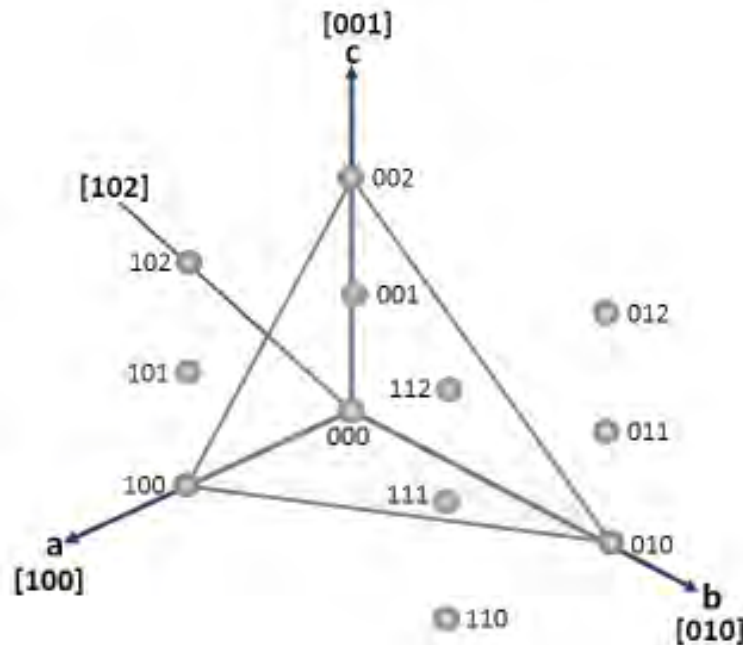
Figura V.2. Direcciones y planos cristalográficos. Fuente: Autoría propia.
