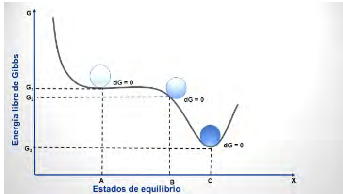
Figura II.1. Variación de la energía libre de Gibbs, el estado de equilibrio “A” está en equilibrio débilmente estable. La configuración “B” se encuentra en equilibrio inestable y la configuración “C” está en equilibrio fuertemente estable. Fuente: Autoría propia.
