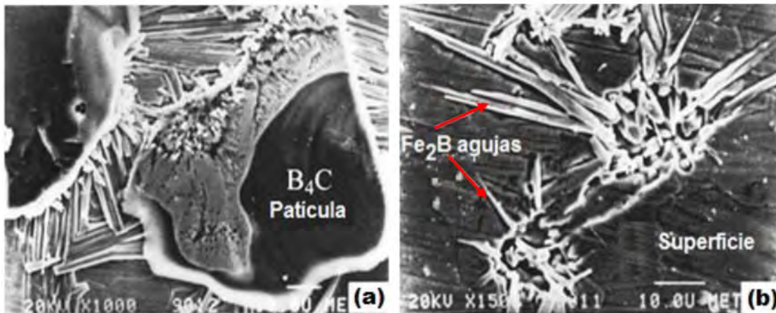
Figura V.1. Muestra de hierro con un tiempo de tratamiento de 1h a la temperatura de 1123 K en contacto con potencial químico de boro bajo (ver Tabla V.1): (a) imagen tomada con un microscopio electrónico de barrido de cristales de B_4C (áreas oscuras) en la superficie del sustrato y cristales acirculares de Fe_2B creciendo sobre la superficie del metal en las zonas de contacto B_4C -metal; (b) detalles del crecimiento de los cristales Fe_2B en (a), después de la remoción de las partículas de carburo de boro. Fuente: C. Martini, G. Palombarini, & M. Carbucchio, 2004.
