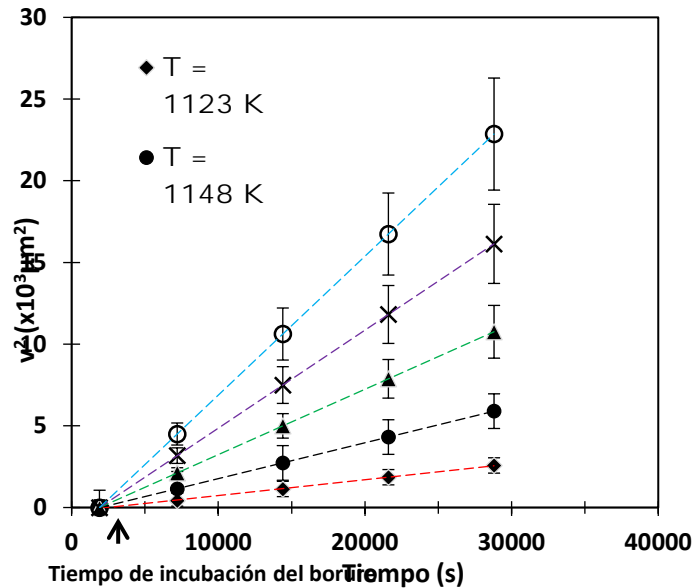
Figura V.20. Espesor al cuadrado de la capa borurada Fe 2 B (v 2 ) vs. (t) tiempo de borurización para diferentes temperaturas. Fuente: Autoría propia.
