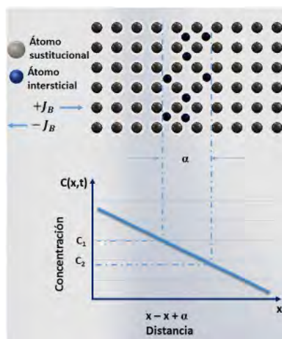
Figura II.6. Representación esquemática de la difusión unidireccional de átomos en una red cristalina. Fuente: Autoría propia.
