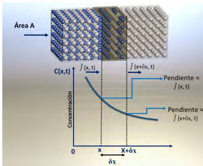
Figura II.9. Esquematización de la segunda ley de Fick. Fuente: Autoría propia.
