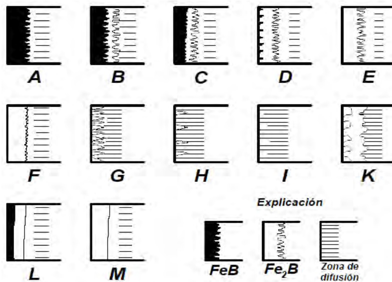
Figura I.7. Tipos de capas boruradas, que se pueden obtener dependiendo del sustrato empleado, potencial de boro, tiempo y temperatura de tratamiento. Fuente: Matuschka, A. & Graf, V., 1980.
