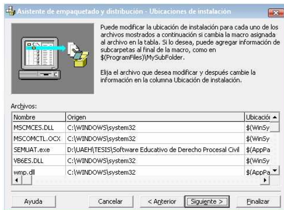
Figura 4.34 Ubicación de instalación de los archivos..
