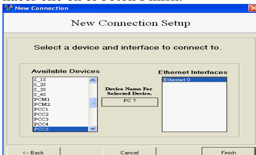
Figura 6.238 Interfaz ethernet 0 de la computadora PCC5
