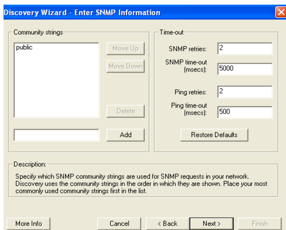
Figura 5.17 Pantalla del Enter SNMP information
