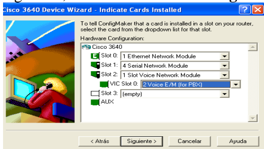
Figura 6.130 Tarjetas del enrutador cisco serie 3640 CD.SAHAGÚN
