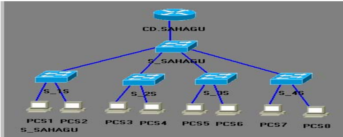
Figura 6.301 Diagrama de las conexiones de la planta manufacturera de la CD.SAHAGUÍN
