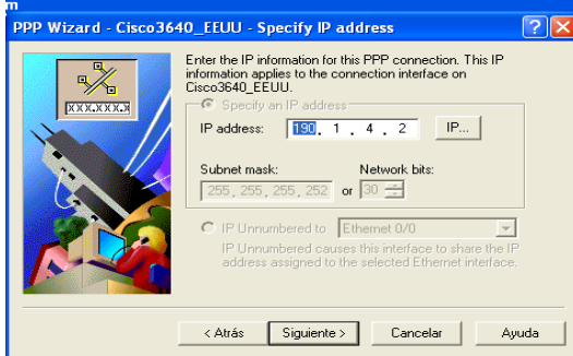
Figura 6.194 Dirección IP del enrutador cisco serie 3640 EEUU para la interfaz serial 1/1
