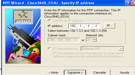
Figura 6.186 Dirección IP del enrutador cisco serie 3640 EEUU para la interfaz serial 1/0
