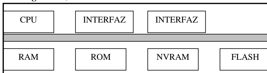
Figura 4.1 Estructura de un enrutador
