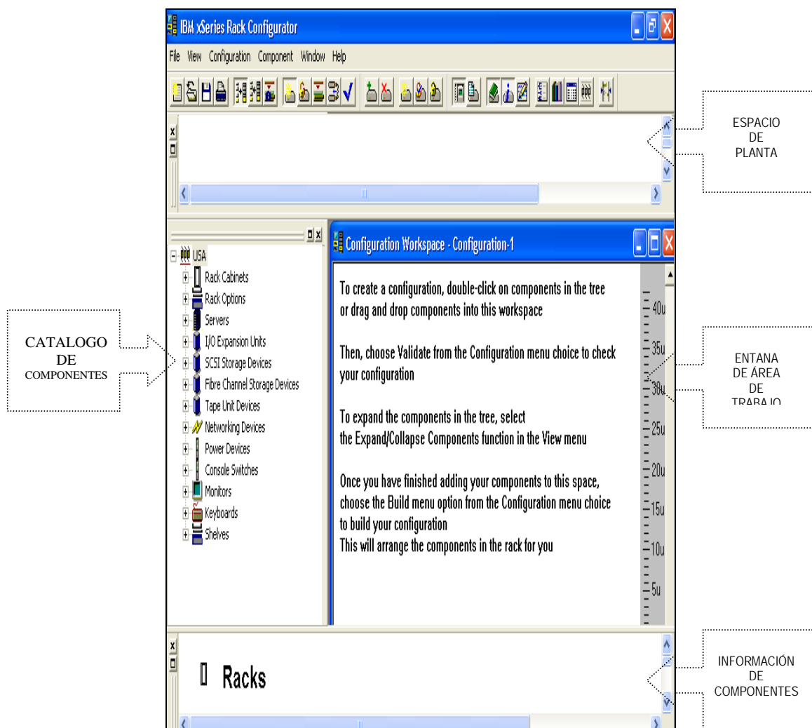
Figura 2.6 Pantalla principal del software IBM xSerie Rack Configurator versión 2.19
