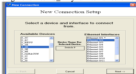
Figura 6.260 Interfaz ethernet 0/2 del switch S_2E
