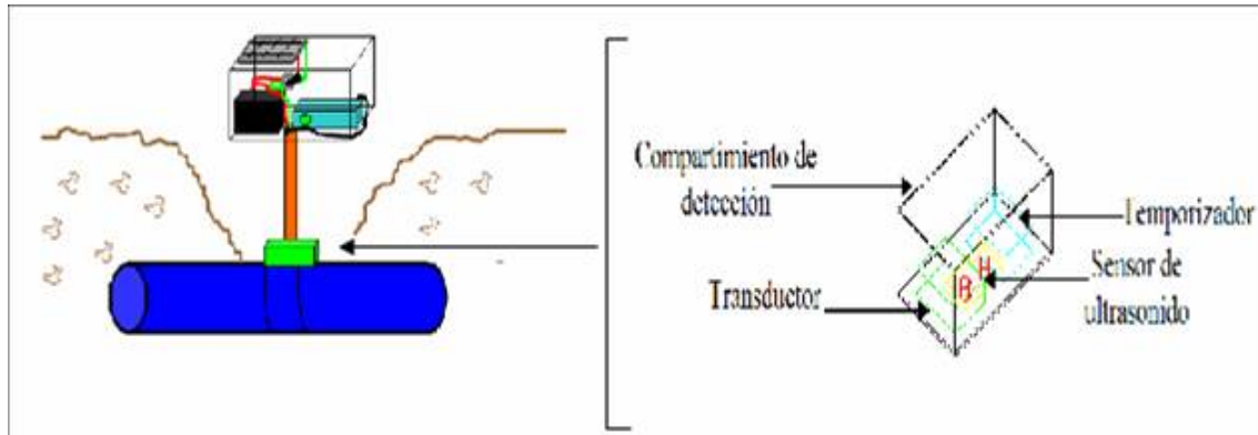
Figura 5.23 Diagrama del dispositivo listo para su funcionamiento
