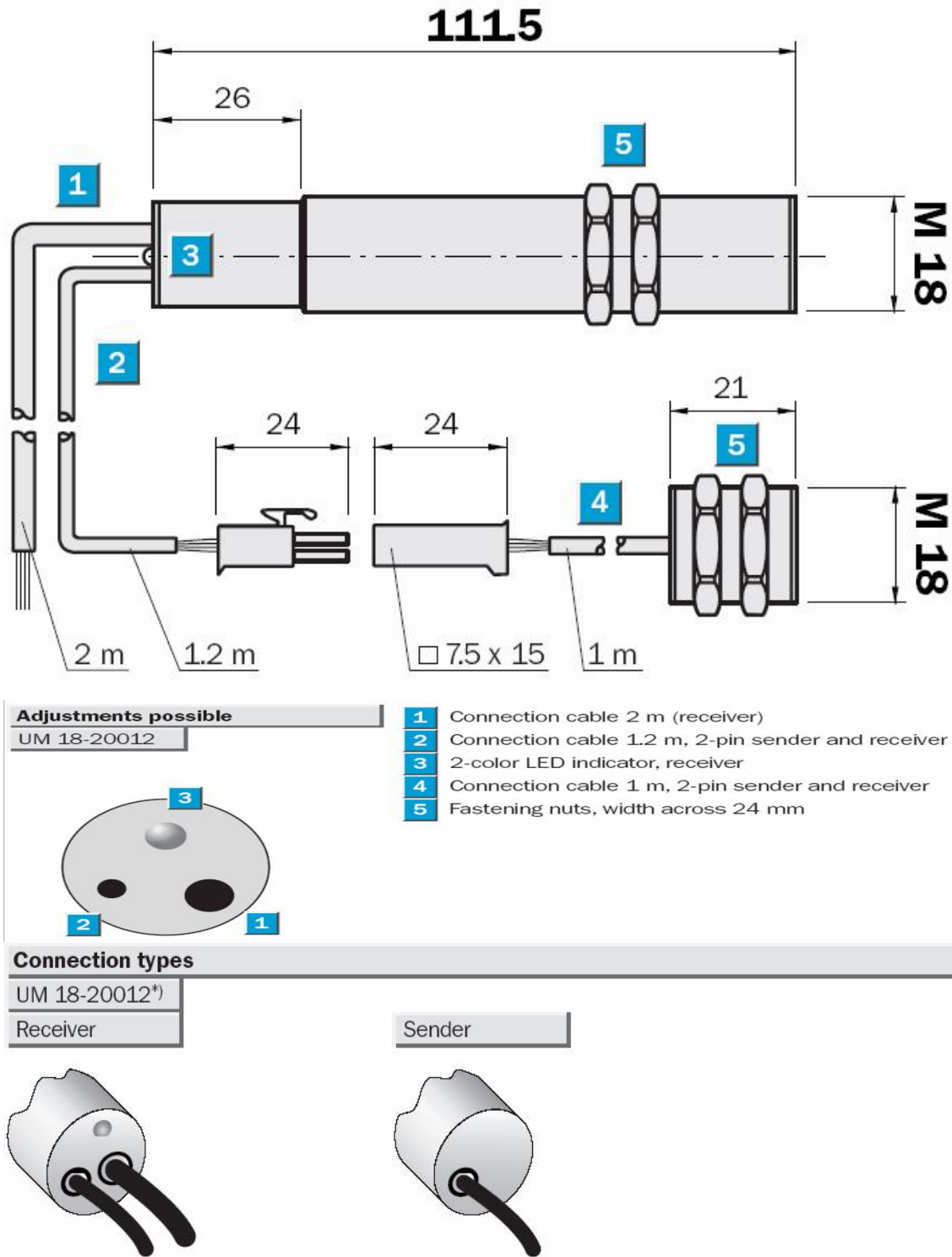
Figura. 5.11. Características del Sensor de ultrasonido UM-1820012. Fuente: www.gemssensors.com
