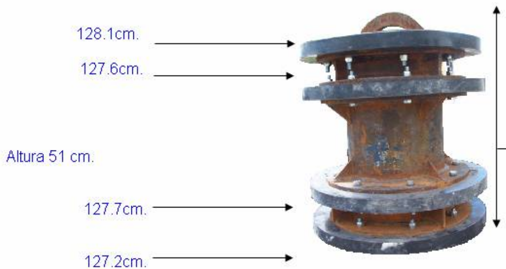
Figura 5.24 Foto del DIM utilizado para esta corrida
