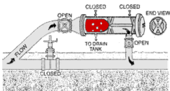
Figura 3.16 Recibo convencional de un DIM. Fuente: http://www.girard.com/valves-launching.html , Foto tomada durante el recibo de un DIM en instalaciones de PEMEX
