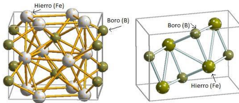
Figura 1.6. Representación esquemática de las celdas unitarias de los boruros de hierro a) tipo \text{Fe}_2\text{B} , b) tipo \text{FeB} . Fuente: Autoría propia.
