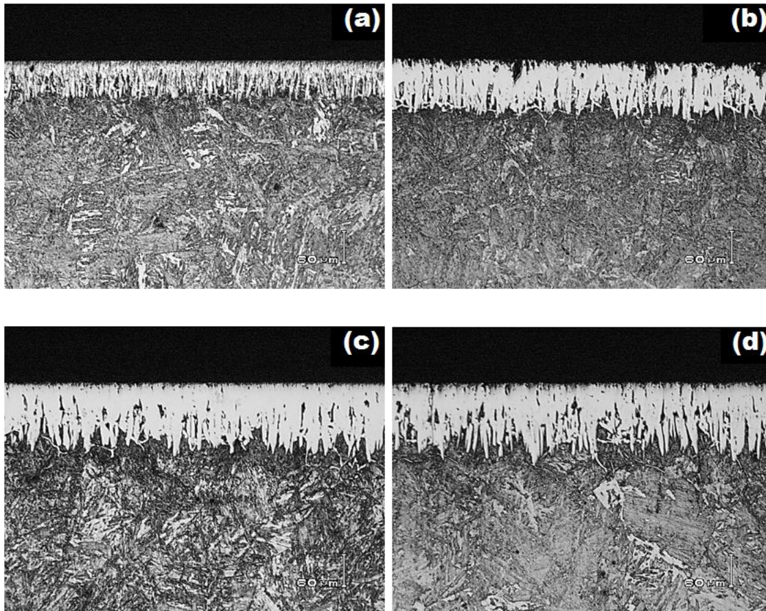
Figura V.13. Microfotografías Ópticas de las secciones transversales de las muestras boruradas del acero AISI P20, con una temperatura de tratamiento de 1223 K durante diferentes tiempos de exposición: (a) 2 h, (b) 4 h, (c) 6 h y (d) 8 h. Fuente: Autoría propia.
