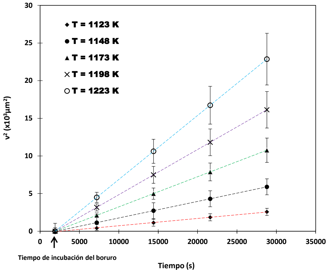
Figura V.20. Espesor al cuadrado de la capa borurada \text{Fe}_2\text{B} ( v^2 ) vs. ( t ) tiempo de borurización para diferentes temperaturas. Fuente: Autoría propia.
