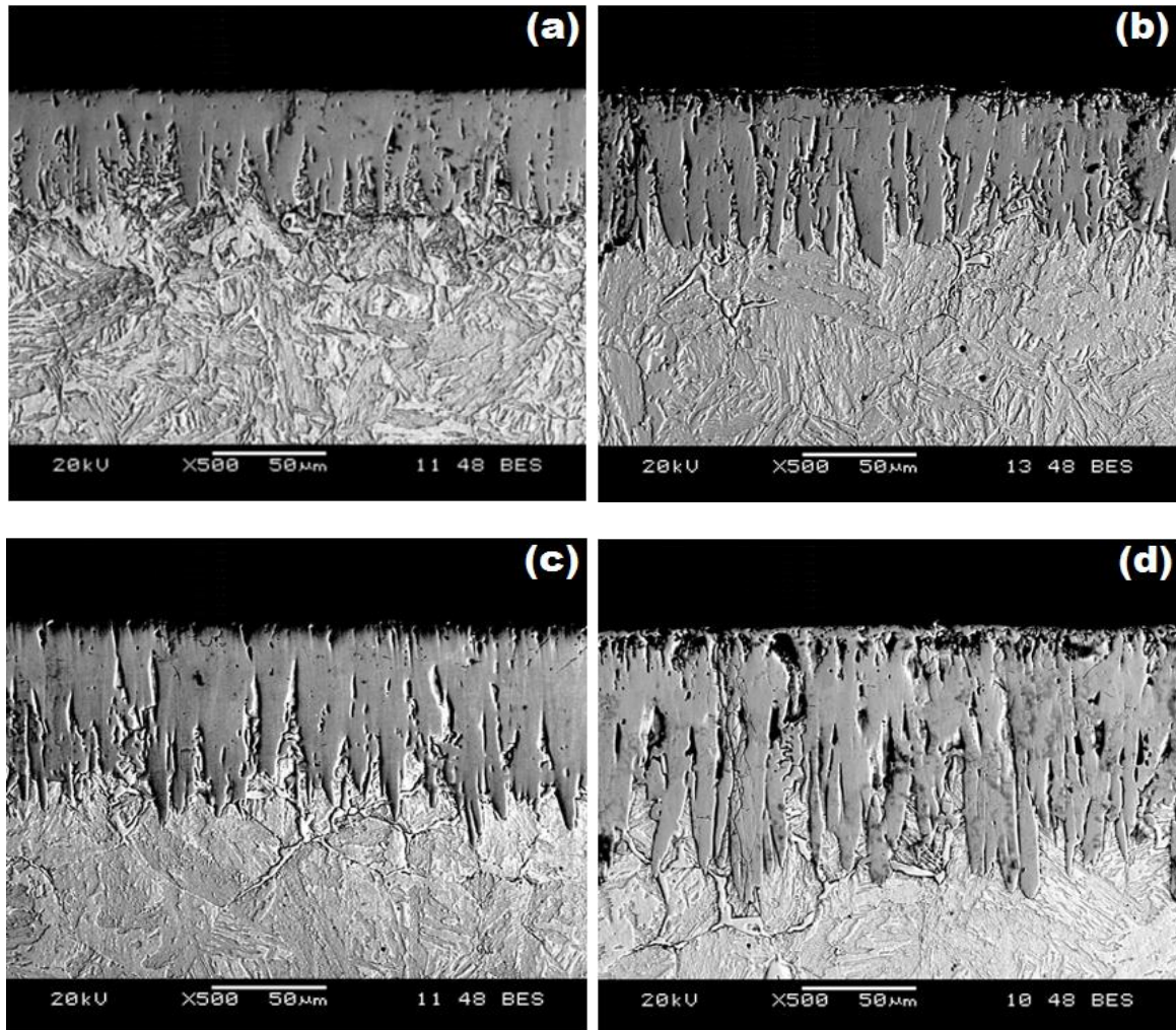
Figura V.17. Microfotografías obtenidas con microscopía electrónica de barrido de las secciones transversales de las muestras boruradas del acero AISI P20, con una temperatura de tratamiento de 1198 K durante diferentes tiempos de exposición: (a) 2 h, (b) 4 h, (c) 6 h y (d) 8 h. Fuente: Autoría propia.
