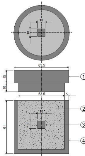
Figura IV.2. Vista esquemática del contenedor de acero AISI 304L empleado para el tratamiento termoquímico de borurización (1: tapa; 2: medio borurante ( \text{B}_4\text{C} + \text{KBF}_4 + \text{SiC} ); 3: muestra; 4: contenedor) (escala en milímetros). Fuente: Elias Espinosa, M., Ortiz Domínguez, M., Keddám, M., Flores Rentería, M. A., Damián Mejía O. & Zuno Silva J., 2015.
