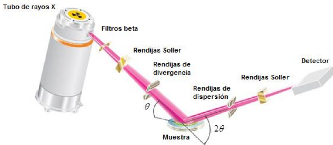
Figura IV.10. Esquematación del funcionamiento de un difractómetro de rayos X. Fuente: Xtal, 2015.
