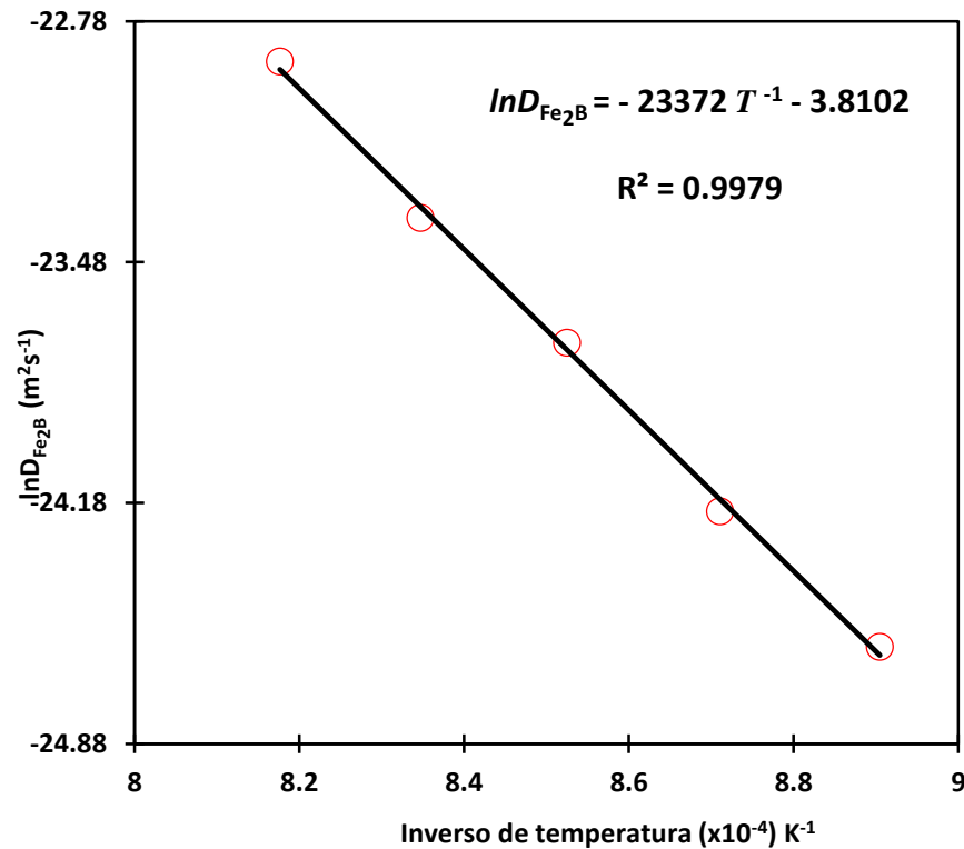
Figura V.22. Relación de Arrhenius para el coeficiente de difusión de boro ( D_{Fe_2B} ) a través de la capa de Fe_2B . Fuente: Autoría propia.
