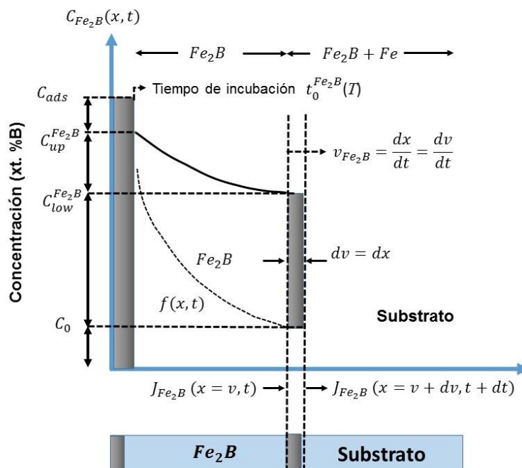
Figura III.1. Perfil de concentración de boro en la capa \text{Fe}_2\text{B} . Fuente: Autoría propia.
