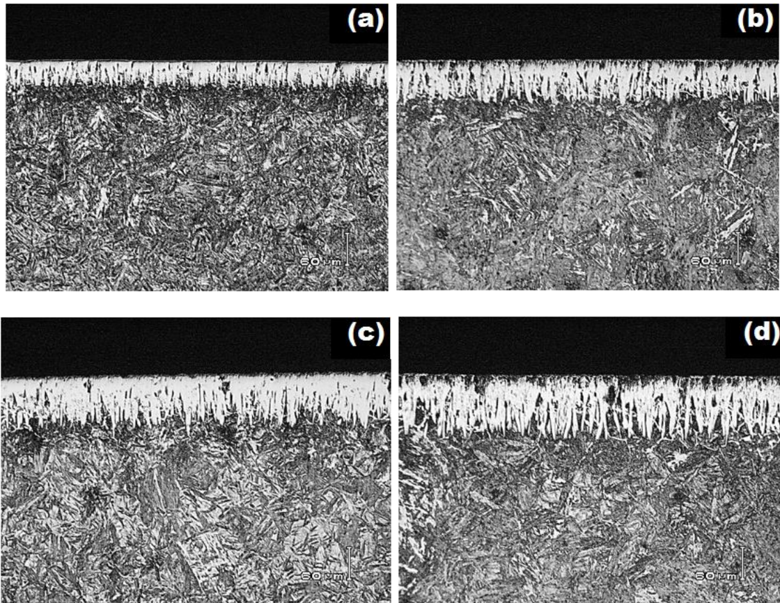
Figura V.12. Microfotografías Ópticas de las secciones transversales de las muestras boruradas del acero AISI P20, con una temperatura de tratamiento de 1198 K durante diferentes tiempos de exposición: (a) 2 h, (b) 4 h, (c) 6 h y (d) 8 h. Fuente: Autoría propia.
