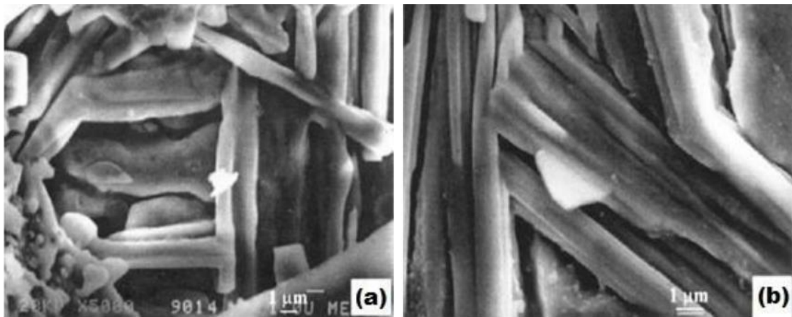
Figura V.6. Micrográficas con la técnica de Microscopía Electrónica de Barrido (SEM) de cristales \text{Fe}_2\text{B} creciendo en la superficie del metal, donde (a) detenido, o (b) forzado a cambiar de dirección como consecuencia de estar en contacto con cristales adyacentes. Fuente: C. Martini, G. Palombarini, & M. Carbucicchio, 2004.
