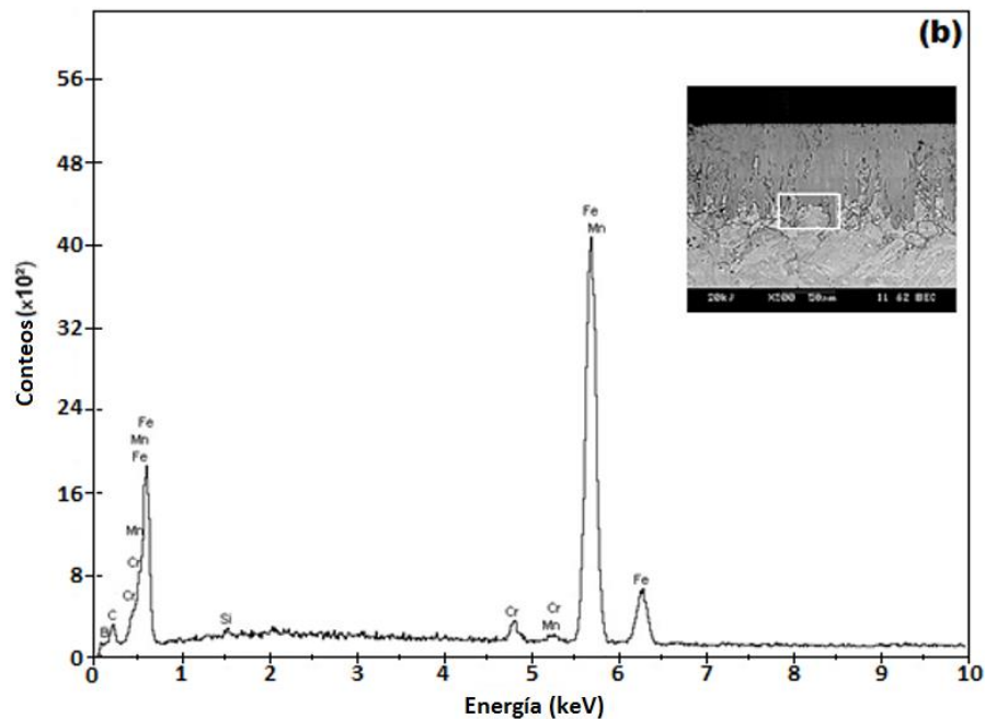
Figura V.19. Una micrografía (SEM) de las secciones transversales de la imagen de la micrografía del acero endurecido AISI P20 obtenida a la temperatura de 1173 K con un tiempo de exposición de 6 h, (a) y (b) espectro EDS de la muestra borurada. Fuente: Autoría propia.
