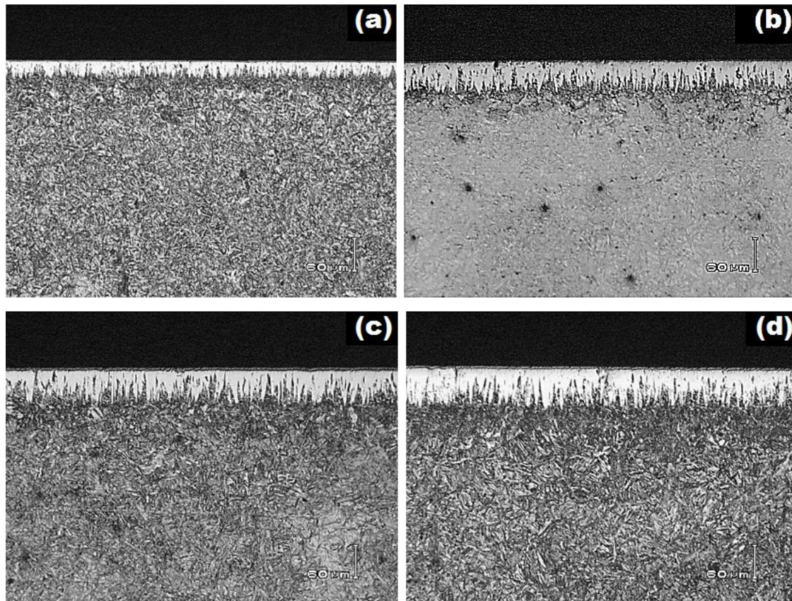
Figura V.10. Microfotografías Ópticas de las secciones transversales de las muestras boruradas del acero AISI P20, con una temperatura de tratamiento de 1148 K durante diferentes tiempos de exposición: (a) 2 h, (b) 4 h, (c) 6 h y (d) 8 h. Fuente: Autoría propia.
