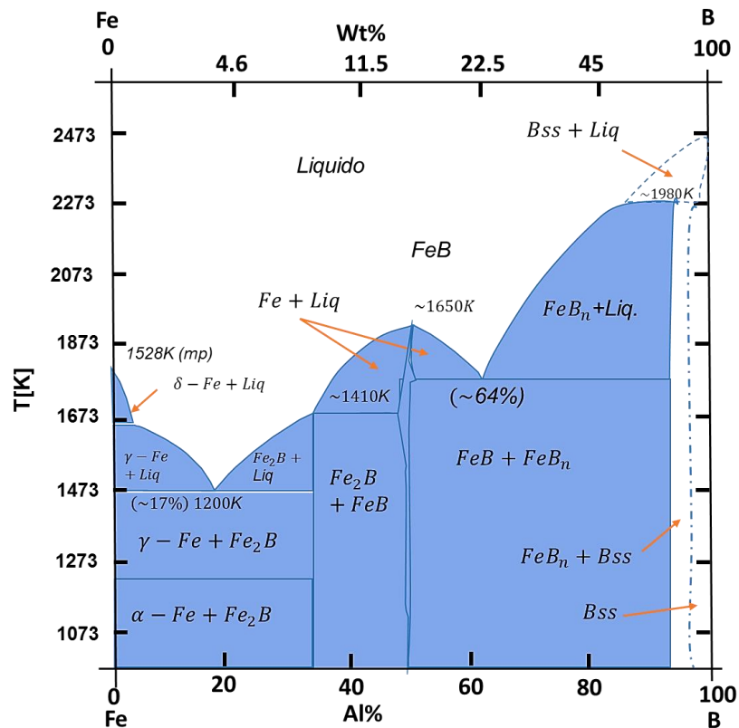
Figura III.2. Diagrama de fases hierro-boro. Fuente: Autoría propia.
