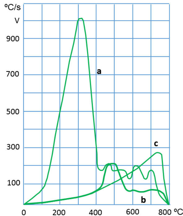
Figura I.2. Representación esquemática de la velocidad de enfriamiento V en función de la temperatura instantánea, para una esfera de plata de 20 mm de diámetro, templada desde 800°C en: (a) agua a 40°C; (b) aceite mineral a 40°C; (c) baño de sal a 200°C. Fuente: Autoría propia.
