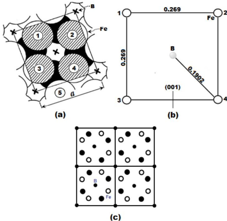
Figura V.3. Proyección de los átomos de hierro Fe sobre el plano perpendicular (001) en el cual un salto atómico de B lleva a cabo en la fase \text{Fe}_2\text{B} . Los puntos centrales de los átomos eclosionados están en un plano a una distancia de 3c/4 por encima del plano de proyección; los puntos centrales de los átomos oscuros están en un plano a una distancia de c/4 por encima del plano de proyección. Los radios atómicos de Fe han sido tomados igual a la mitad de la distancia más corta en la estructura Fe-Fe: 0.120 nm (por ejemplo, el par de átomos 4-5 en (a)). Los átomos de B no han sido dibujados, pero las proyecciones de los átomos de B coinciden con las cruces que se indican en (a). En (b) se representa la configuración del átomo de Fe alrededor del átomo de B para la fase \text{Fe}_2\text{B} en el momento de máximo acercamiento durante un salto atómico de B perpendicular a (001); y finalmente en (c) representa la misma estructura de la fase \text{Fe}_2\text{B} proyectada sobre el plano (001) con la colocación de los átomos en la estructura cristalina tetragonal = átomo de Fe en 1/4 c ; \bullet = átomo de Fe en 3/4 c ; \circ = 3 átomos de B en 0, 1/2, 1 c . Fuente: Brakman, C. M., Gommers, A. W. J. & Mittermeijer, E. J., 1989.
