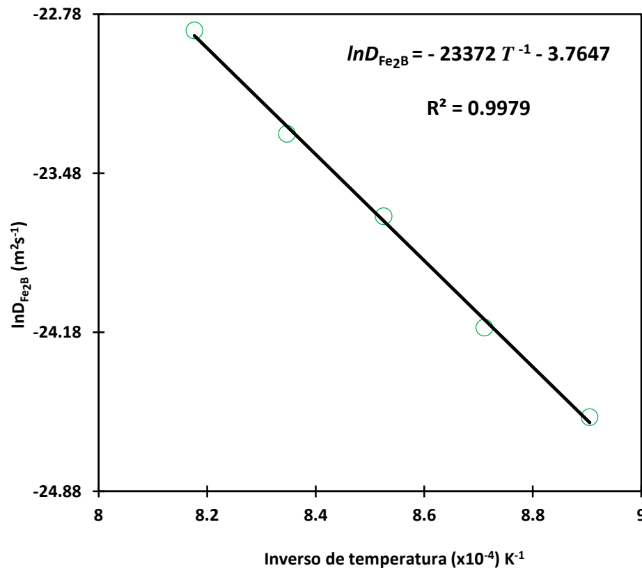
Figura V.21. Relación de Arrhenius para el coeficiente de difusión de boro ( D_{Fe_2B} ) a través de la capa de Fe_2B . Fuente: Autoría propia.
