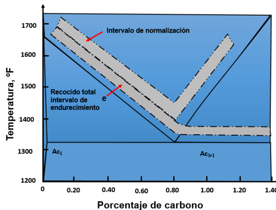
Figura I.1. Intervalo de recocido, normalizado y endurecimiento para aceros al carbono. Fuente: Autoría propia.
