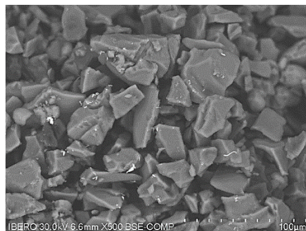
Figura V.7. Medio borurante en polvo ( \text{B}_4\text{C} + \text{KBF}_4 + \text{SiC} ). Fuente: Elias-Espinosa, M., Zuno-Silva, J. Ortiz-Domínguez, M. Hernández-Ávila, J. & Damián-Mejía O., 2015.
