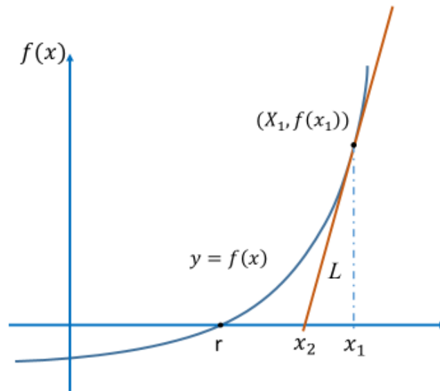
Figura III.5. Descripción gráfica del método de Newton-Raphson. Fuente: Autoría propia.
