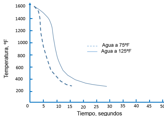
Figura I.3. Curvas de enfriamiento obtenidas en el centro de muestras templadas en agua a temperaturas de 75°F (24°C) y 125°F (52°C) sin agitación. Fuente: Autoría propia.
