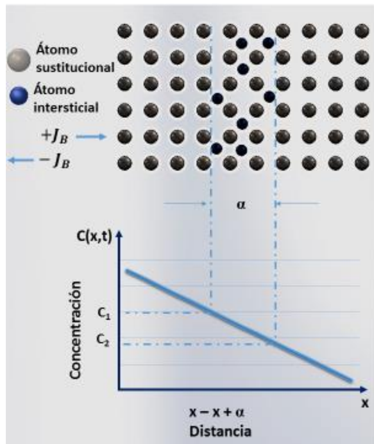
Figura II.6. Representación esquemática de la difusión unidireccional de átomos en una red cristalina. Fuente: Autoría propia.
