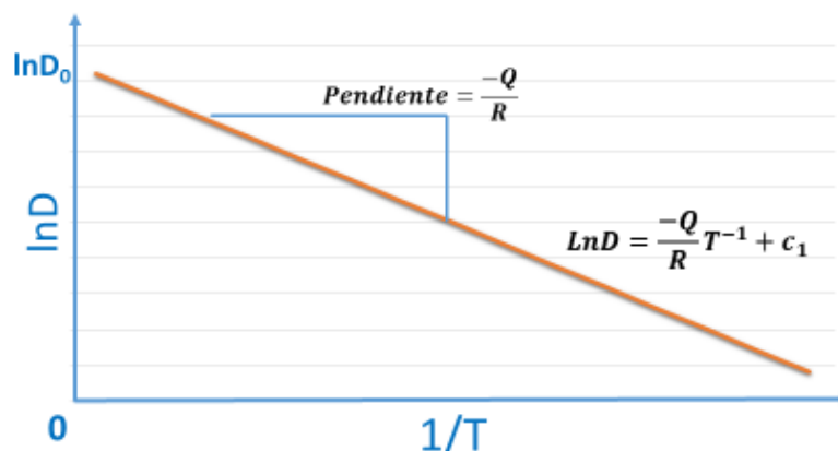
Figura II.8. Gráfica de pendiente de \ln D vs 1/T . Fuente: Autoría propia.
