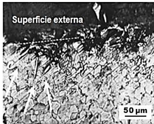
Figura V.4. Metalografía de una sección transversal de una muestra de hierro puro donde se puede apreciar cavidades en la superficie debido al crecimiento de cristales \text{Fe}_2\text{B} dentro del sustrato. Fuente: C. Martini, G. Palombarini, & M. Carbucicchio, 2004.
