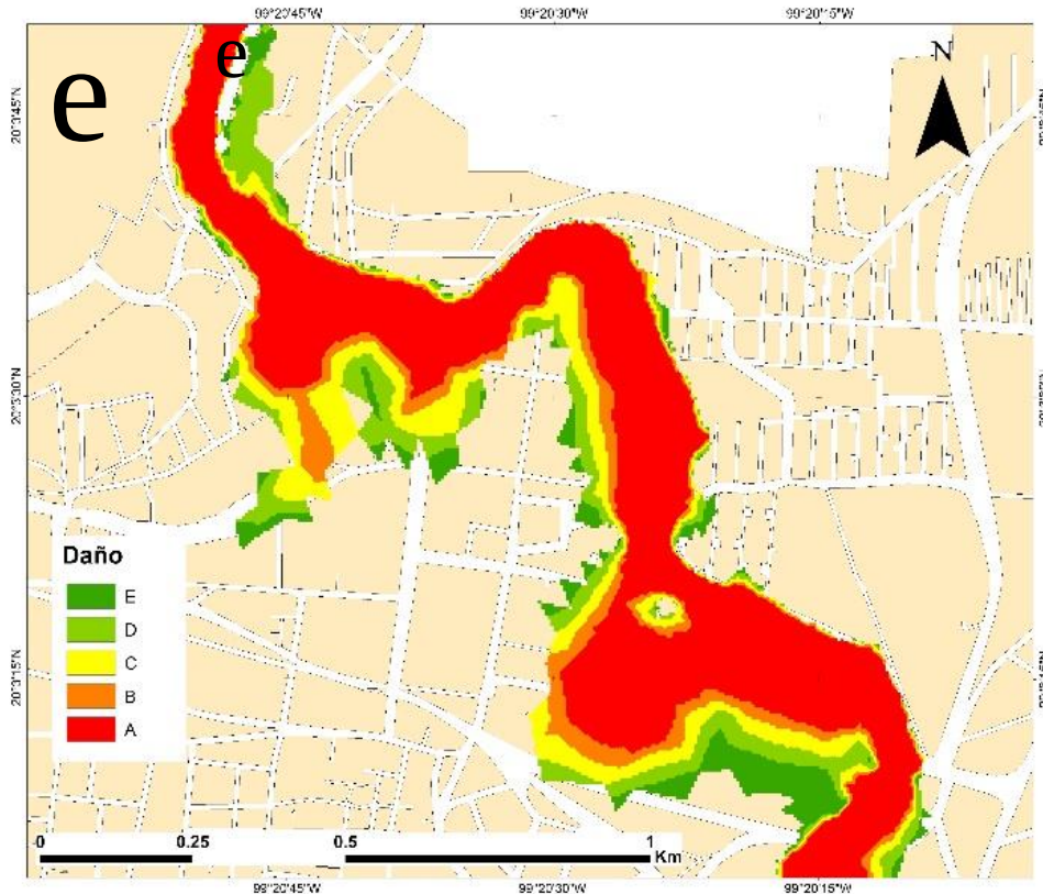
Figura 15. Mapas reclasificados de peligrosidad a diferentes periodos de retorno: a) 10 años b) 50 años c) 100 años d) 500 años e)1000 años.
