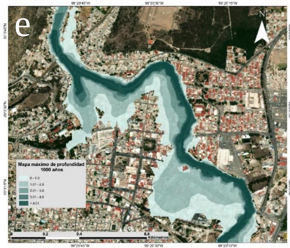
Figura 13. Mapas de profundidad a diferentes periodos de retorno: a) 10 años b) 50 años c) 100 años d) 500 años e)1000 años.
