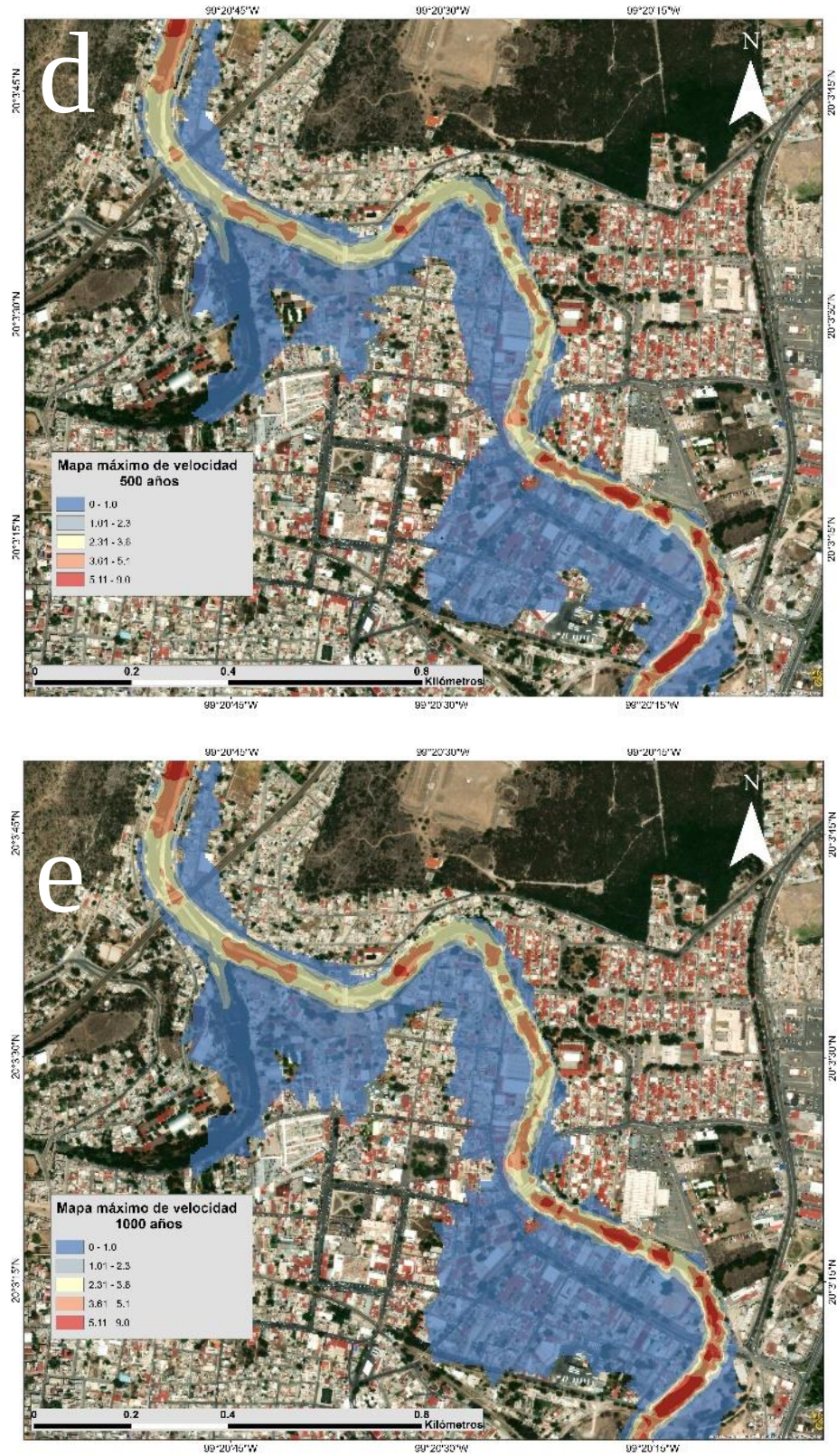
Figura 12. Mapas de velocidad a diferentes periodos de retorno: a) 10 años b) 50 años c) 100 años d) 500 años e) 1000 años.
