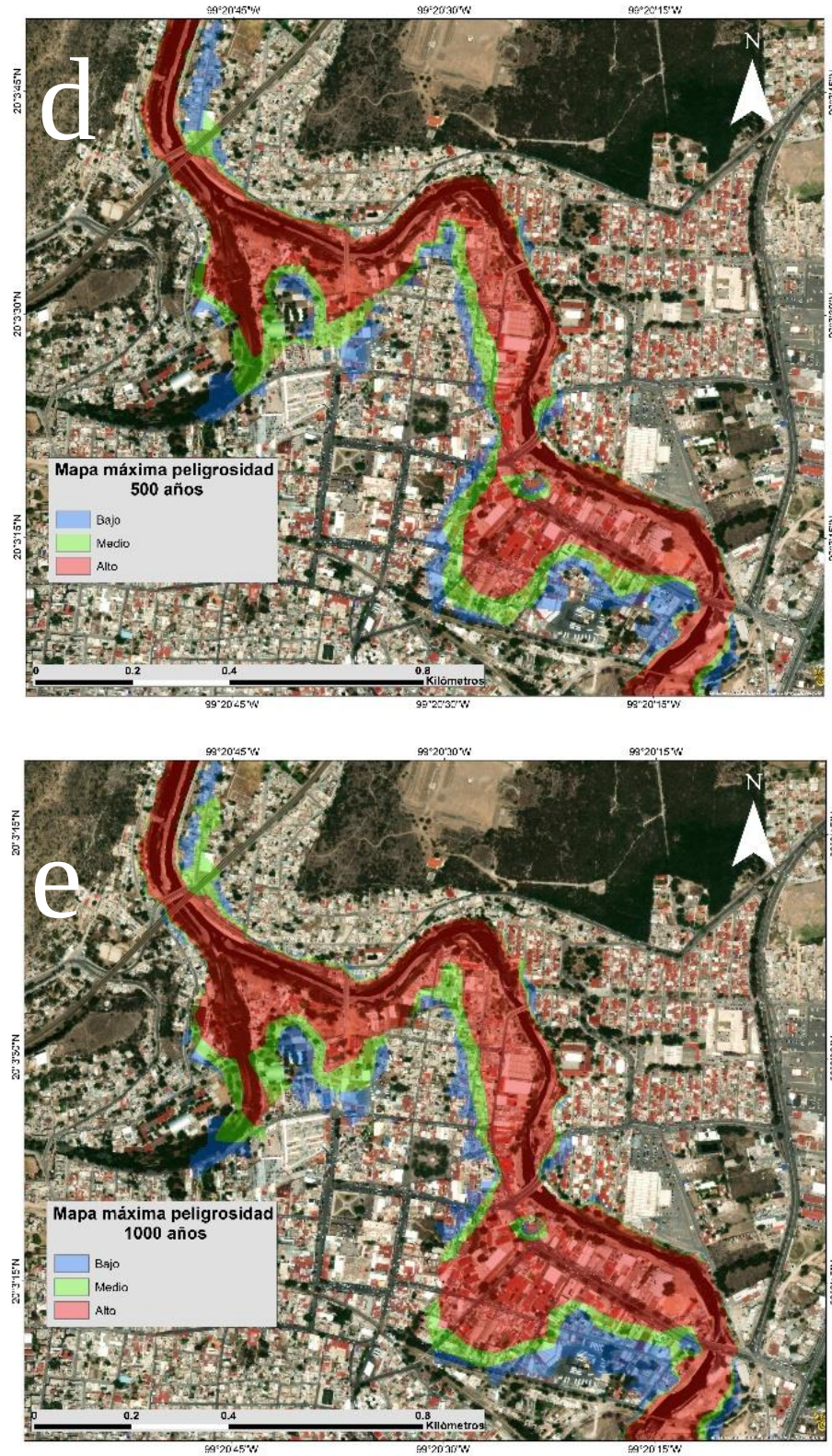
Figura 14. Mapas de peligrosidad a diferentes periodos de retorno: a) 10 años b) 50 años c) 100 años d) 500 años e) 1000 años.
