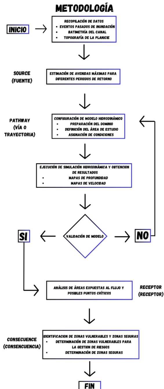
Figura 7. Metodología Source-Pathway-Receptor-Consequence.
