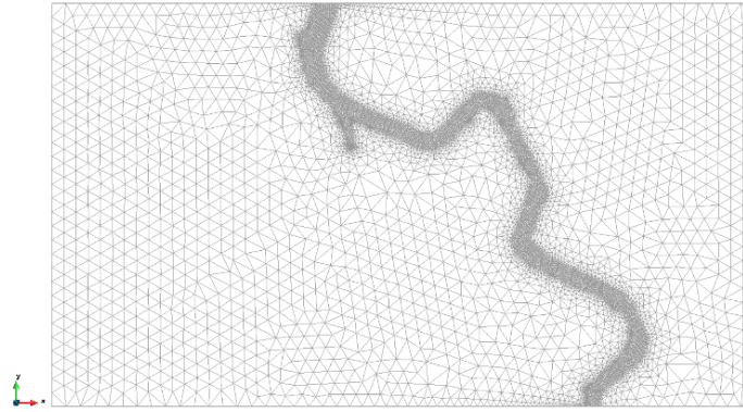
Figura 9. Malla de la planicie y batimetría del canal en Iber Model.
