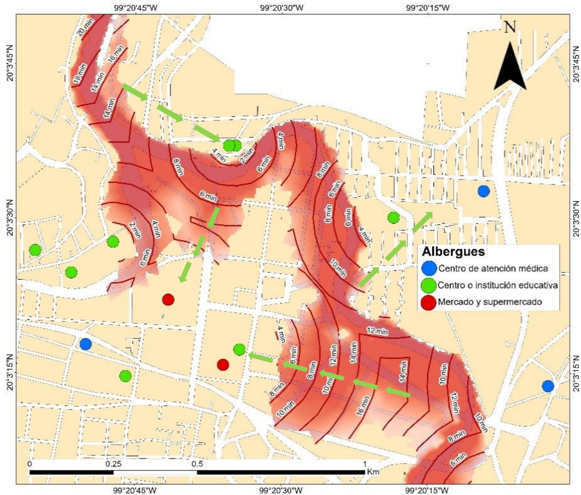
Figura 16. Tiempo necesario para evacuar la zona inundada hacia los albergues.
