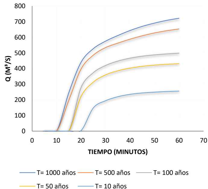
Figura 11. Hidrograma del Río Tula, aplicado a diferentes periodos de retorno.
