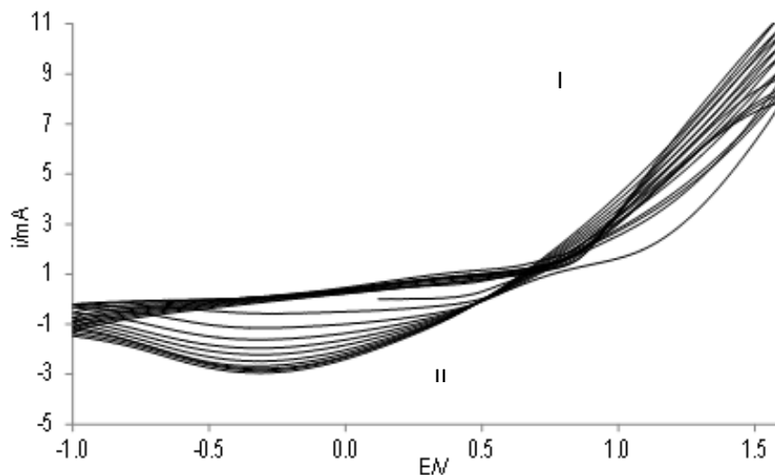
Figura 11. Voltamperograma cíclico obtenido utilizando una solución de Py 0.1 M. Utilizando una ventana de potencial de -1.0 a 1.5 V vs Ag/AgCl, a una velocidad de barrido de 0.05 V s -1 . Se realizaron 10 ciclos. Se utilizó un electrodo de grafito. I) Oxidación del monómero Py a partir de 0.8 V. II) Reducción de Ppy a Py en un valor de -0.3 V.
