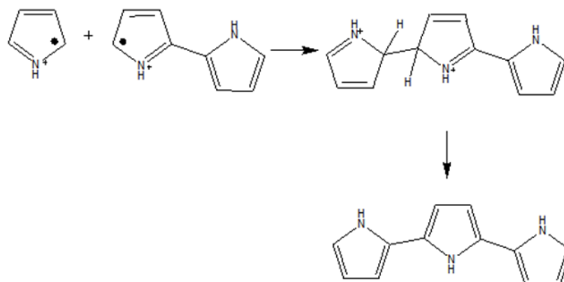
Figura B.6 Formación del trímero.
