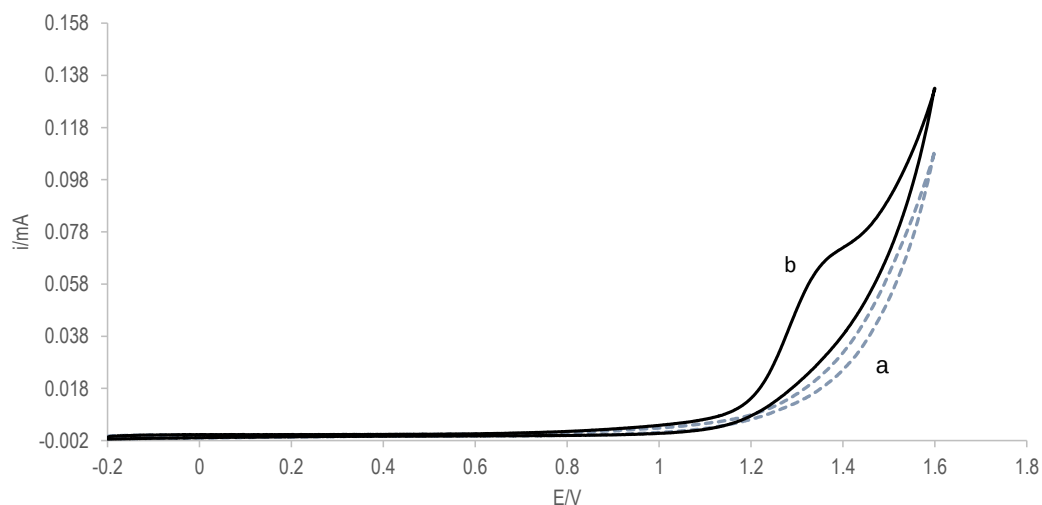
Figura 28. a) Voltamperograma cíclico para el sistema 0.5 M de \text{Na}_2\text{SO}_4 , 0.5 M de buffer de fosfatos, no se observan procesos redox asociados al electrolito soporte, b) voltamperograma cíclico para el sistema con ibuprofeno, se utilizó una ventana de potencial de -0.2 a 1.6 V a una velocidad de barrido de 0.05 \text{ V s}^{-1} . El barrido se realizó en sentido anódico.
