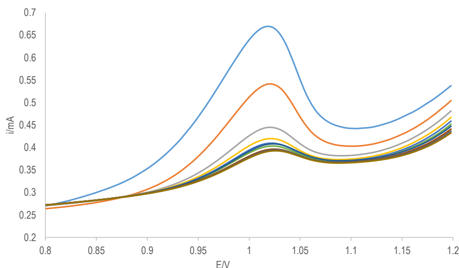
Figura 26. VDP ventana de potencial de 0.5 a 1.2 V vs Ag/AgCl, velocidad de barrido 0.012 V s -1 , se utilizó una solución 1 mM de ibuprofenato sódico en un buffer 0.5 M de fosfatos a pH 7.02 en Na 2 SO 4 0.5 M como electrolito soporte.
