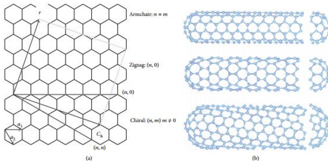
Figura 17. a) Estructura de un NTCP, b) estructuras de NTCP y las tres diferentes estructuras. Fuente: Saifuddin et al 2012.
