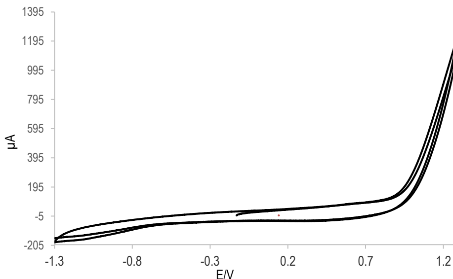
Figura 10. Voltamperograma cíclico obtenido para el ibuprofeno, utilizando una solución 0.1 M de ibuprofenato sódico y \text{NaNO}_3 0.1 M como electrolito soporte utilizando una ventana de potencial -1.3 a 1.3 V vs Ag/AgCl a una velocidad de barrido de 0.05 \text{ V s}^{-1} . Se empleó una barra de grafito como electrodo de trabajo.
