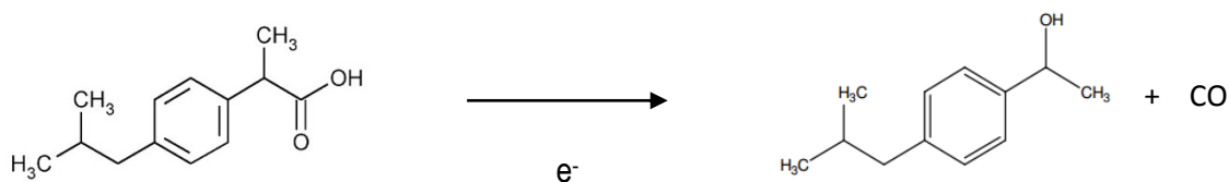
Figura 22. Proceso de oxidación del ibuprofeno con el reactivo de Fenton, al transferir un electrón se obtiene como producto de oxidación el (1-hidrooxietil)-4-isobutil-benceno.
