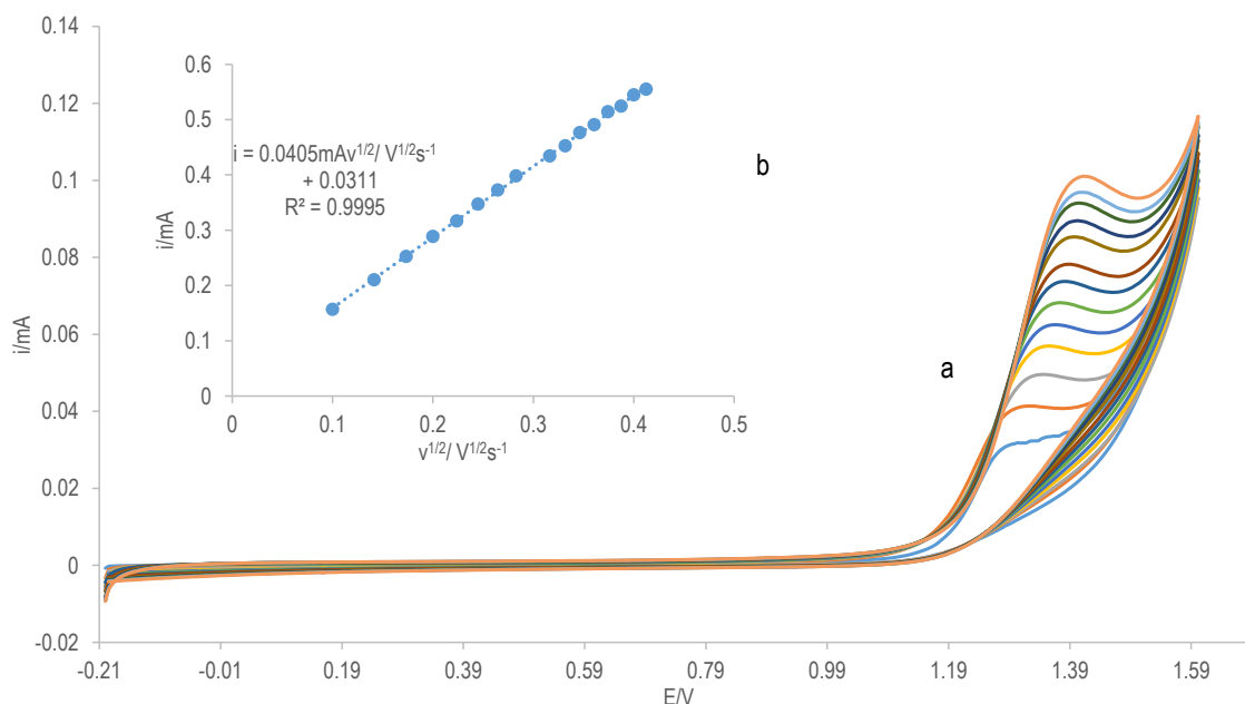
Figura 29. a) Voltamperogramas obtenidos a diferentes velocidades de barrido. b) Ajuste lineal al graficar la máxima intensidad de corriente anódica en función de la raíz cuadrada de la velocidad de barrido.
