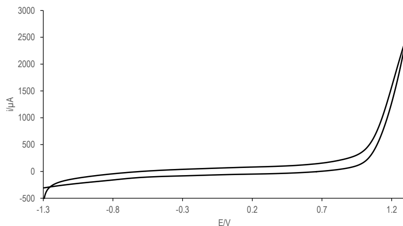
Figura 3. Voltamperograma cíclico obtenido utilizando un electrodo de barra de grafito. Ventana de potencial -1.3 a 1.3 vs Ag/AgClV. Velocidad de barrido 0.1 \text{ V s}^{-1} . Se empleó una solución 0.05 M de ibuprofenato sódico en 0.1 M de \text{NaNO}_3 como electrolito soporte.
