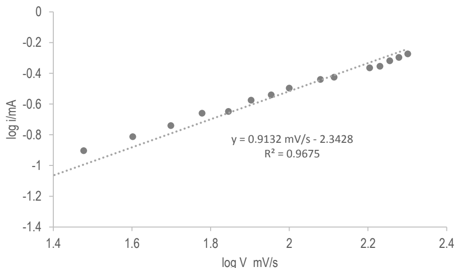
Figura 24. Ajuste lineal al graficar \log V vs \log i .
