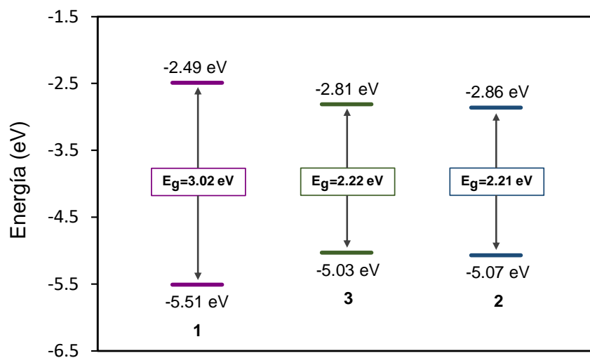
Figura 52. Diagrama de energía de los orbitales frontera calculados para los rotores 1 , 2 y 3 .
