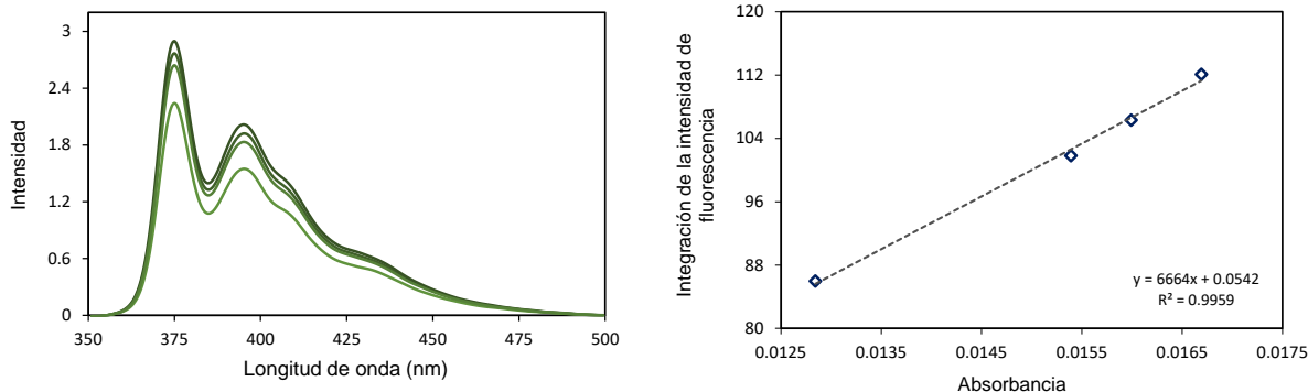
Figura 47. Espectros de emisión (izquierda) y gráfico de la integración de la intensidad de fluorescencia contra la absorbancia medida (derecha), usados para el cálculo del rendimiento cuántico del rotor molecular 3 en THF a temperatura ambiente.
