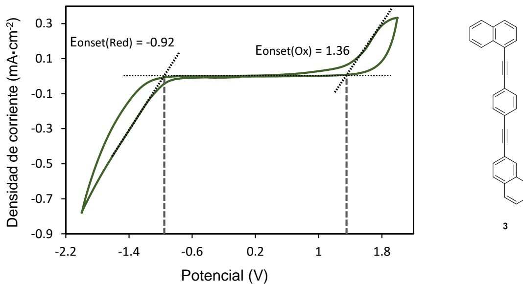
Figura K3. Voltamperograma cíclico del rotor molecular 1-[[4-(naftalen-2-iletinil)fenil]etinil]naftaleno ( 3 ) usando un sistema ITO/0.01 M de 3 + 0.1 M de perclorato de tetrabutilamonio en diclorometano anhidro a 20 mV s -1 .
