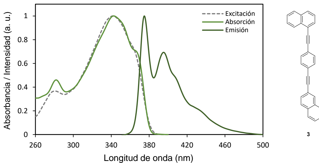
Figura J3. Espectro de absorción, excitación y emisión normalizado del rotor molecular 1-[[4-(2-naftalen-2-iletinil)fenil]etinil]naftaleno ( 3 ) en THF.
