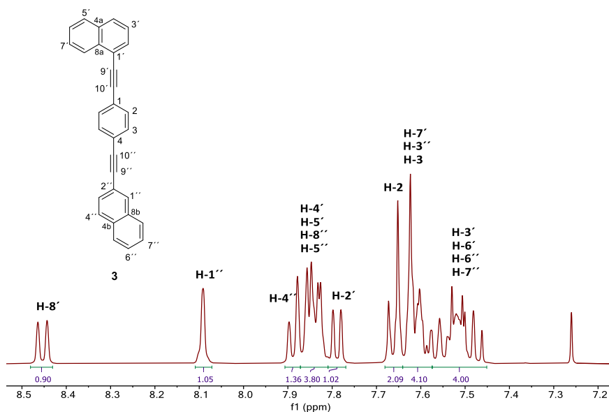
Figura 30. Espectro de RMN de ^1\text{H} del rotor molecular 1-[[4-naftalen-2-iletinil]fenil]etinil}naftaleno ( 3 ) adquirido a 400 MHz en \text{CDCl}_3 a 25 °C.
