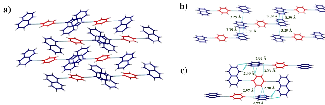
Figura 36. a) Empaquetamiento del rotor molecular 1 con estructura de tipo “cabeza-cola” formada por b) interacciones \pi\cdots\pi entre los anillos de naftaleno y c) interacciones C-H \cdots\pi entre el rotador y los estatores.
