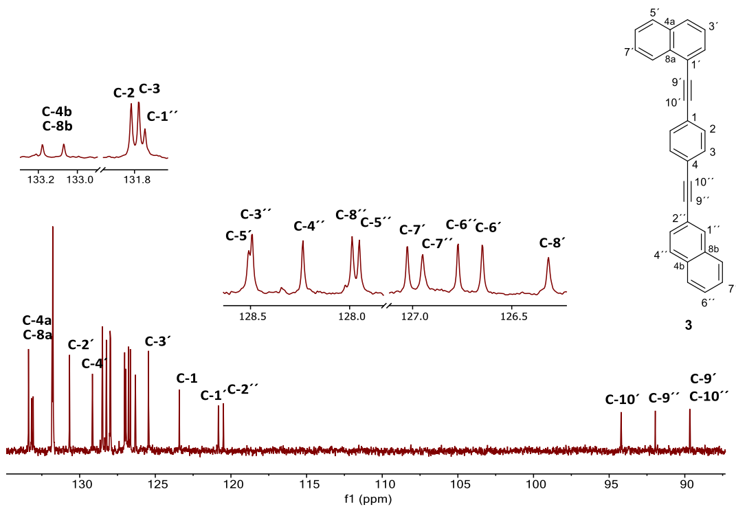
Figura H43. Espectro de RMN de ^{13}\text{C} del rotor molecular 1-[[4-naftalen-2-iletinil]fenil]etinil]naftaleno ( 3 ) adquirido a 101 MHz en \text{CDCl}_3 a 25 °C.
