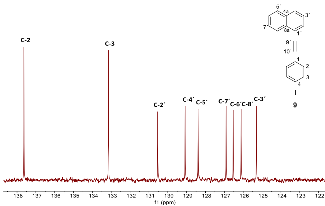
Figura H37. DEPT-135 del 1-[(4-yodofenil)etnil]naftaleno ( 9 ) adquirido a 101 MHz en \text{CDCl}_3 a 25 °C.
