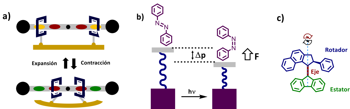
Figura 3. Colección de máquinas moleculares que pueden generar trabajo: a) Interruptores electroquímicos basados en rotaxanos biestables unidos a una superficie de oro que pueden inducir su expansión o contracción; b) Bajo irradiación de luz los azobencenos isomerizan E \rightarrow Z , resultando en una fuerza F y un desplazamiento \Delta p del objeto A; c) Estructura de un motor molecular que al ser iluminado con luz UV puede provocar la rotación de pequeños objetos macroscópicos sobre una superficie de cristales líquidos. Figura adaptada de la referencia 9.
