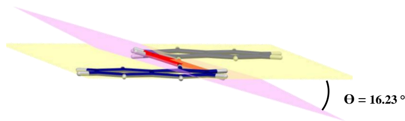
Figura 35. Estructura molecular del rotor 1 y ángulo interplanar generado por la intersección del plano del anillo de fenileno (violeta) con respecto al plano de los estatores (amarillo).
