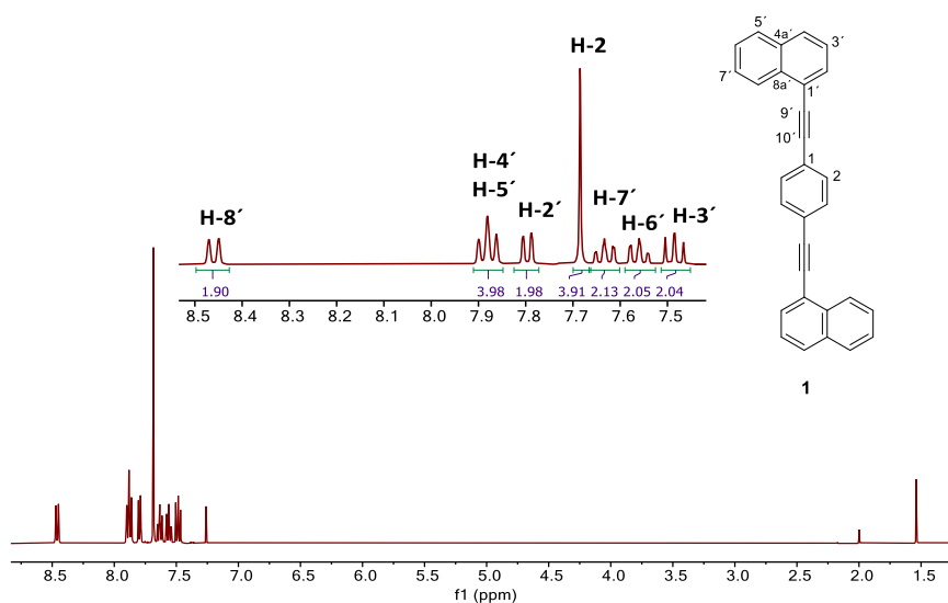
Figura 22. Espectro de RMN de ^1\text{H} del rotor molecular 1,4-bis(naftalen-1-iletinil)benceno ( 1 ) adquirido a 400 MHz en \text{CDCl}_3 a 25 ^\circ\text{C} .
