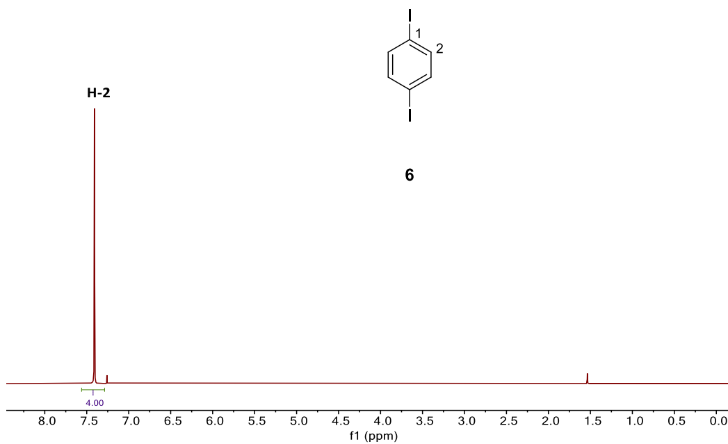
Figura H9. Espectro de RMN de 1 H del 1,4-diyodobenceno ( 6 ) adquirido a 400 MHz en CDCl 3 a 25 °C.
