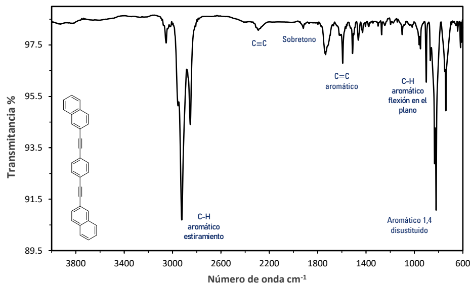
Figura 28. Espectro de infrarrojo del rotor molecular 1,4-bis(naftalen-2-iletinil)benceno ( 2 ) en película.
