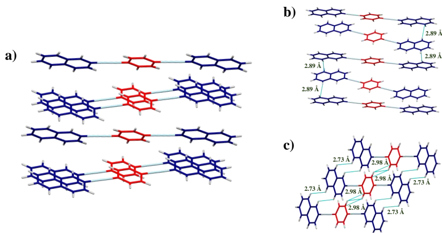
Figura 38. a) Empaquetamiento del rotor molecular 2 con b) interacciones C-H \cdots\pi entre los anillos de naftaleno y c) interacciones entre los hidrógenos del fragmento 2-naftilo y del rotor.
