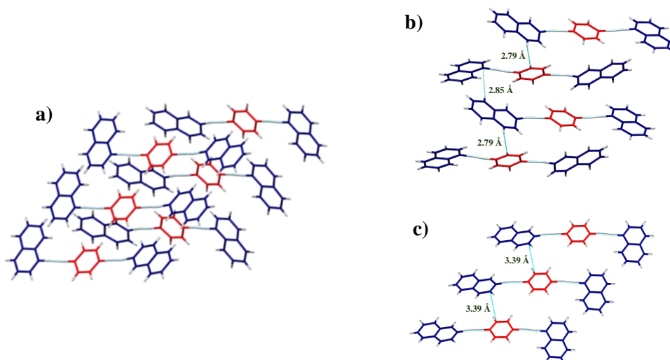
Figura 40. a) Empaquetamiento del rotor molecular 3 de tipo "borde-cara" causado por las b) interacciones C-H \cdots \pi entre los anillos de naftaleno y c) interacciones entre los hidrógenos del fragmento 2-naftilo y del rotor al apilarse.
