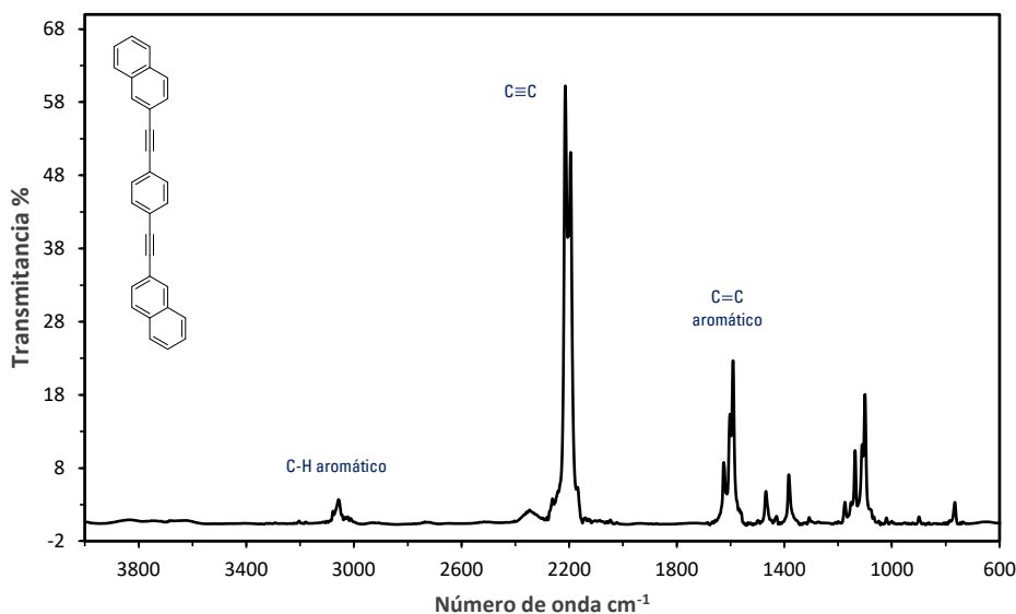
Figura 29. Espectro Raman del rotor molecular 1,4-bis(naftalen-2-iletinil)benceno ( 2 ).
