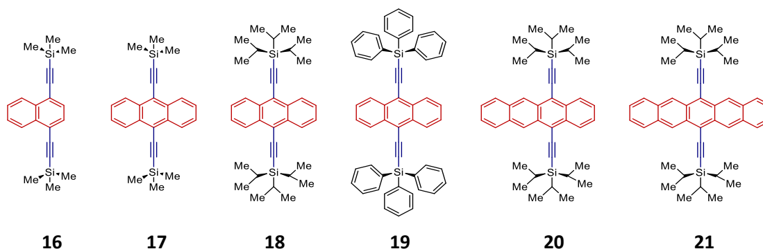
Figura 19. Rotores moleculares sintetizados por Howe y col. con estatores de trialquilsililo y triarilsililo (negro) y enlaces triples como conectores (azul) de la parte móvil y los estatores. Para los rotadores se usaron los acenos de naftaleno ( 16 ), antraceno ( 17 , 18 , 19 ), tetraceno ( 20 ) y pentaceno ( 21 ). Figura adaptada de la referencia 46.
