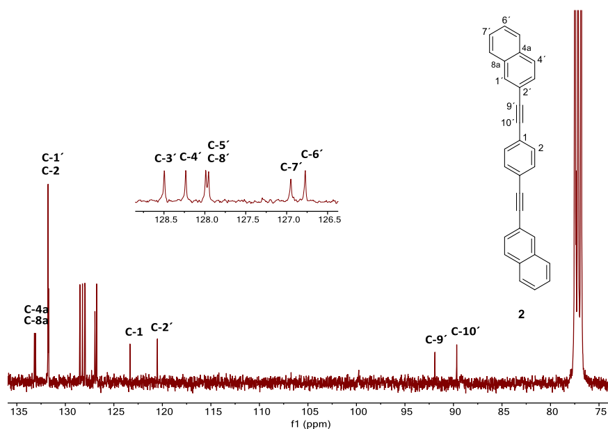
Figura 27. Espectro de RMN de ^{13}\text{C} del rotor molecular 1,4-bis(naftalen-2-iletinil)benceno ( 2 ) adquirido a 101 MHz en \text{CDCl}_3 a 25 °C.
