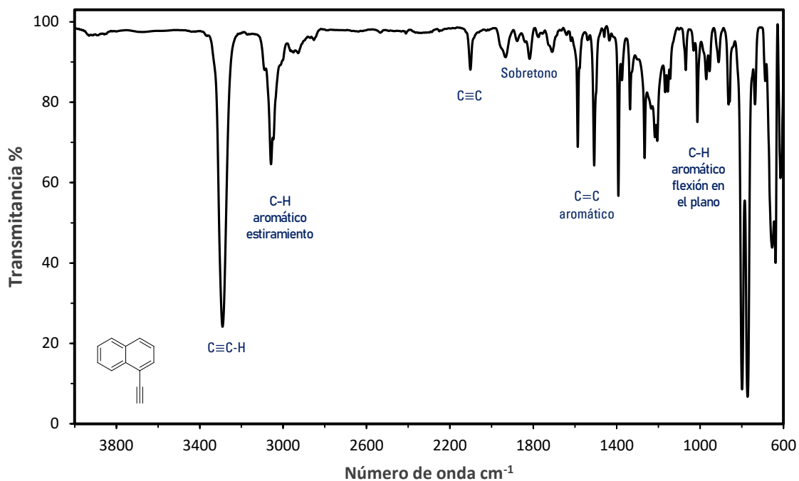
Figura H8. Espectro de infrarrojo del 1-etinilnaftaleno ( 5 ) en película.
