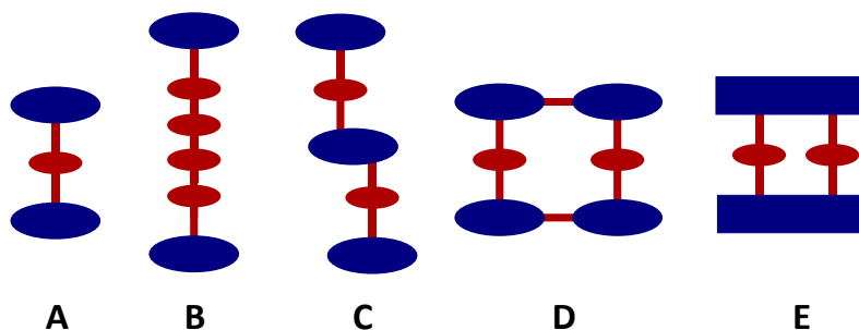
Figura 8. Representación esquemática de rotores moleculares donde un estator voluminoso (azul) genera un espacio libre para el rotador (rojo) y permite la rotación. Figura adaptada de la referencia 24.
