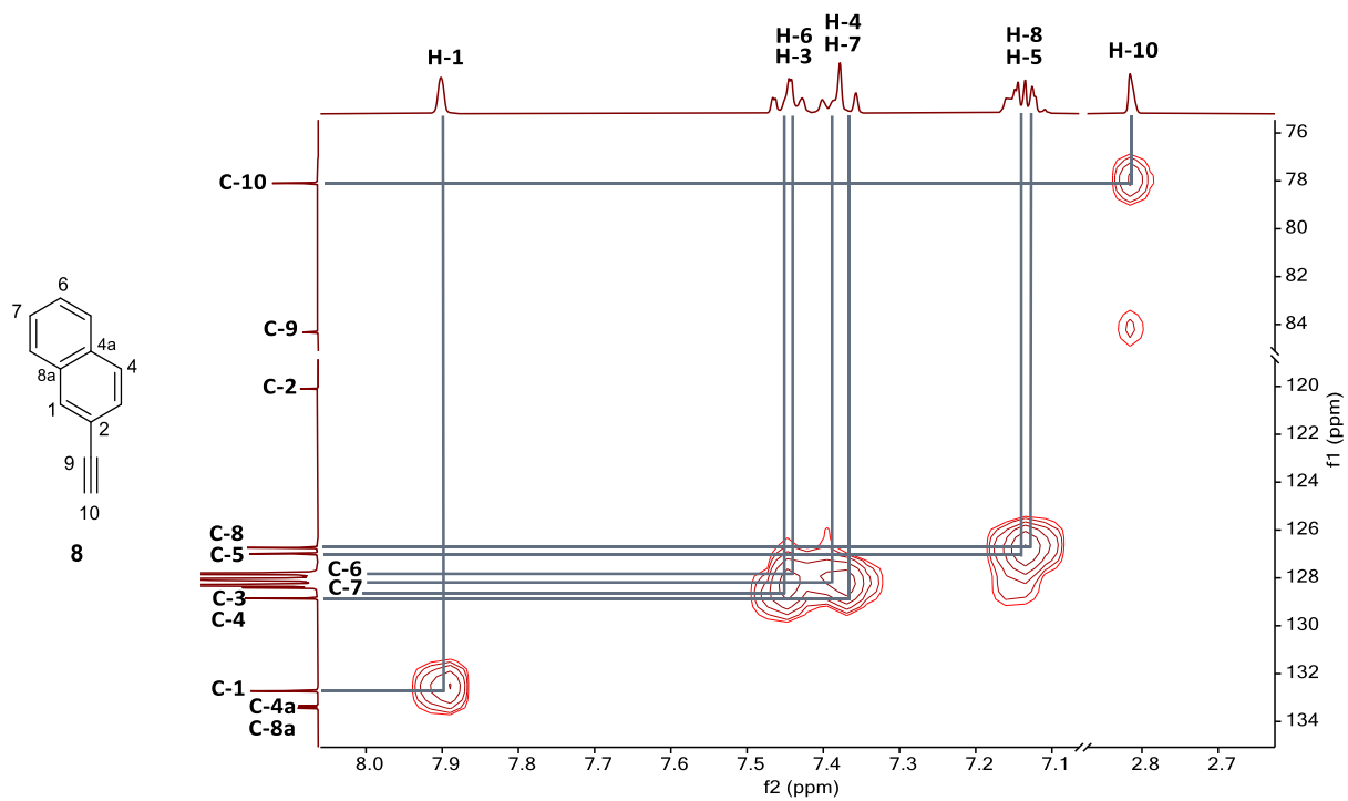
Figura H28. Espectro HSQC del 2-etinilnaftaleno ( 8 ) en C 6 D 6 a 25 °C.
