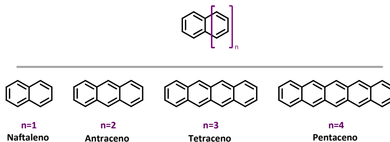
Figura 14. Acenos formados por la unión de anillos bencénicos. Considerando la condición de n \geq 1 se pueden formar los acenos de naftaleno ( n=1 ), antraceno ( n=2 ), tetraceno ( n=3 ), entre otros. Acenos con n superiores a 7 necesitan de condiciones especiales para su formación y/o estabilidad en el estado sólido. Figura adaptada de la referencia 36.
