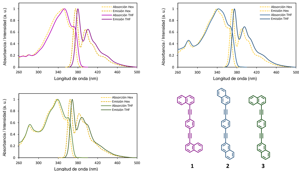
Figura 44. Espectros de absorción y emisión de los rotores moleculares 1 , 2 y 3 normalizados en hexano (línea punteada) y THF (línea sólida) a temperatura ambiente.
