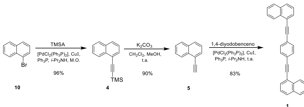
Esquema 2. Síntesis del rotor molecular 1,4-bis(naftalen-1-iletinil)benceno (1).
