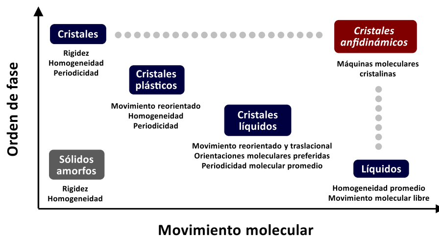
Figura 5. Diagrama que correlaciona la dinámica de la materia condensada y el orden de fase con el movimiento molecular. Figura adaptada de la referencia 25.
