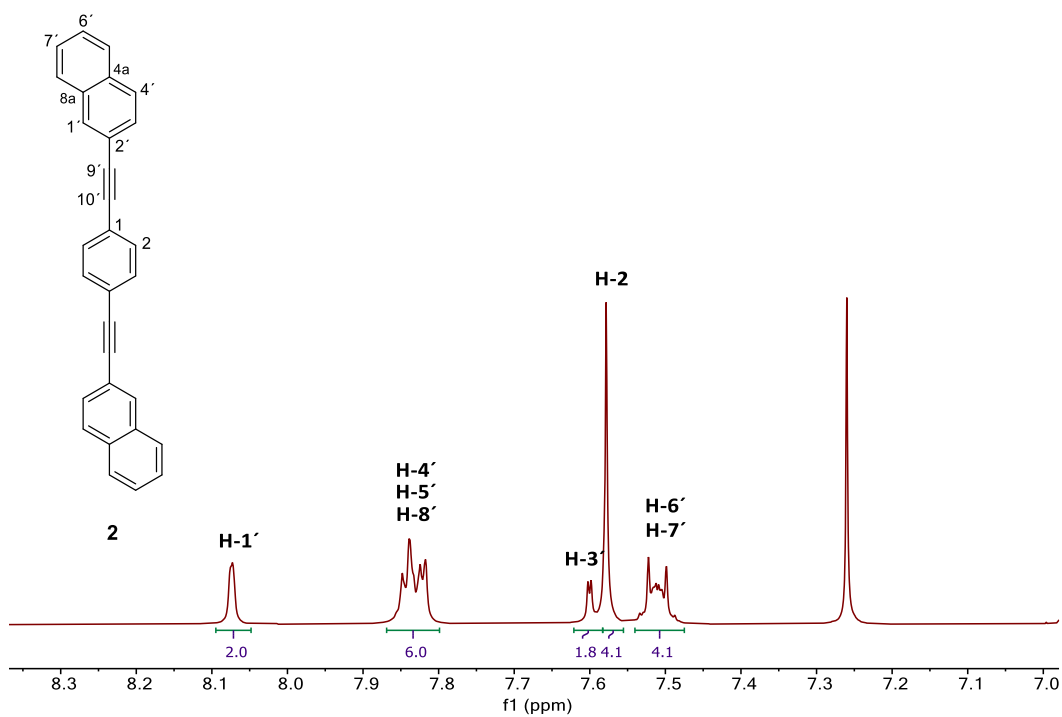
Figura H31. Espectro de RMN de ^1\text{H} del rotor molecular 1,4-bis(naftalen-2-iletinil)benceno ( 2 ) adquirido a 400 MHz en \text{CDCl}_3 a 25 °C.
