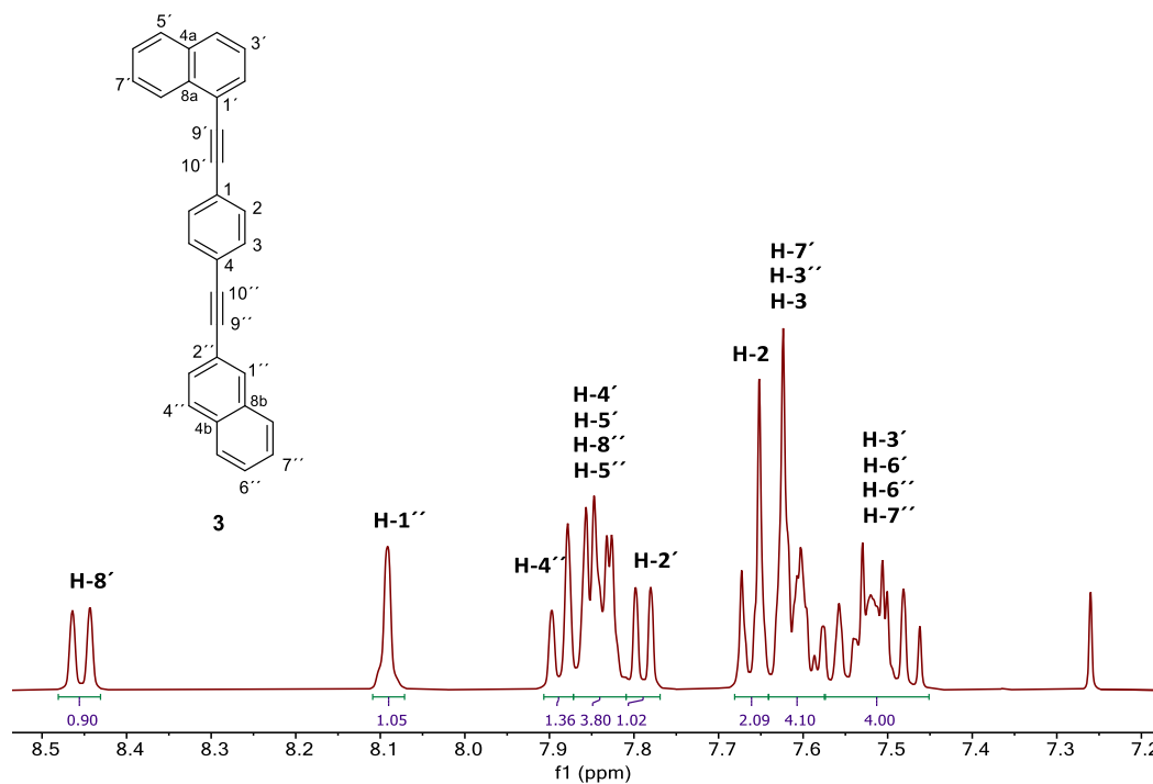
Figura H42. Espectro de RMN de ^1\text{H} del rotor molecular 1-[[4-naftalen-2-iletinil]fenil]etnil]naftaleno ( 3 ) adquirido a 400 MHz en \text{CDCl}_3 a 25 °C.
