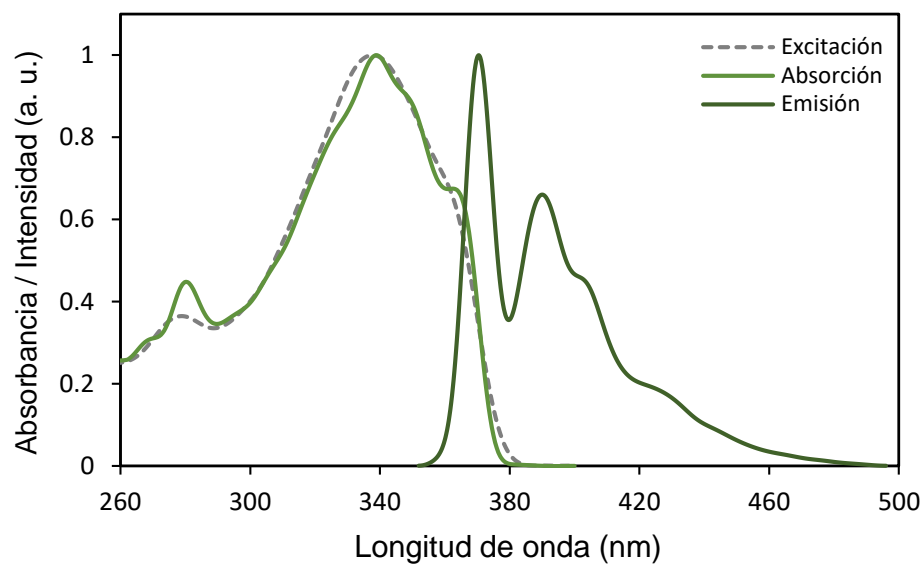
Figura J6. Espectro de excitación y emisión normalizado del rotor molecular 1-[(4-naftalen-2-iletinil)fenil]etinil}naftaleno ( 3 ) en n -hexano.
