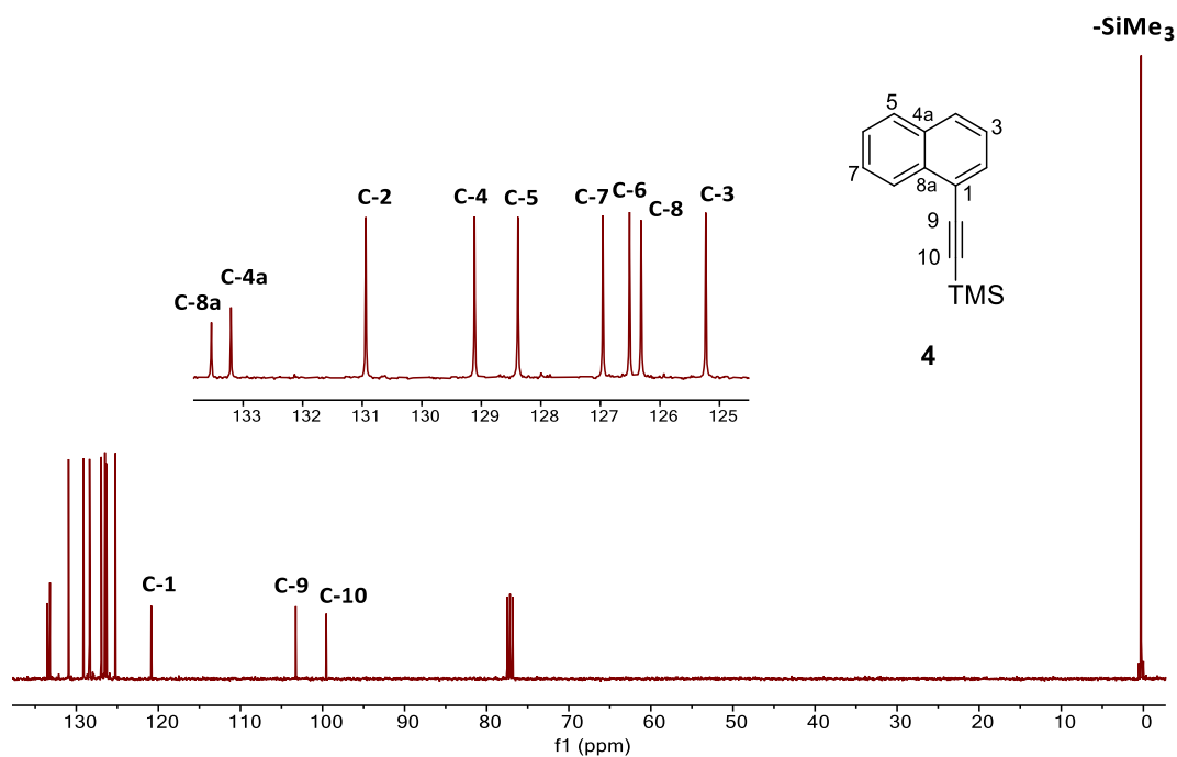
Figura H2. Espectro de RMN de ^{13}\text{C} del 1-(trimetilsilil)etnilnaftaleno ( 4 ) adquirido a 101 MHz en \text{CDCl}_3 a 25^\circ\text{C} .
