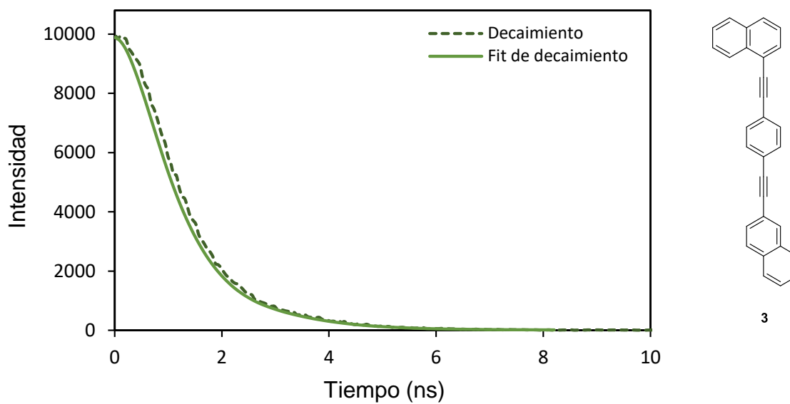
Figura J12. Curva de decaimiento de fluorescencia experimental y ajuste exponencial para el rotor molecular 1-[[4-(2-naftalen-2-iletinil)fenil]etinil]naftaleno ( 3 ).
