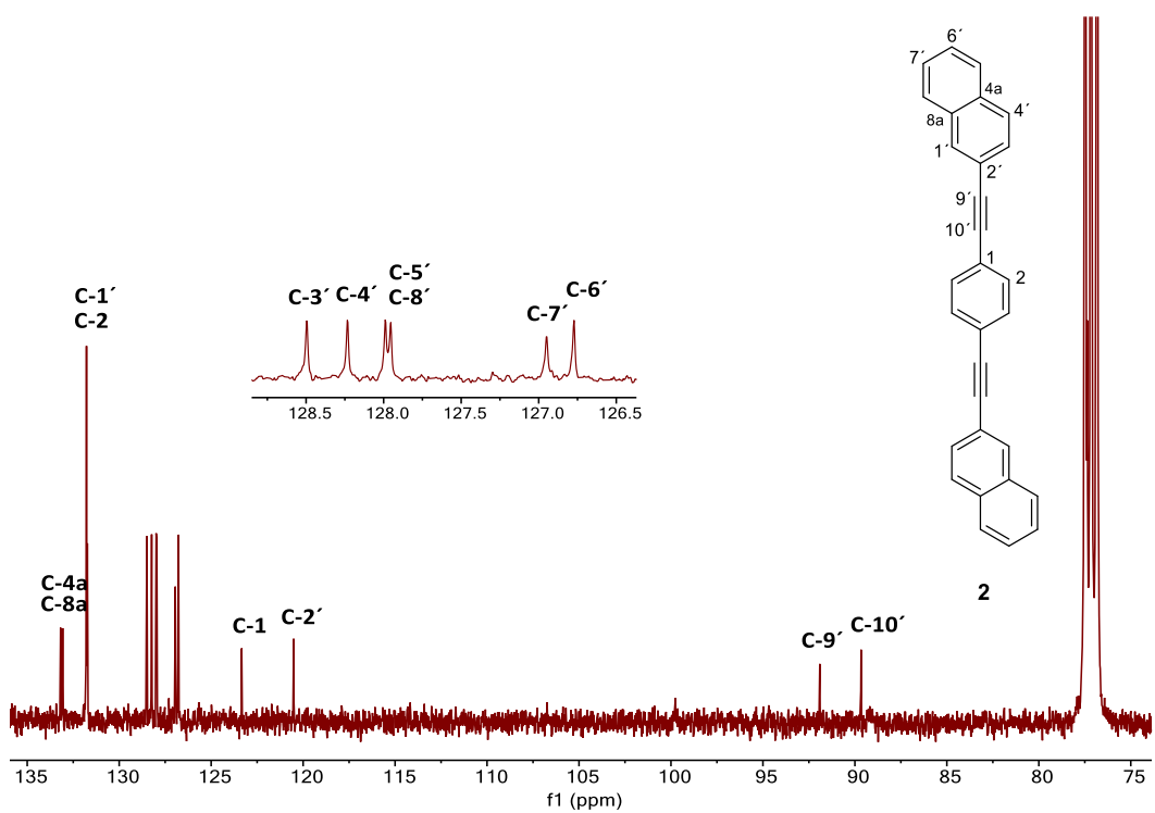
Figura H32. Espectro de RMN de ^{13}\text{C} del rotor molecular 1,4-bis(naftalen-2-iletinil)benceno ( 2 ) adquirido a 101 MHz en \text{CDCl}_3 a 25 °C.
