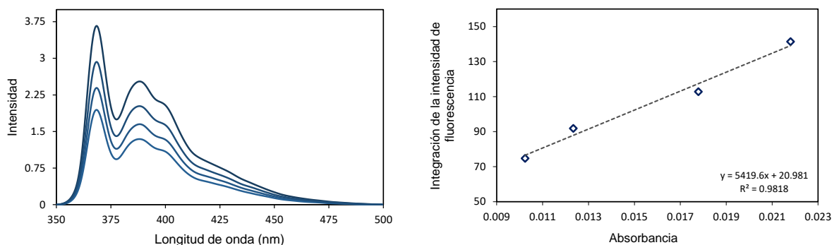
Figura 46. Espectros de emisión (izquierda) y gráfico de la integración de la intensidad de fluorescencia contra la absorbancia medida (derecha), usados para el cálculo del rendimiento cuántico del rotor molecular 2 en THF a temperatura ambiente.
