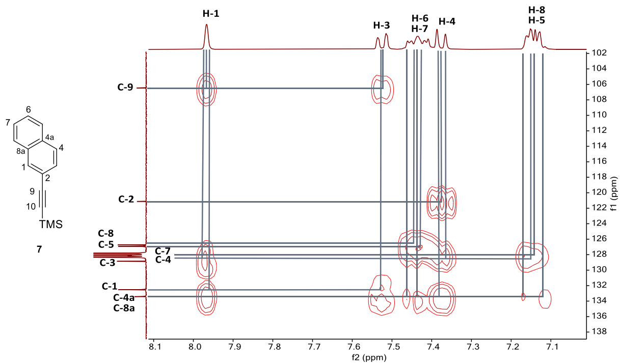
Figura H22. Espectro HMBC del 2-(trimetilsilil)etnilnaftaleno ( 7 ) en C_6D_6 a 25 °C.
