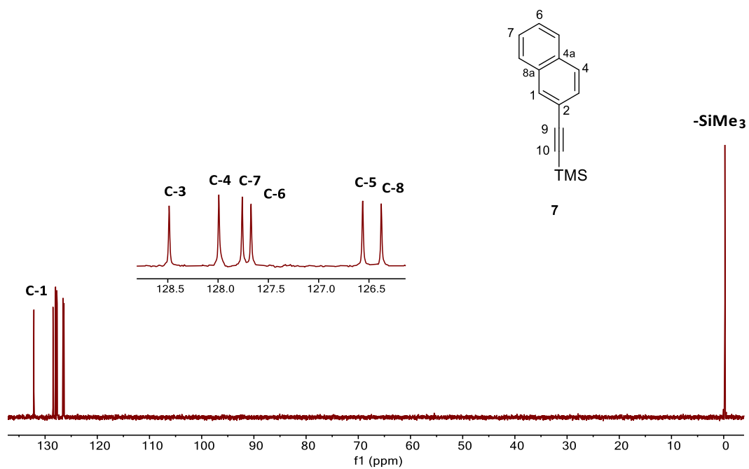
Figura H19. Espectro de RMN de ^{13}\text{C} experimento DEPT-135 del 2-(trimetilsilil)etnilnaftaleno ( 7 ) adquirido a 101 MHz en \text{C}_6\text{D}_6 a 25 °C.
