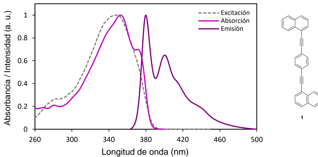
Figura J1. Espectro de absorción, excitación y emisión normalizado del rotor molecular 1,4-bis(naftalen-1-iletinil)benceno ( 1 ) en THF.
