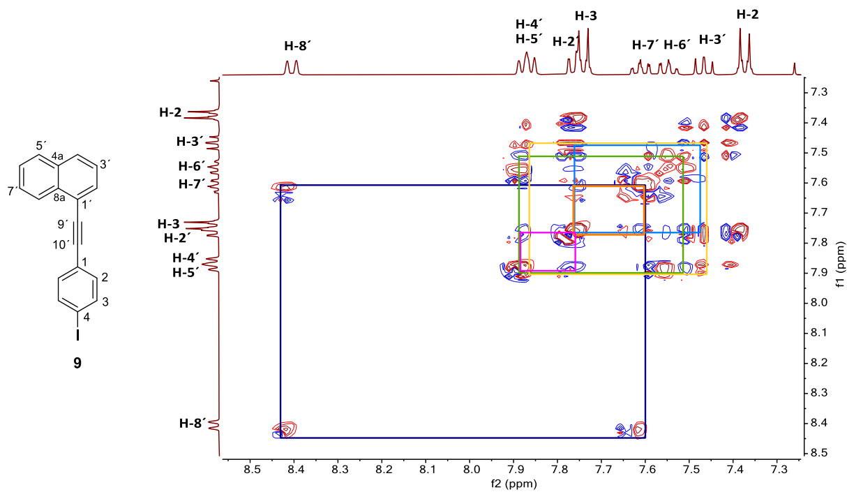
Figura H38. Espectro COSY del 1-[(4-yodofenil)etnil]naftaleno ( 9 ) en \text{CDCl}_3 a 25 °C.
