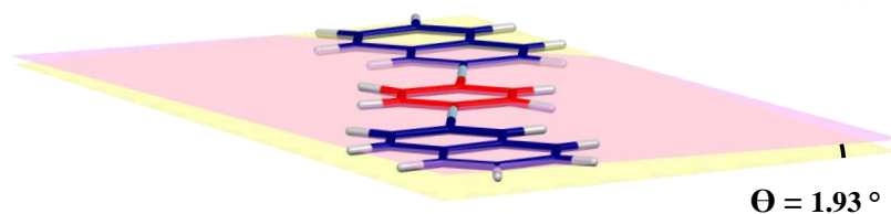
Figura 37. Estructura molecular del rotor 2 ángulo interplanar generado entre los planos.
