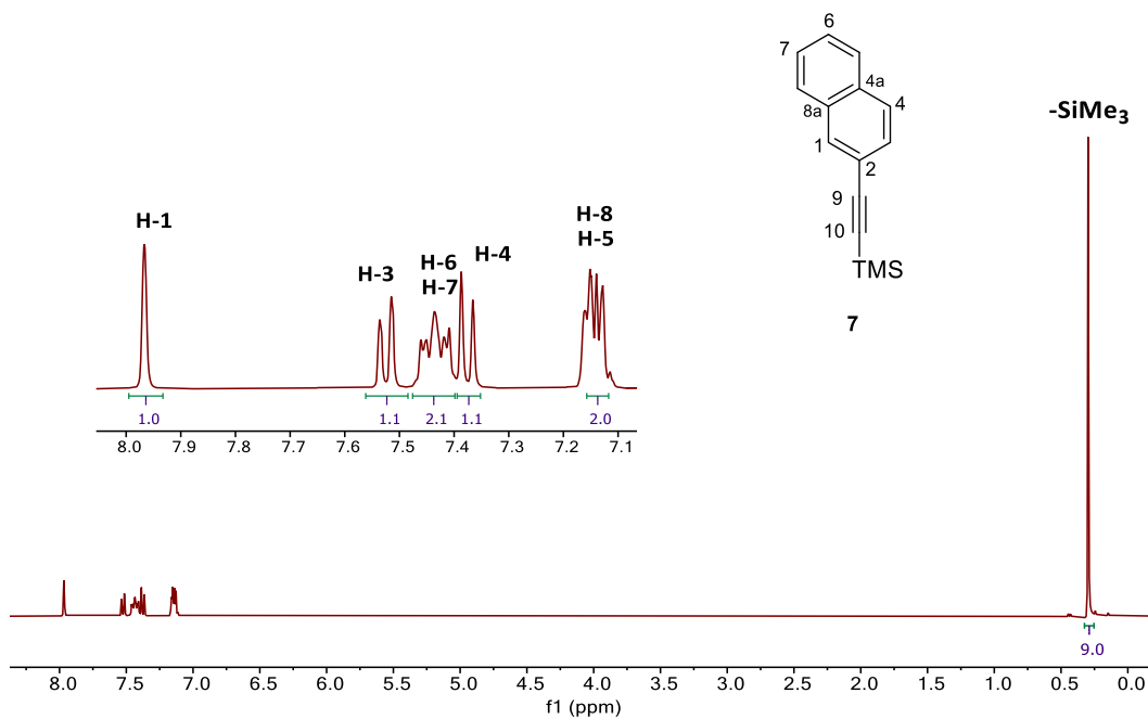
Figura H17. Espectro de RMN de ^1\text{H} del 2-(trimetilsilil)etininftaleno ( 7 ) adquirido a 400 MHz en \text{C}_6\text{D}_6 a 25^\circ\text{C} .
