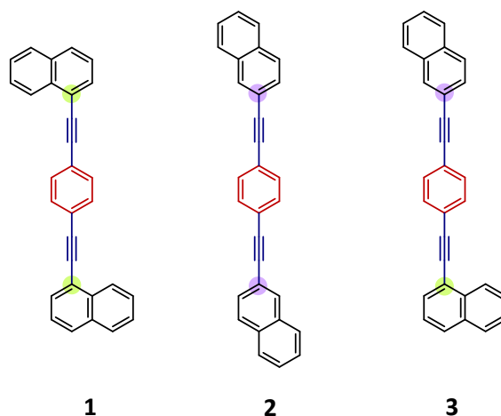
Figura 21. Rotores moleculares 1 , 2 y 3 sintetizados donde se encuentra sombreado en verde la unión del fragmento 1-naftilo y en morado el 2-naftilo como estatores (negro) al eje (azul) de cada rotor. El rotador de fenileno (rojo) es el mismo para todos los casos.
