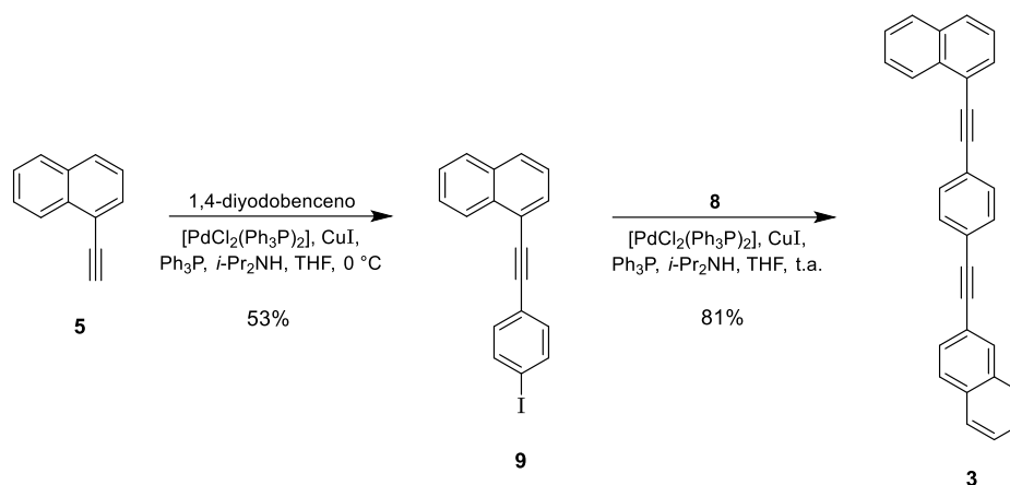
Esquema 6. Síntesis del rotor molecular 1-{[(4-naftalen-2-iletinil)fenil]etinil}naftaleno ( 3 ).
