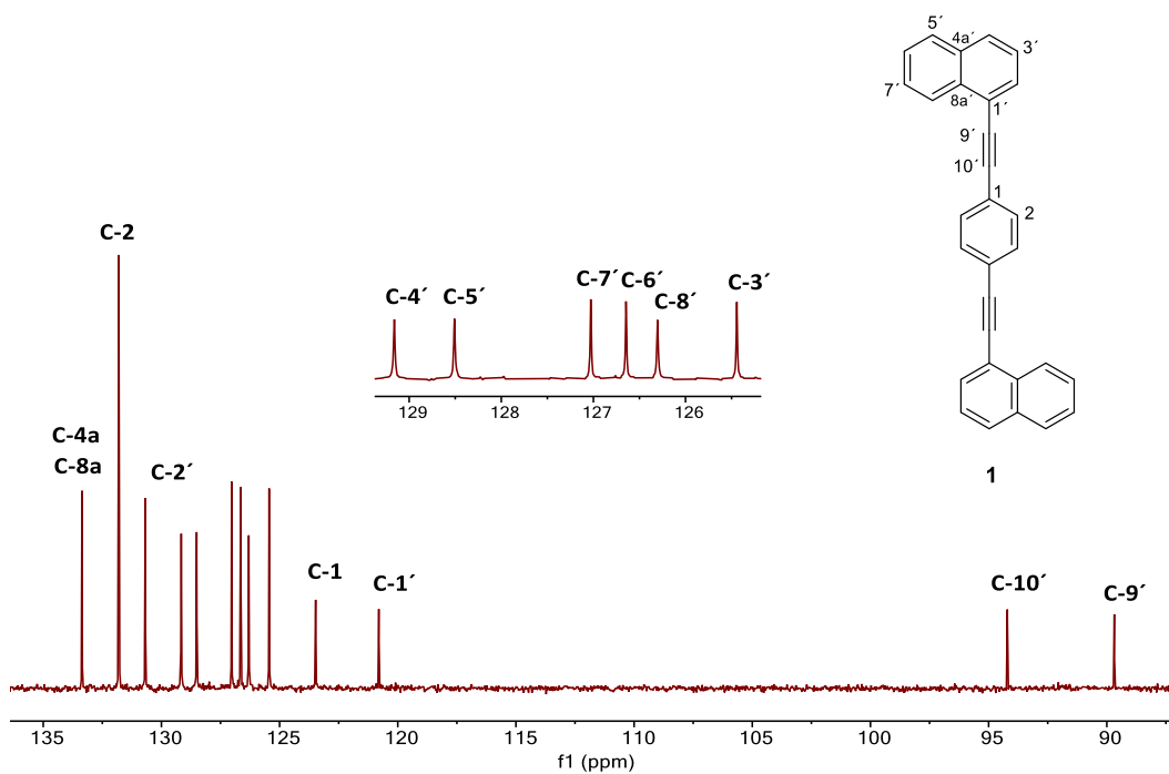
Figura H13. Espectro de RMN de ^{13}\text{C} del rotor molecular 1,4-bis(naftalen-1-iletinil)benzeno ( 1 ) adquirido a 101 MHz en \text{CDCl}_3 a 25^\circ\text{C} .
