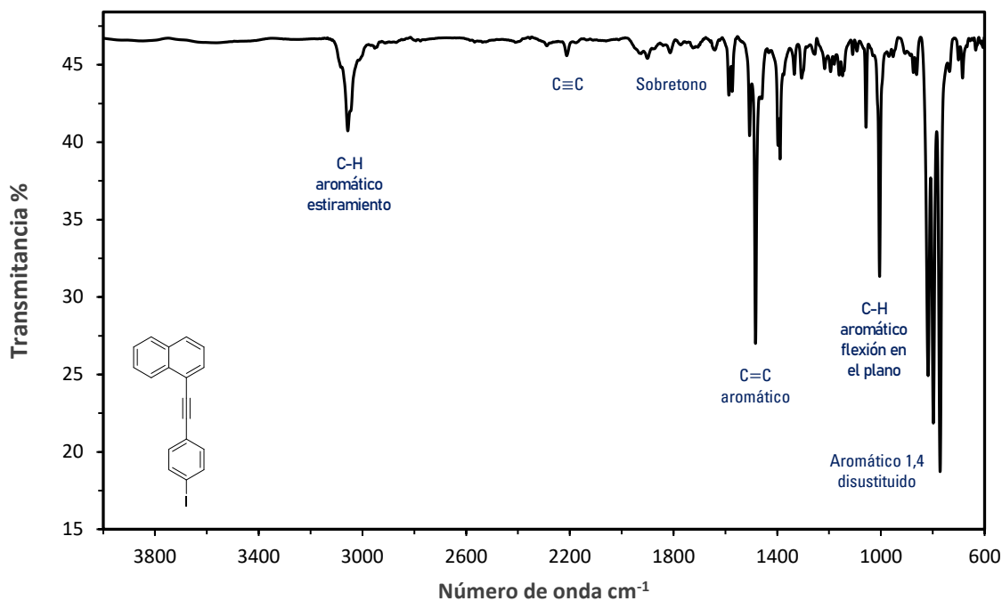
Figura H41. Espectro de infrarrojo del 1-[(4-yodofenil)etnil]naftaleno ( 9 ) en película.
