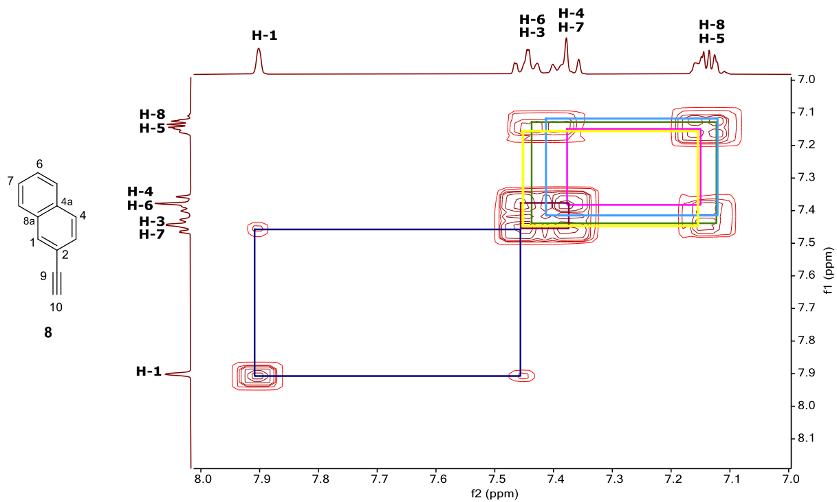
Figura H27. Espectro COSY del 2-etinilnaftaleno ( 8 ) en C 6 D 6 a 25 °C.
