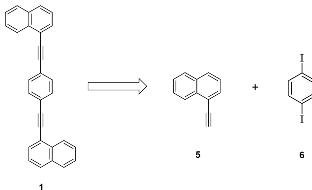
Esquema 1. Retrosíntesis para la obtención del rotor molecular 1,4-bis(naftalen-1-iletinil)benceno (1) a partir de los sintones 1-etinilnaftaleno (5) y 1,4-diyodobenceno (6).
