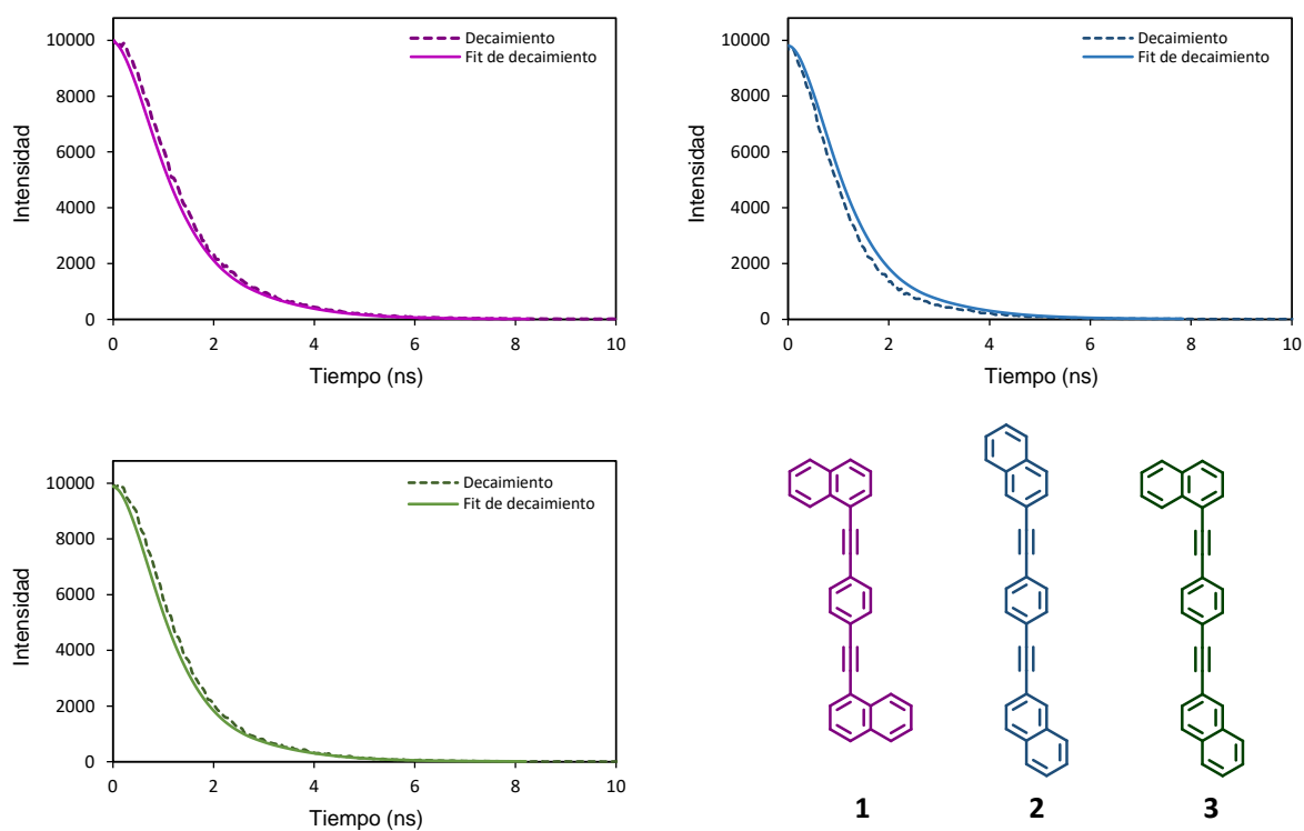
Figura 48. Curvas de decaimiento de fluorescencia experimental (línea entrecortada) y curva calculada (línea sólida) para las soluciones de los rotores moleculares 1 , 2 y 3 en THF.
