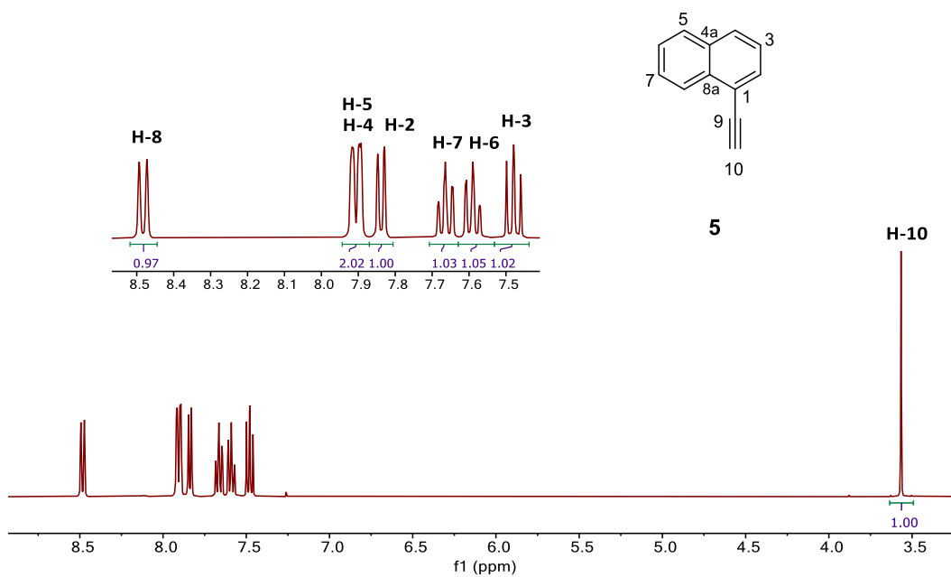
Figura H5. Espectro de RMN de ^1\text{H} del 1-etinilnaftaleno ( 5 ) adquirido a 400 MHz en \text{CDCl}_3 a 25 ^\circ\text{C} .
