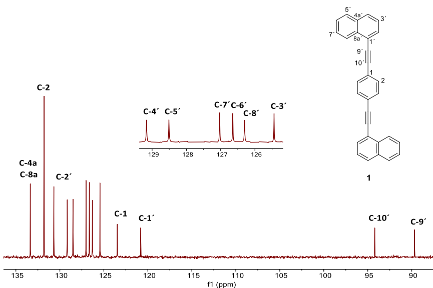
Figura 23. Espectro de RMN de ^{13}\text{C} del rotor molecular 1,4-bis(naftalen-1-iletinil)benceno ( 1 ) adquirido a 101 MHz en \text{CDCl}_3 a 25 ^\circ\text{C} .
