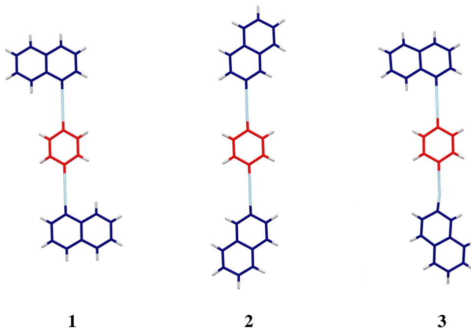
Figura 34. Estructuras moleculares de los rotores 1 , 2 y 3 obtenidos a través de difracción de rayos X de monocristal.
