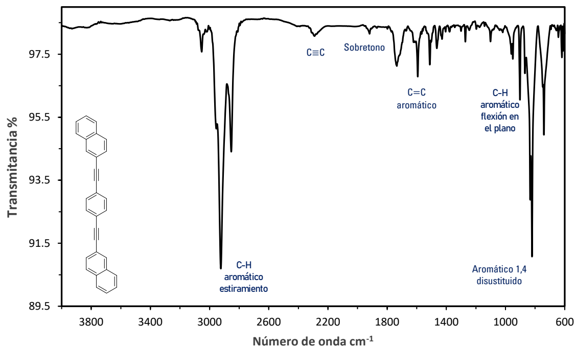
Figura H33. Espectro de infrarrojo del rotor molecular 1,4-bis(naftalen-2-iletinil)benceno (2) en película.
