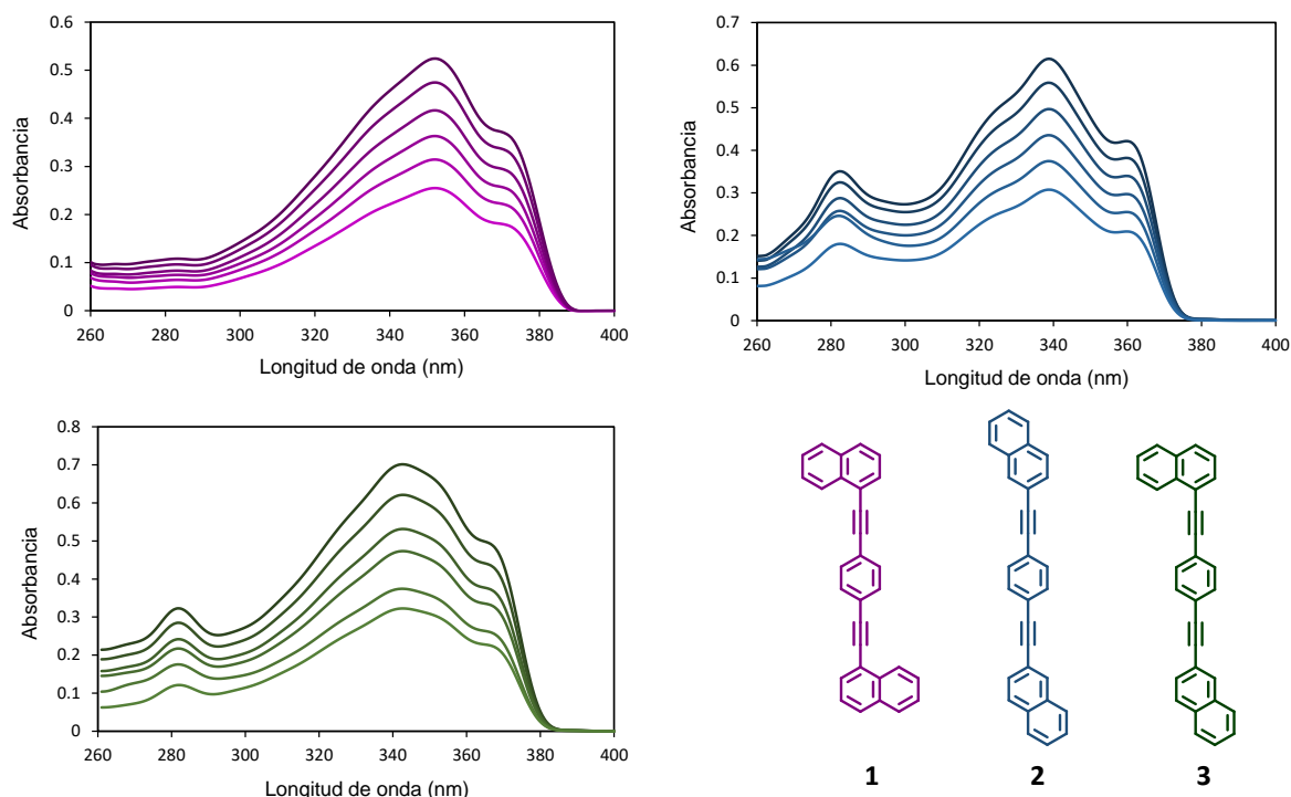
Figura 42. Espectros de absorción de los rotores moleculares 1 , 2 y 3 en THF con concentraciones de 1.16 \times 10^{-5} a 5.82 \times 10^{-6} M, 1.16 \times 10^{-5} a 5.96 \times 10^{-6} M y 1.08 \times 10^{-5} a 5.29 \times 10^{-6} M, respectivamente, utilizados para el cálculo del coeficiente de extinción molar, \epsilon .
