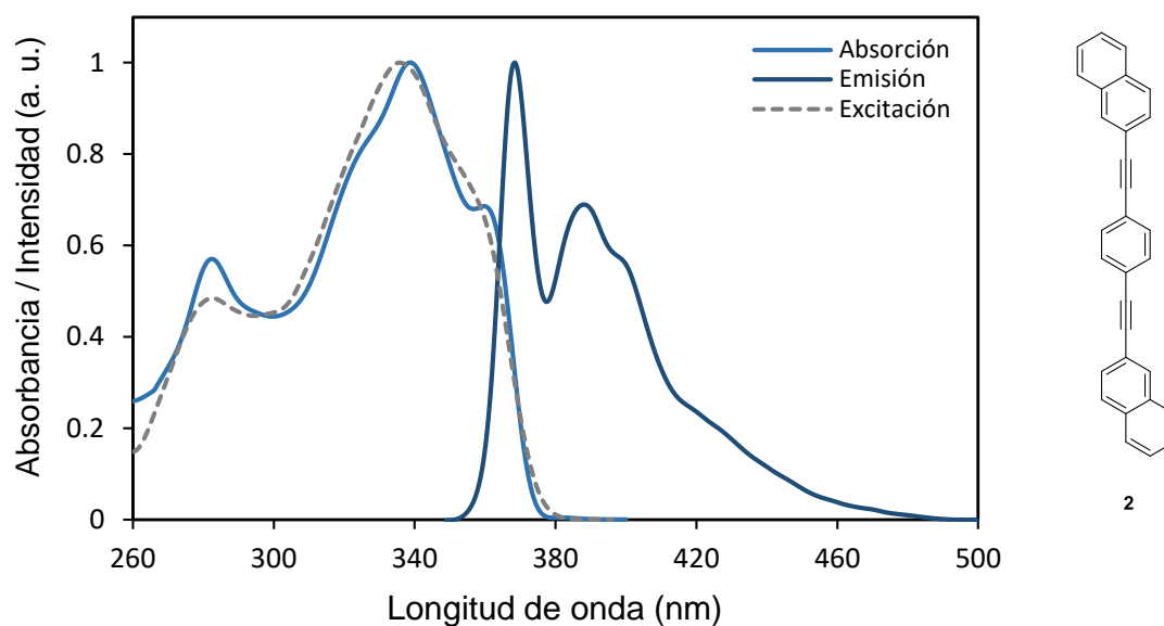
Figura J2. Espectro de absorción, excitación y emisión normalizado del rotor molecular 1,4-bis(naftalen-2-iletinil)benceno ( 2 ) en THF.
