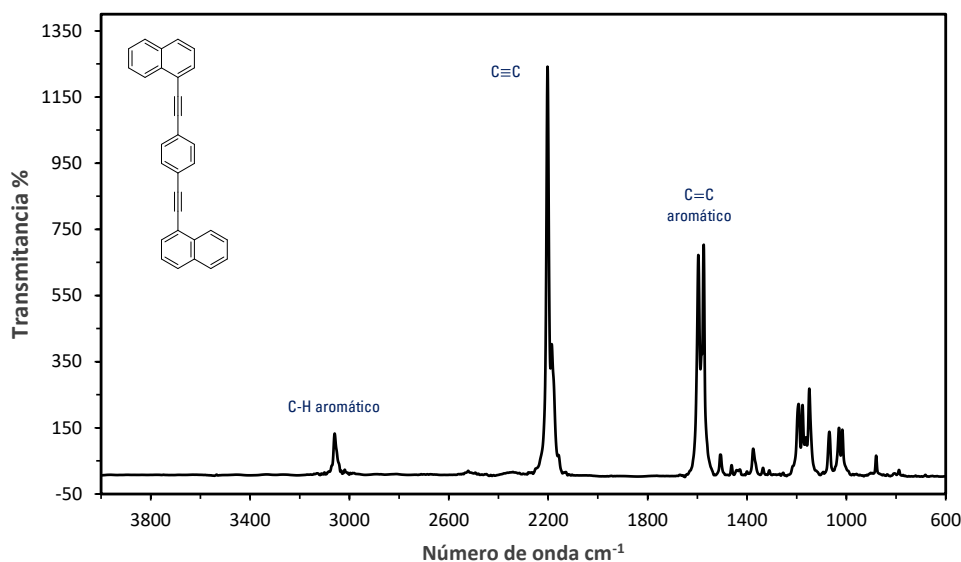
Figura 25. Espectro Raman del rotor molecular 1,4-bis(naftalen-1-iletinil)benceno ( 1 ).
