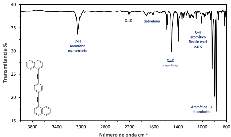
Figura 24. Espectro de infrarrojo del rotor molecular 1,4-bis(naftalen-1-iletinil)benceno ( 1 ) en película.
