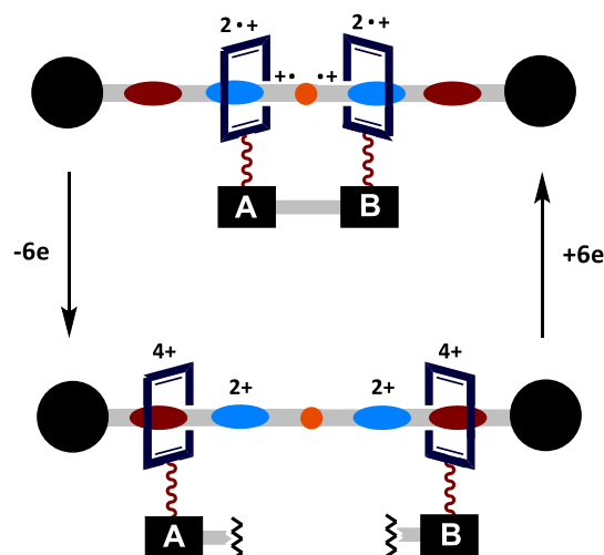
Figura 2. Adición cíclica entre A y B asistida por una máquina molecular compuesta por dos interruptores de rotaxano. Figura adaptada de la referencia 9.
