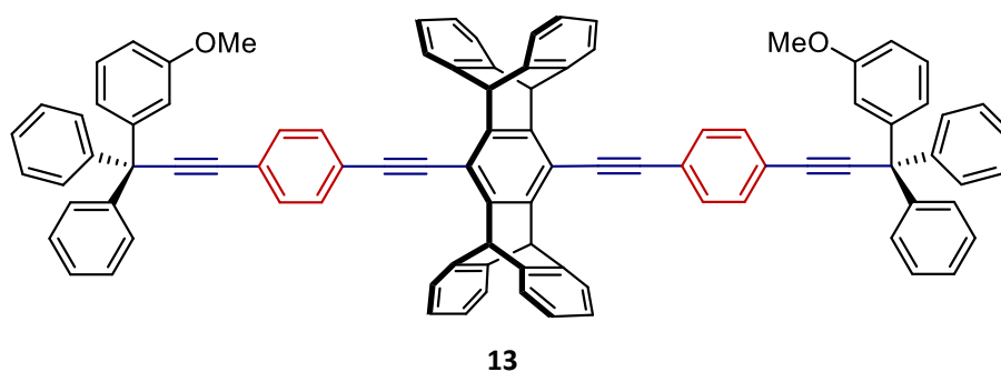
Figura 16. Estructura del dirrotor molecular 6,13-bis({4-[3-(3-metoxifenil)-3,3-difenilprop-1-in-1-il]fenil}etinil)-5,7,12,14-tetrahidro-5,14:7,12-bis([1,2]benceno)pentaceno ( 13 ) sintetizado por Huhgs y col., cuya estructura cuenta con dos fenilenos (rojo) como rotadores y cuatro grupos etinileno (azul) actuando como ejes y conectores de las partes móviles con los estatores (negro). Figura adaptada de la referencia 44.
