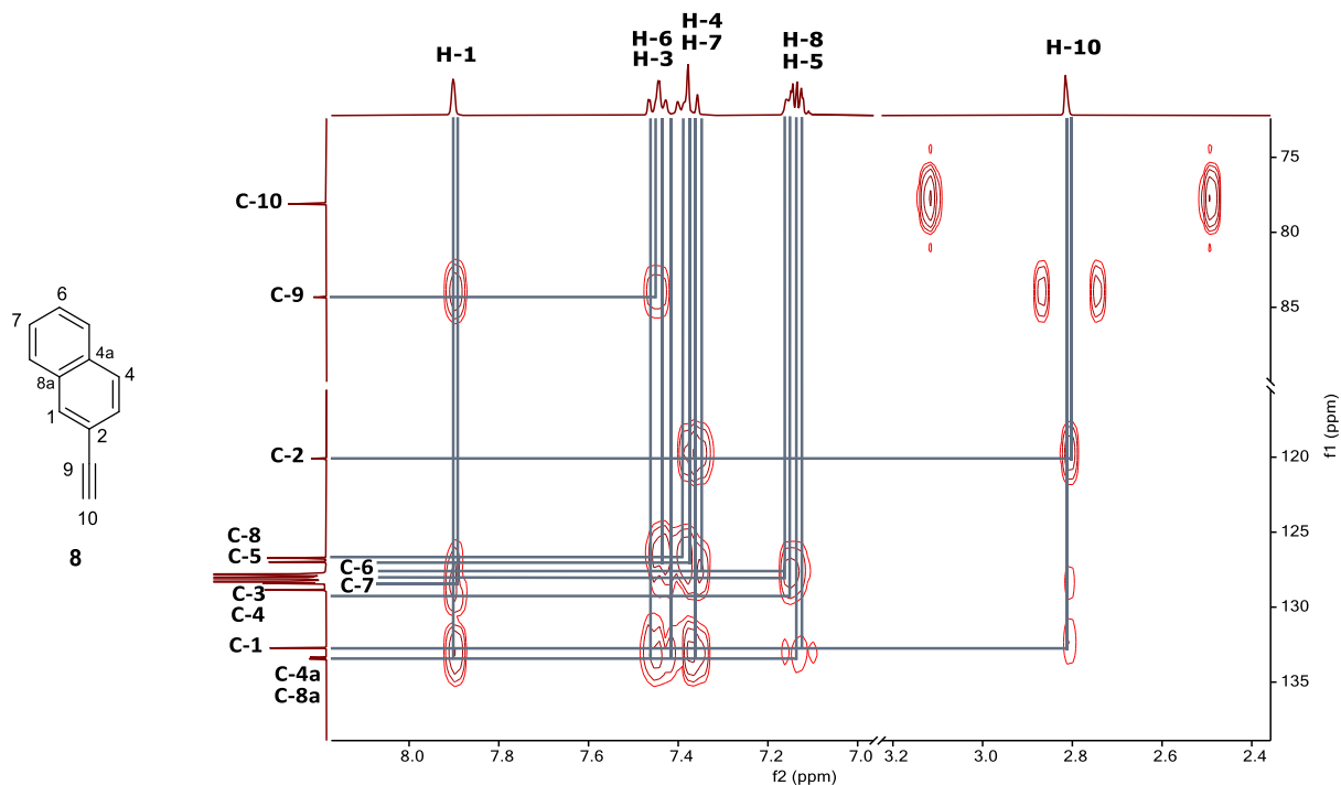
Figura H29. Espectro HMBC del 2-etinilnaftaleno ( 8 ) en C_6D_6 a 25 °C.
