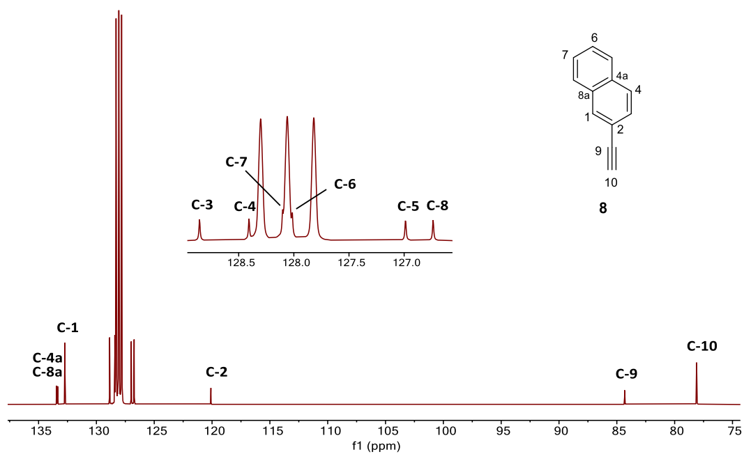
Figura H25. Espectro de RMN de ^{13}\text{C} del 2-etinilnaftaleno ( 8 ) adquirido a 101 MHz en \text{C}_6\text{D}_6 a 25 °C.
