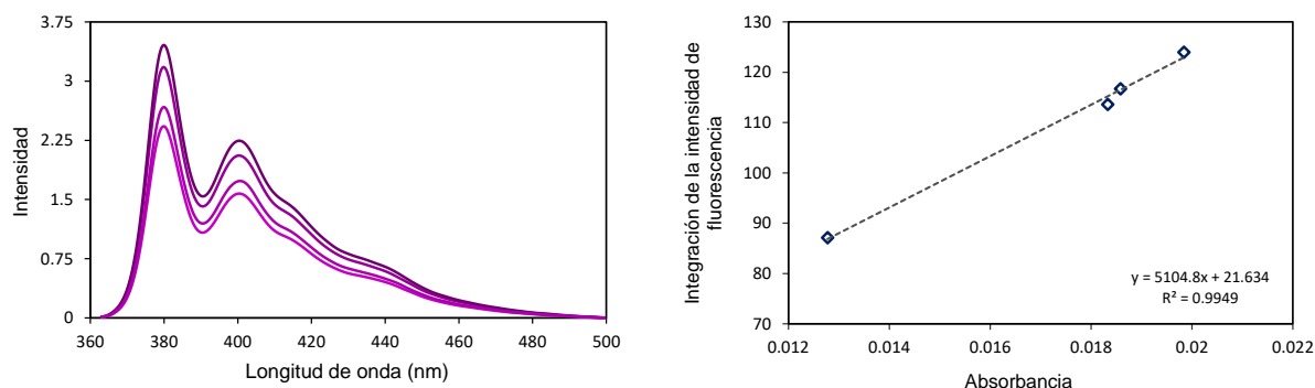
Figura 45. Espectros de emisión (izquierda) y gráfico de la integración de la intensidad de fluorescencia contra la absorbancia medida (derecha), usados para el cálculo del rendimiento cuántico del rotor molecular 1 en THF a temperatura ambiente.
