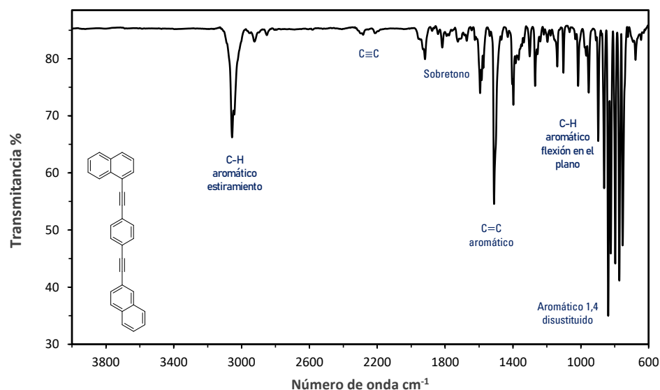
Figura 32. Espectro de infrarrojo del rotor molecular 1-[[4-(naphthalen-2-iletinil)fenil]etinil]naftaleno ( 3 ) en película.
