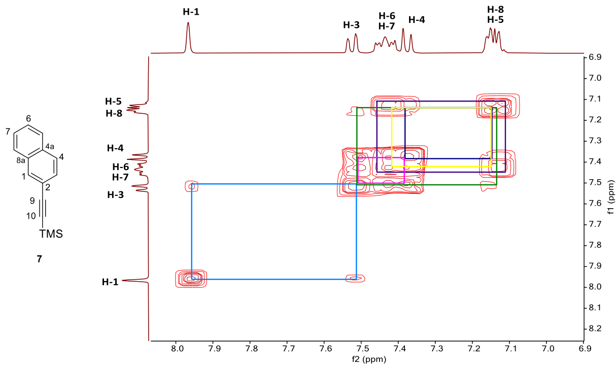
Figura H20. Espectro COSY del 2-(trimetilsilil)etnilnaftaleno ( 7 ) en \text{C}_6\text{D}_6 a 25 °C.
