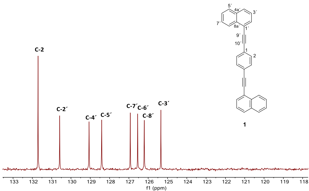
Figura H14. DEPT-135 del rotor molecular 1,4-bis(naftalen-1-iletinil)benzeno ( 1 ) adquirido a 101 MHz en \text{CDCl}_3 a 25^\circ\text{C} .
