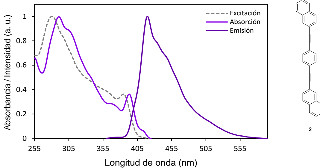
Figura J8. Espectro de absorción, emisión y excitación normalizados del rotor molecular 1,4-bis(naftalen-2-iletinil)benceno ( 2 ) en película.
