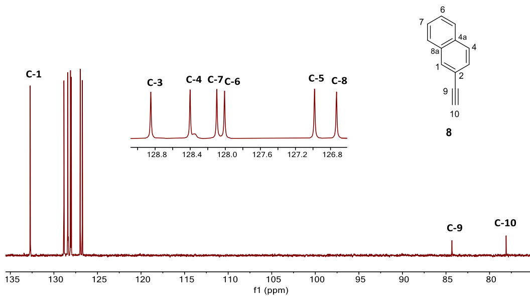
Figura H26. DEPT-135 del 2-etinilnaftaleno ( 8 ) adquirido a 101 MHz en \text{C}_6\text{D}_6 a 25 °C.
