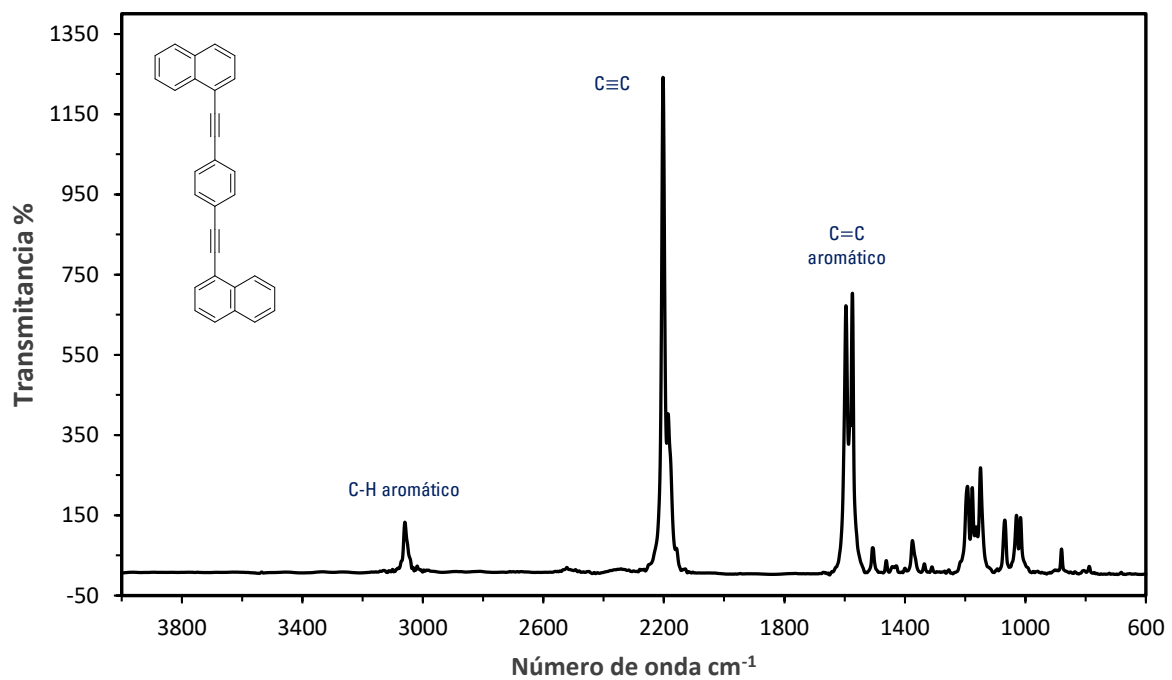
Figura H16. Espectro Raman del rotor molecular 1,4-bis(naftalen-1-iletinil)benceno ( 1 ).
