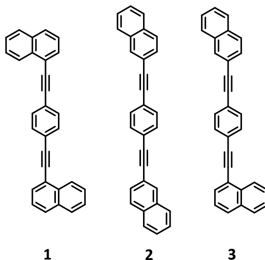
Figura 20. Rotores moleculares 1,4-bis(naftalen-1-iletinil)benceno (1), 1,4-bis(naftalen-2-iletinil)benceno (2) y 1-{[(4-naftalen-2-iletinil)fenil]etinil} (3) sintetizados y presentados en este trabajo de tesis.
