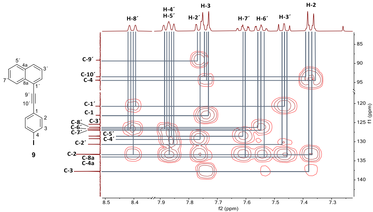
Figura H40. Espectro HMBC del 1-[(4-yodofenil)etnil]naftaleno ( 9 ) en \text{CDCl}_3 a 25 °C.
