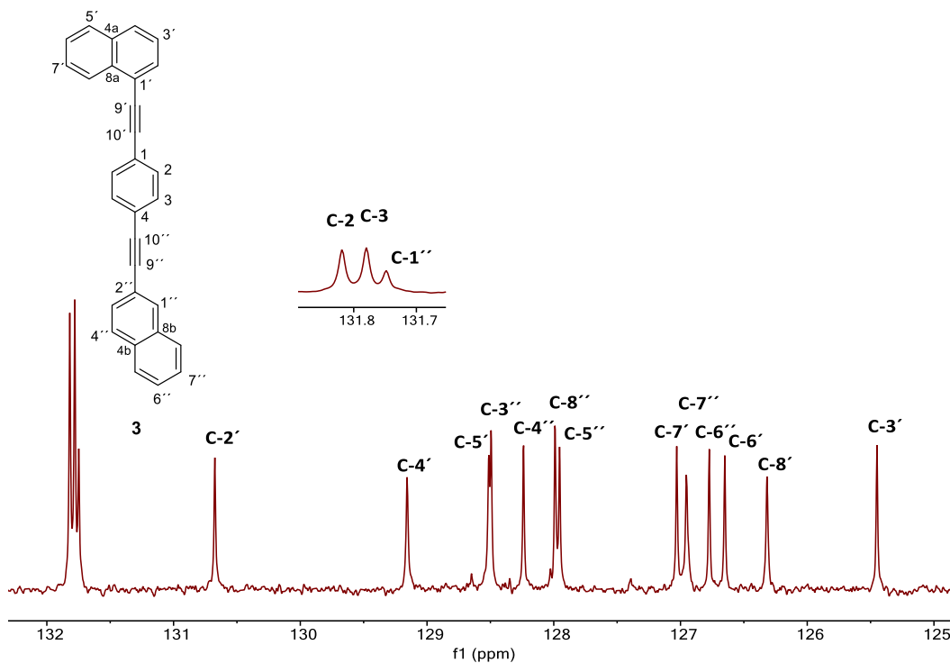
Figura H44. DEPT-135 del rotor molecular 1-[[4-naftalen-2-iletinil]fenil]etinil]naftaleno ( 3 ) adquirido a 101 MHz en \text{CDCl}_3 a 25 °C.
