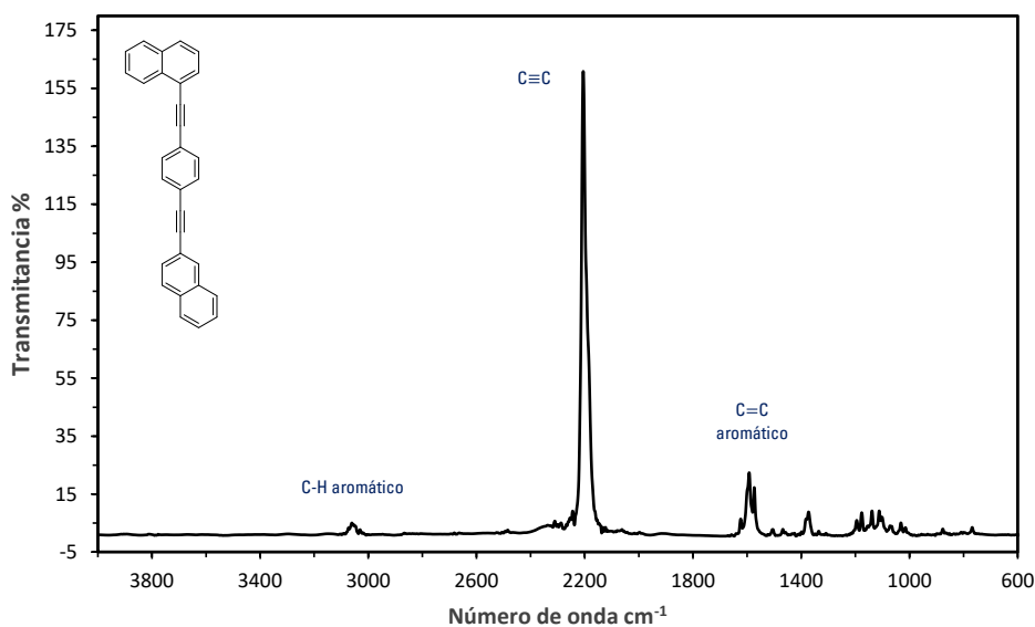
Figura 33. Espectro de Raman del rotor molecular 1-[[4-(naphthalen-2-iletinil)fenil]etinil]naftaleno ( 3 ).
