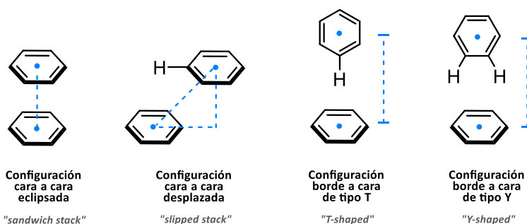
Figura 13. Configuraciones o geometrías que pueden adoptar los anillos aromáticos. Figura adaptada de la referencia 35.
