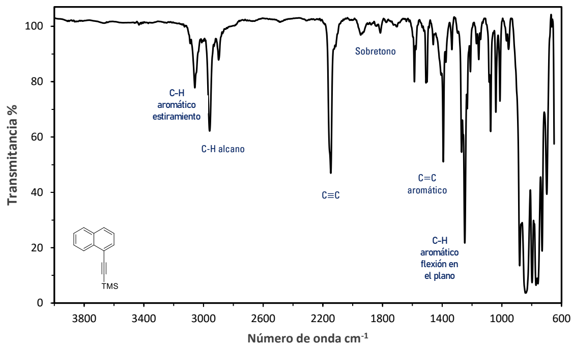
Figura H4. Espectro de infrarrojo del 1-(trimetilsilil)etnilnaftaleno ( 4 ) en película.
