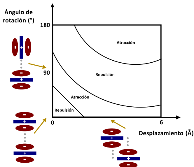
Figura 12. Interacciones electrostáticas entre la distribución de carga \pi como función de su orientación en sistemas aromáticos. Figura adaptada de las referencias 34 y 35.
