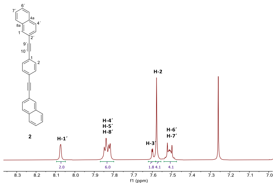
Figura 26. Espectro de RMN de ^1\text{H} del rotor molecular 1,4-bis(naftalen-2-iletinil)benceno ( 2 ) adquirido a 400 MHz en \text{CDCl}_3 a 25 °C.
