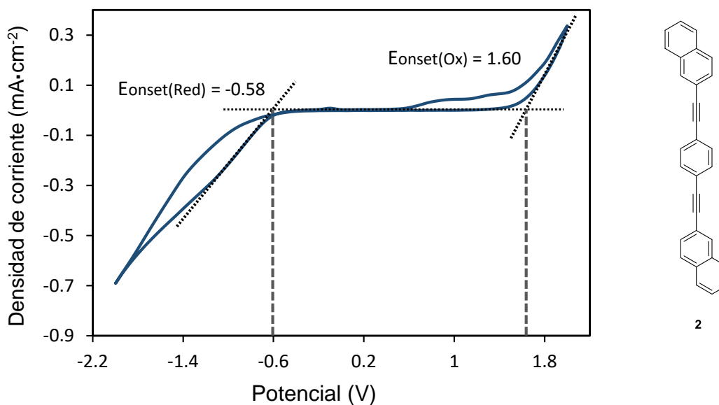
Figura K2. Voltamperograma cíclico del rotor molecular 1,4-bis(naftalen-2-iletinil)benceno ( 2 ) usando un sistema ITO/0.01 M de 2 + 0.1 M de perclorato de tetrabutilamonio en diclorometano anhidro a 20 mV s -1 .
