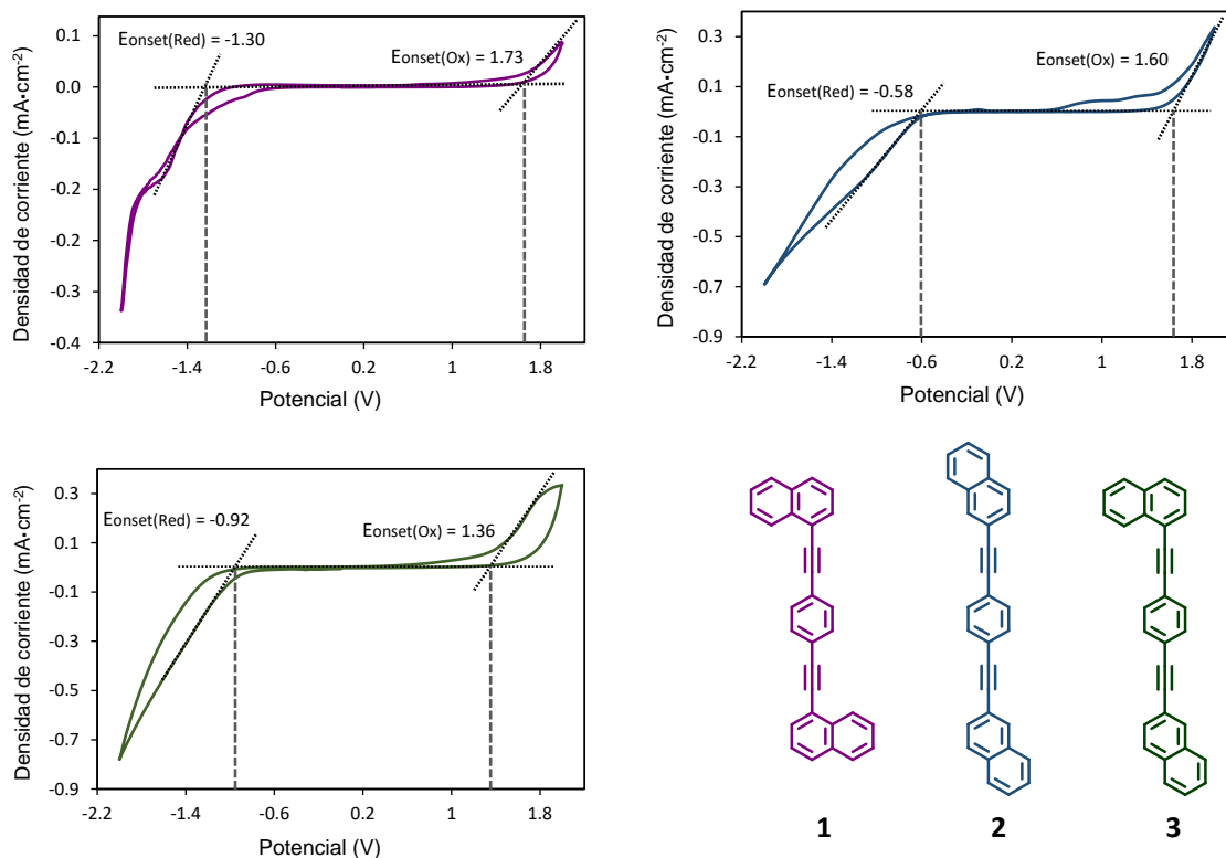
Figura 51. Voltamperograma cíclico de los rotore 1, 2 y 3 usando un sistema ITO/0.01 M de cada rotor + 0.1 M de perclorato de tetrabutilamonio en diclorometano anhidro a 20 mV s -1 .
