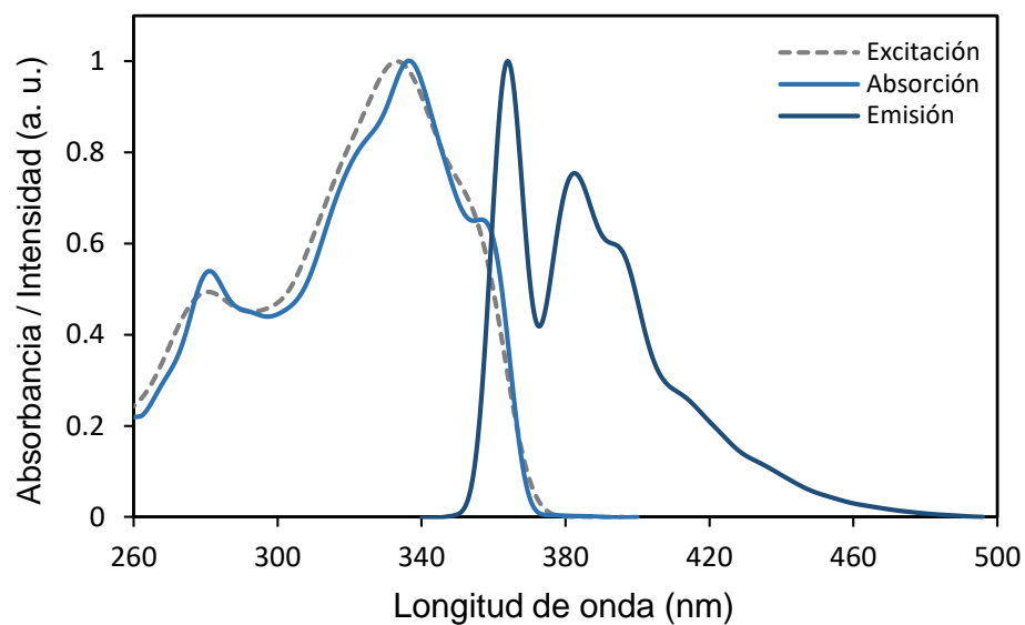
Figura J5. Espectro de excitación y emisión normalizado del rotor molecular 1,4-bis(2-naftalen-2-iletinil)benceno ( 2 ) en n -hexano.
