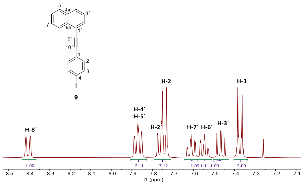
Figura H35. Espectro de RMN de ^1\text{H} del 1-[(4-yodofenil)etnil]naftaleno ( 9 ) adquirido a 400 MHz en \text{CDCl}_3 a 25 °C.
