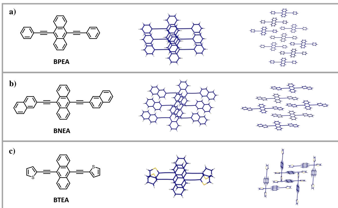
Figura 15. Estructura química y apilamiento de los cristales a) BPEA , b) BNEA y c) BTEA sintetizados por el grupo de Wang para fabricar transistores. Figura adaptada de la referencia 43.
