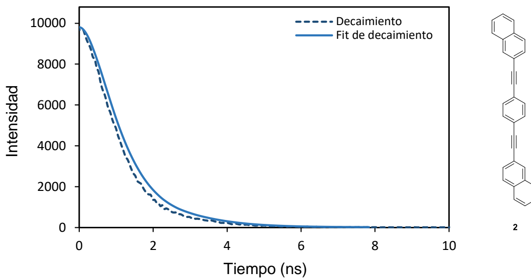
Figura J11. Curva de decaimiento de fluorescencia experimental y ajuste exponencial para el rotor molecular 1,4-bis(naftalen-2-iletinil)benzeno ( 2 ).
