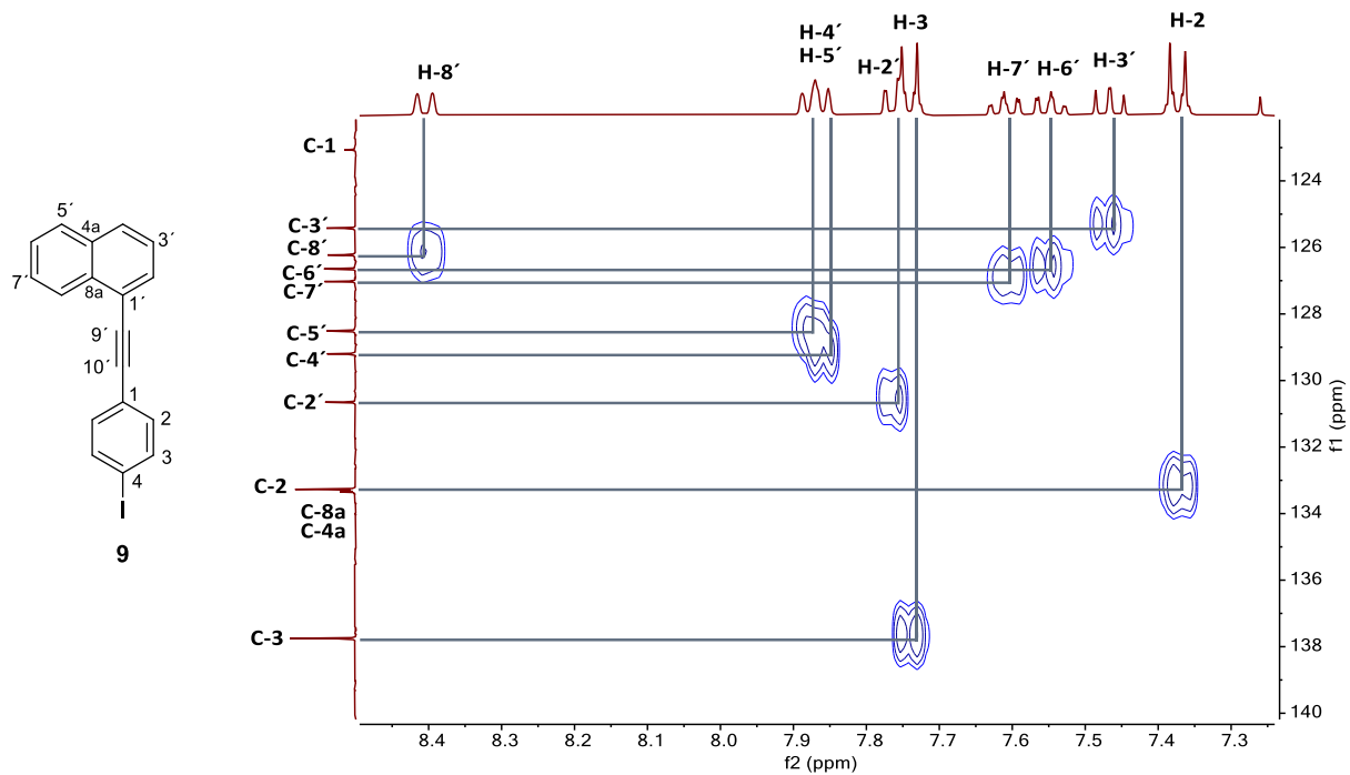
Figura H39. Espectro HSQC del 1-[(4-yodofenil)etnil]naftaleno ( 9 ) en \text{CDCl}_3 a 25 °C.
