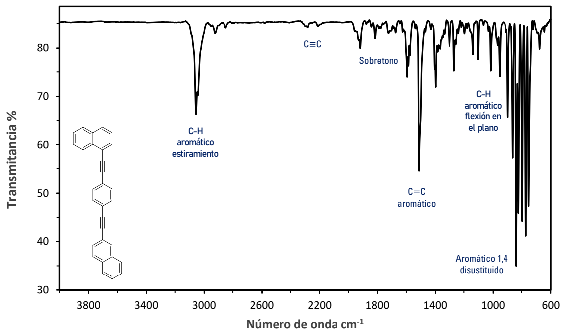
Figura H45. Espectro de infrarrojo del rotor molecular 1-[(4-naftalen-2-iletinil)fenil]etinil}naftaleno ( 3 ) en película.
