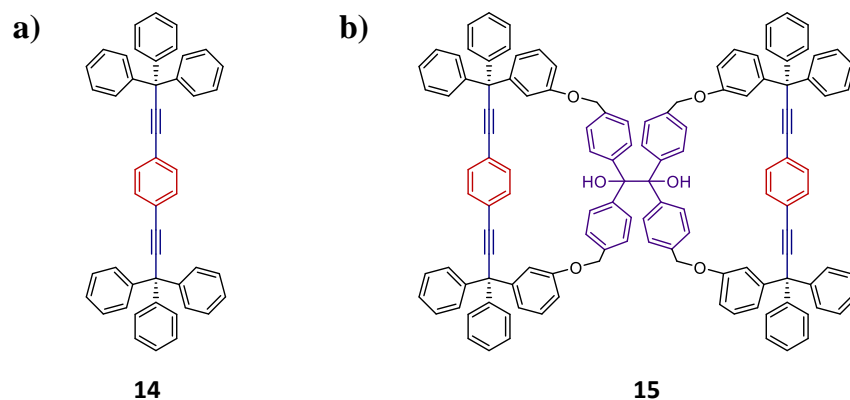
Figura 18. a) Rotor molecular 14 sintetizado por Howe y col., cuya estructura cuenta con un fenileno (rojo) como rotador, dos grupos etinilo (azul) actuando como ejes y los grupos trifenilmetil como estatores; b) Dirrotor
