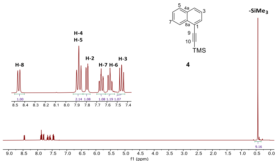
Figura H1. Espectro de RMN de ^1\text{H} del 1-(trimetilsilil)etnilnaftaleno ( 4 ) adquirido a 400 MHz en \text{CDCl}_3 a 25^\circ\text{C} .
