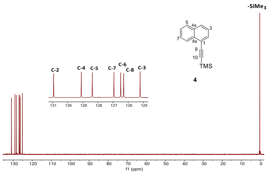
Figura H3. DEPT-135 del 1-(trimetilsilil)etnilnaftaleno ( 4 ) adquirido a 101 MHz en \text{CDCl}_3 a 25 °C.
