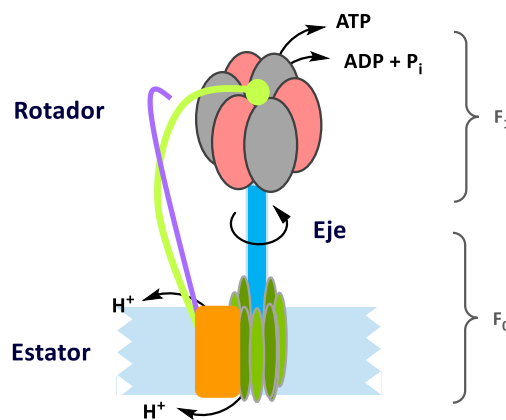
Figura 1. Motor rotatorio de ATP sintasa ( Archetypal F 1 F 0 ) como ejemplo de una máquina molecular biológica de transmembrana. Figura adaptada de la referencia 5.
