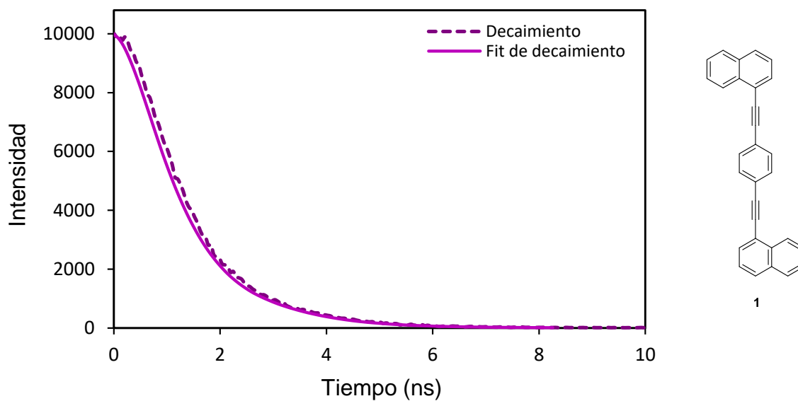
Figura J10. Curva de decaimiento de fluorescencia experimental y ajuste exponencial para el rotor molecular 1,4-bis(naftalen-1-iletinil)benceno ( 1 ).
