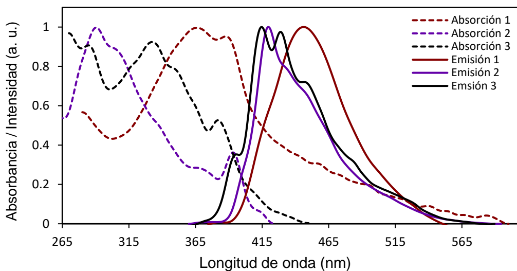
Figura 50. Comparación de los espectros de absorción (línea punteada) y emisión (línea sólida) normalizados de los rotores 1 , 2 y 3 en película.
