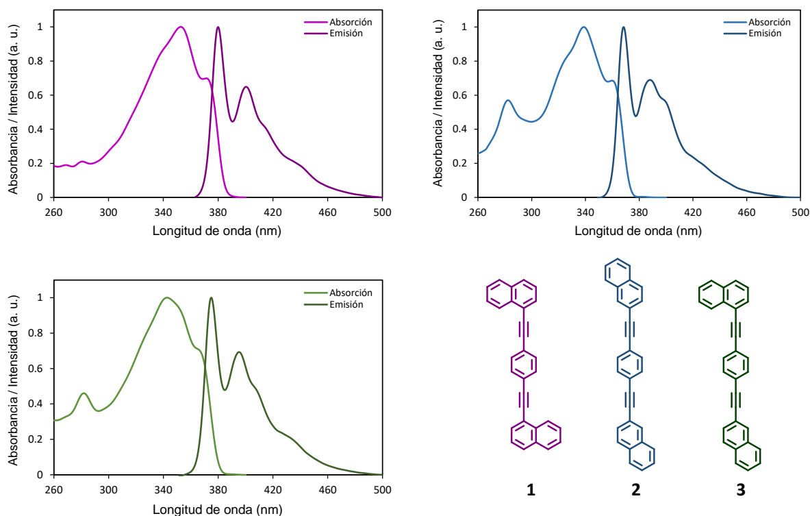
Figura 41. Espectros de absorción y emisión de los rotores moleculares 1 , 2 y 3 en THF a temperatura ambiente.
