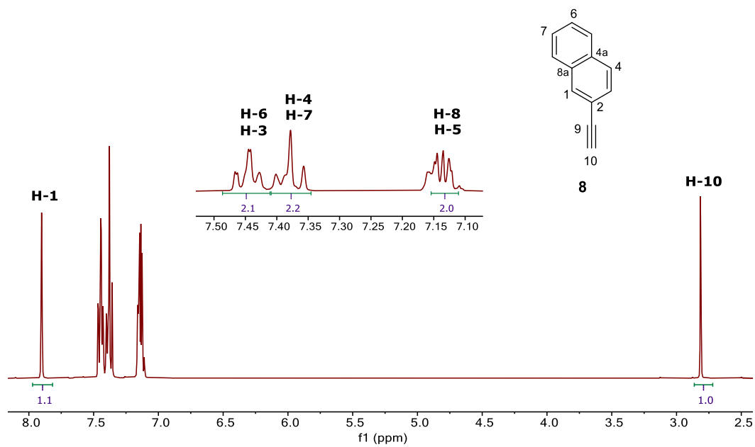
Figura H24. Espectro de RMN de ^1\text{H} del 2-etnilnaftaleno ( 8 ) adquirido a 400 MHz en \text{C}_6\text{D}_6 a 25 °C.
