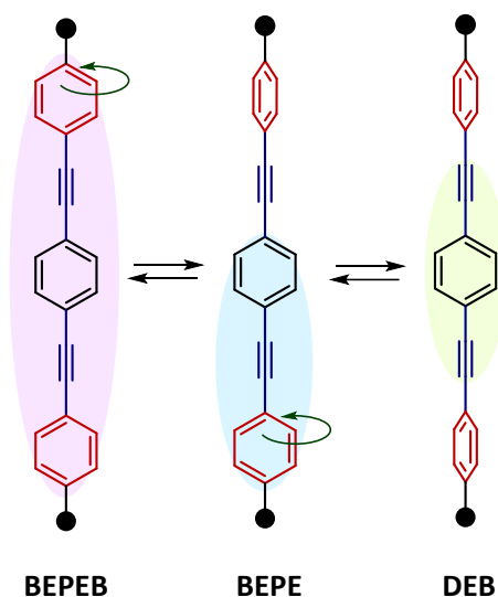
Figura 17. Grado de extensión de la conjugación \pi de los cromóforos 1,4-bis[(4-etinilfenil)etnil]benceno ( BEPEB ) (sombreado en morado), 1,2-bis(4-etinilfenil)-etino ( BEPE ) (sombreado en azul) y 1,4-dietinil benceno ( DEB ) (sombreado en verde) dependiente de la torsión de los grupos fenileno. Ciertos elementos o grupos de cada molécula de los rotores fueron omitidos para un mejor entendimiento de la conjugación del sistema. Figura adaptada de la referencia 44.
