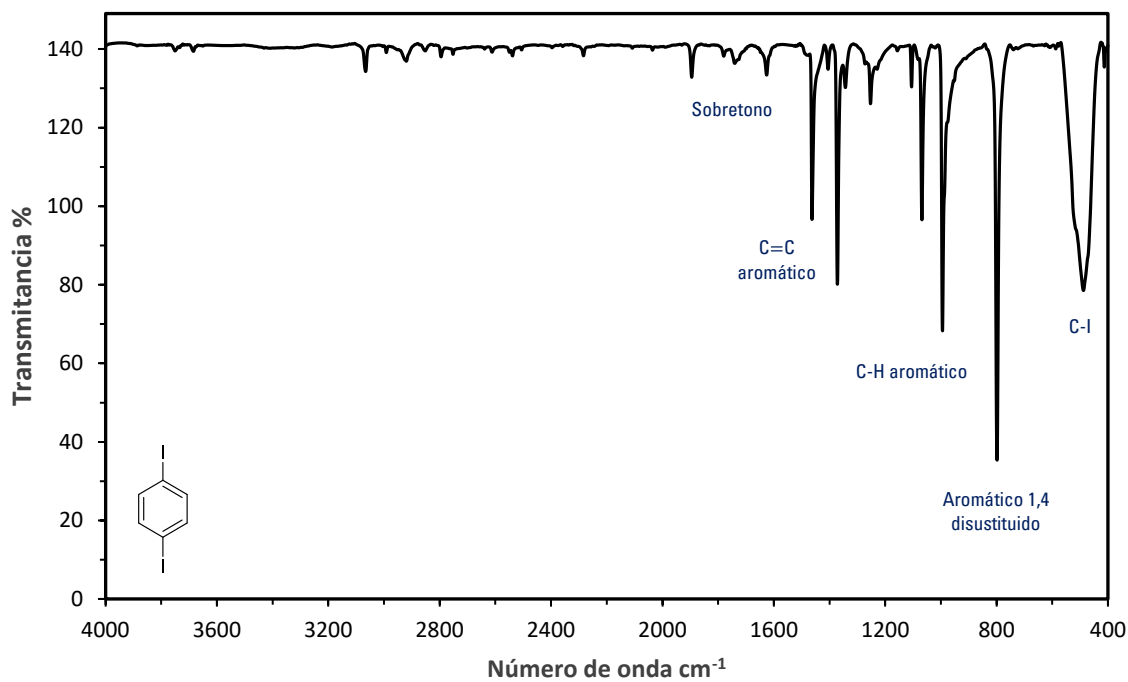
Figura H11. Espectro de infrarrojo del 1,4-diyodobenceno ( 6 ) en película.
