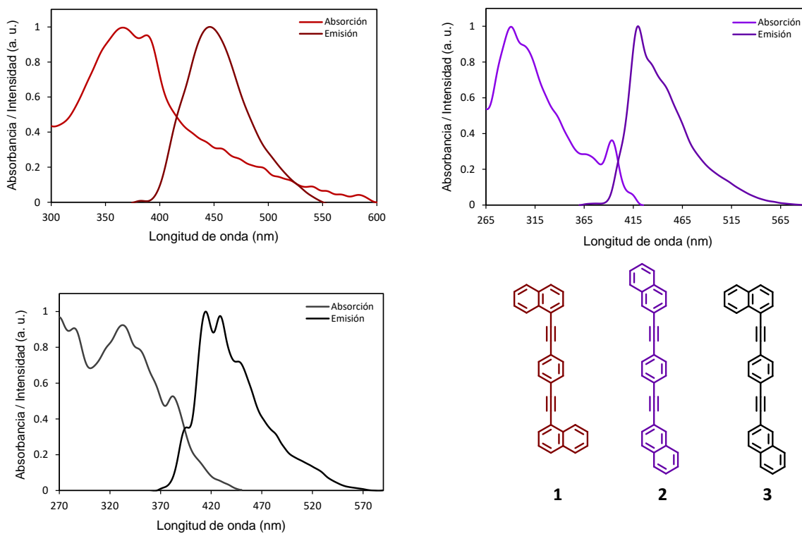
Figura 49. Espectros de absorción y emisión de los rotores moleculares 1 , 2 y 3 en película a temperatura ambiente.
