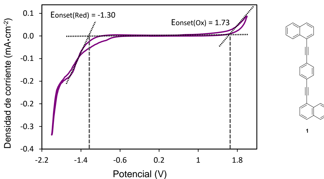
Figura K1. Voltamperograma cíclico del rotor molecular 1,4-bis(naftalen-1-iletinil)benceno ( 1 ) usando un sistema ITO/0.01 M de 1 + 0.1 M de perclorato de tetrabutilamonio en diclorometano anhidro a 20 mV s -1 .
