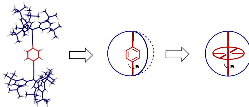
Figura 9. Comparación analógica entre un giroscopio molecular reportado por Khuong y col. y un giroscopio macroscópico. Figura adaptada de la referencia 31.
