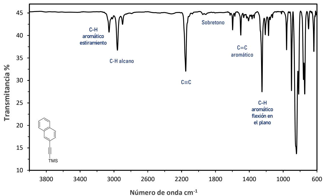
Figura H23. Espectro de infrarrojo del 2-(trimetilsilil)etnilnaftaleno ( 7 ) en película.
