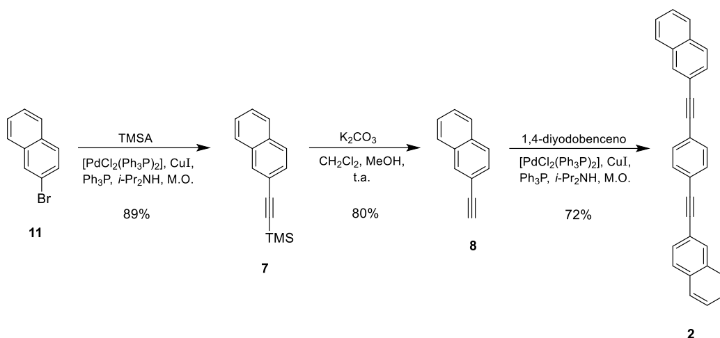
Esquema 4. Síntesis del rotor molecular 1,4-bis(naftalen-2-iletinil)benceno ( 2 ).
