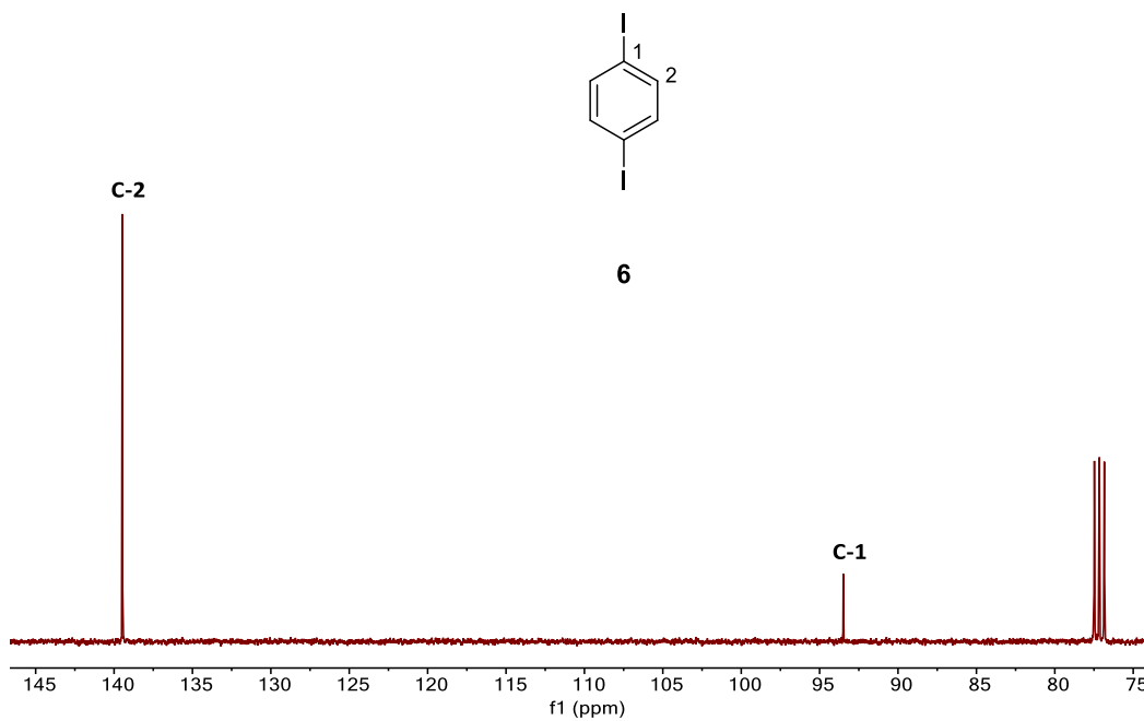
Figura H10. Espectro de RMN de 13 C del 1,4-diyodobenceno ( 6 ) adquirido a 101 MHz en CDCl 3 a 25 °C.
