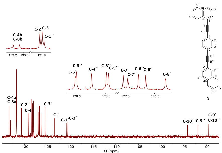
Figura 31. Espectro de RMN de ^{13}\text{C} del rotor molecular 1-[[4-naftalen-2-iletinil]fenil]etinil}naftaleno ( 3 ) adquirido a 101 MHz en \text{CDCl}_3 a 25 °C.
