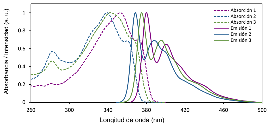
Figura 43. Comparación de los espectros de absorción (línea punteada) y emisión (línea sólida) normalizados de los rotores 1 , 2 y 3 en THF.
