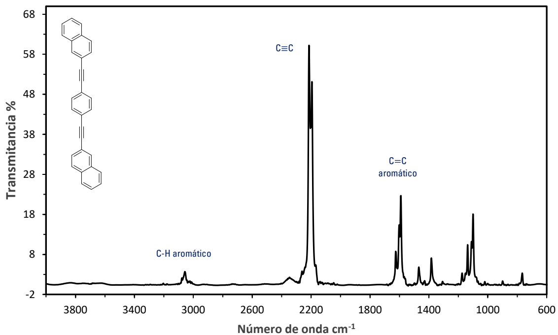
Figura H34. Espectro Raman del rotor molecular 1,4-bis(naftalen-2-iletinil)benceno (2).
