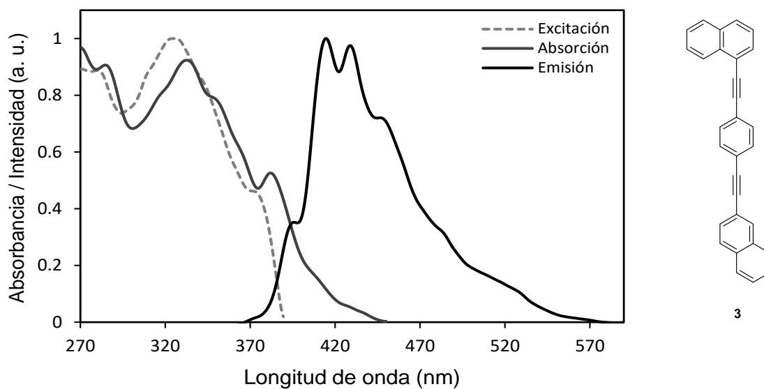
Figura J9. Espectro de absorción, emisión y excitación normalizados del rotor molecular 1-[(4-naftalen-2-iletinil)fenil]etnil}naftaleno ( 3 ) en película.
