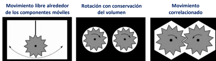
Figura 7. Representación de los requerimientos generales para la obtención de dinámica dentro de ambientes rígidos o en medios con alta densidad. Figura adaptada de la referencia 26.
