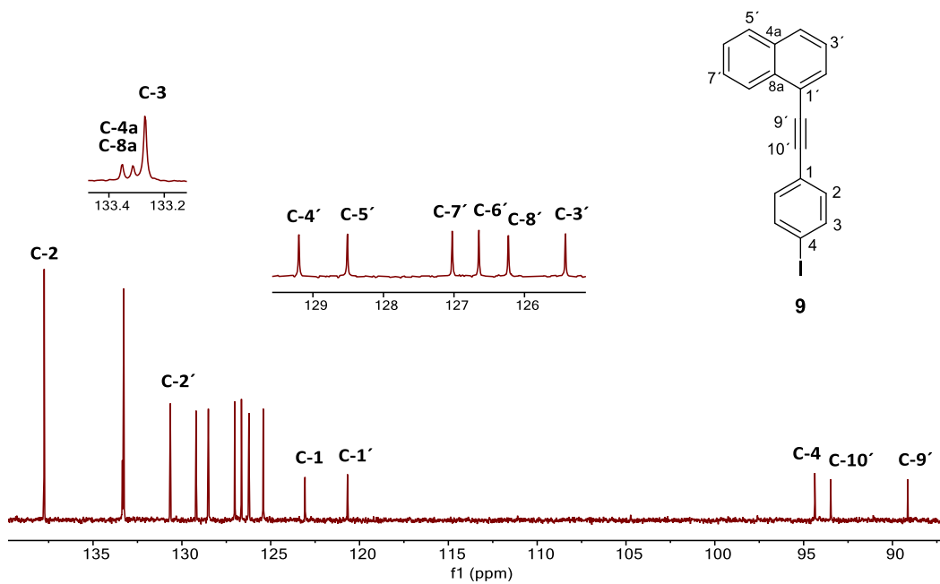
Figura H36. Espectro de RMN de ^{13}\text{C} del 1-[(4-yodofenil)etnil]naftaleno ( 9 ) adquirido a 101 MHz en \text{CDCl}_3 a 25 °C.
