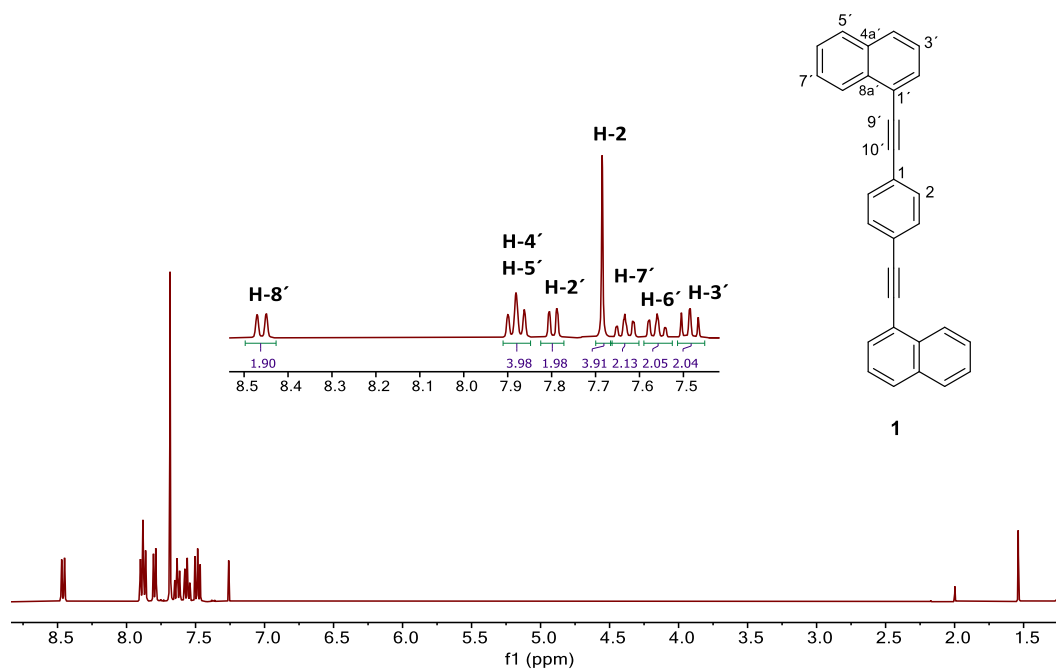
Figura H12. Espectro de RMN de ^1\text{H} del rotor molecular 1,4-bis(naftalen-1-iletinil)benceno ( 1 ) adquirido a 400 MHz en \text{CDCl}_3 a 25 °C.
