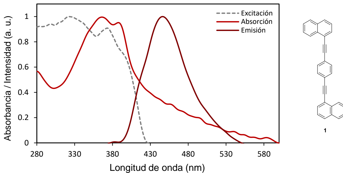
Figura J7. Espectro de absorción, excitación y emisión normalizados del rotor molecular 1,4-bis(naftalen-1-iletinil)benceno ( 1 ) en película.
