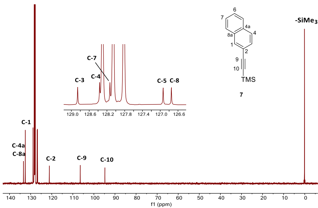
Figura H18. Espectro de RMN de ^{13}\text{C} del 2-(trimetilsilil)etininftaleno ( 7 ) adquirido a 101 MHz en \text{C}_6\text{D}_6 a 25^\circ\text{C} .
