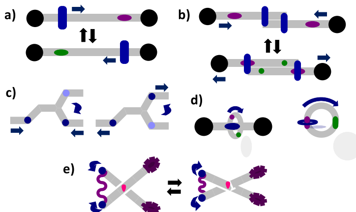
Figura 4. Principales interruptores moleculares clasificados según su tipo de movimiento y modo de operación: a) Lanzaderas (ej. rotaxanos); b) Expansión/contracción (ej. músculos moleculares); c) Agitadores (ej. azobencenos); d) Rotadores (ej. rotores moleculares); e) “Movimiento tipo tijera” (ej. enzimas de restricción o tijeras moleculares). Figura adaptada de la referencia 9.
