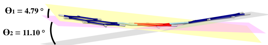
Figura 39. Estructura molecular del rotor 3 y b) ángulo interplanar generado por la intersección de los planos de los estatores (amarillo y gris) con respecto al plano del anillo de fenileno (violeta).
