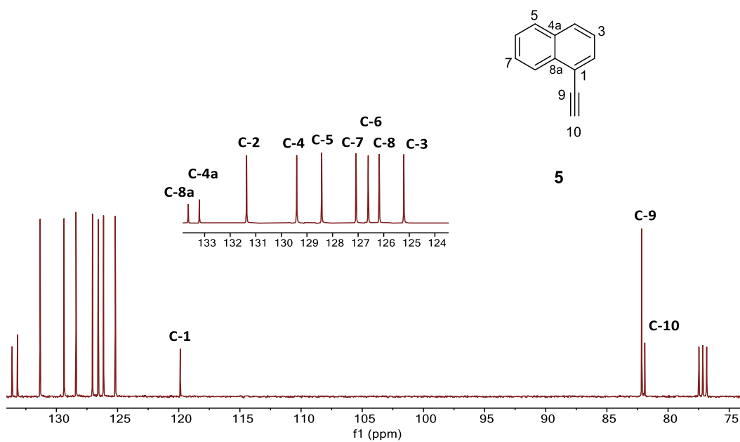
Figura H6. Espectro de RMN de ^{13}\text{C} del 1-etinilnaftaleno ( 5 ) adquirido a 101 MHz en \text{CDCl}_3 a 25 ^\circ\text{C} .
