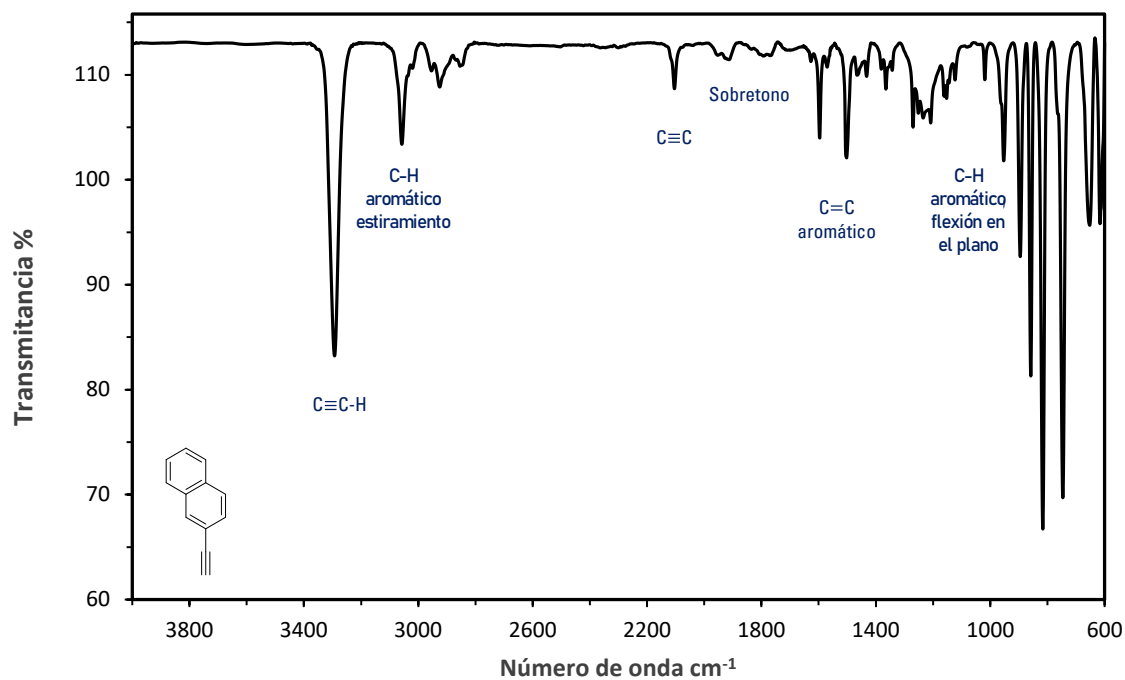
Figura H30. Espectro de infrarrojo del 2-etinilnaftaleno ( 8 ) en película.
