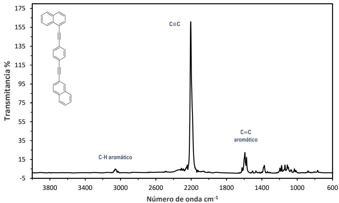
Figura H46. Espectro Raman del rotor molecular 1-[(4-naftalen-2-iletinil)fenil]etinil}naftaleno ( 3 ).
