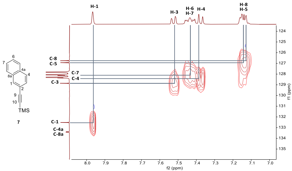
Figura H21. Espectro HSQC del 2-(trimetilsilil)etnilnaftaleno ( 7 ) en C_6D_6 a 25 °C.
