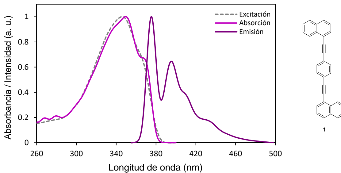
Figura J4. Espectro de excitación y emisión normalizado del rotor molecular 1,4-bis(naftalen-1-iletinil)benceno ( 1 ) en n -hexano.
