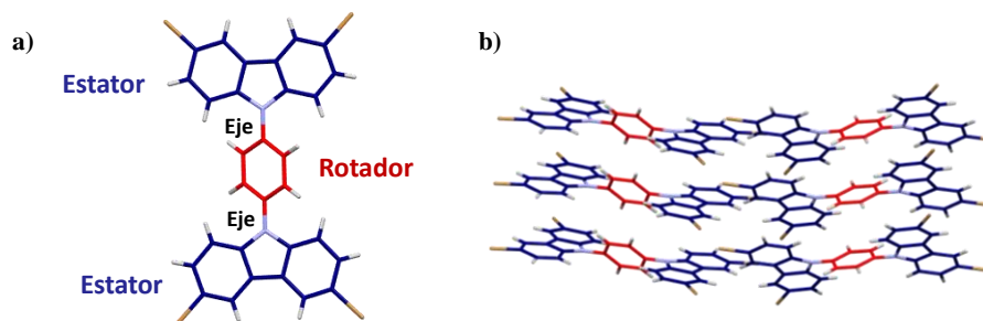
Figura 6. a) Partes señaladas de un rotor molecular sintetizado y reportado por Colín-Molina y col. b) en el que aprecia el empaquetamiento de mismos para formar un cristal anfidinámico. La parte móvil de cada rotor se encuentra resaltada en rojo y la parte estática en azul. Figura adaptada de la referencia 28.
