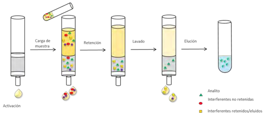
Figura 19. Diagrama del proceso de limpieza de muestras mediante cartucho de SPE.
