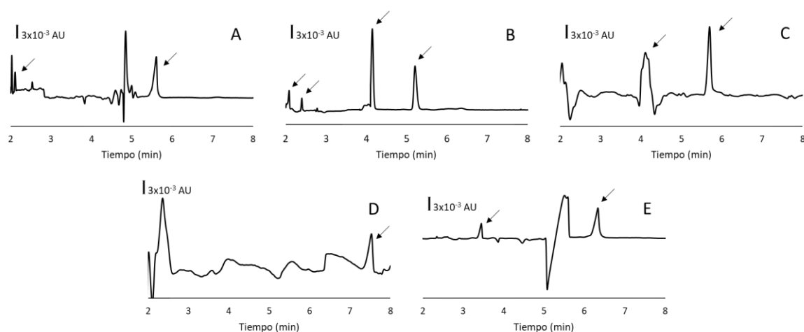
Figura 11. Electroferogramas correspondientes a la evaluación de pH. A) ES de fosfatos pH=8, B) ES de boratos pH=9, C) ES de boratos pH=10, D) ES fosfatos pH=11, E) ES de fosfatos pH=12. 18 KV, \lambda=215 nm.
