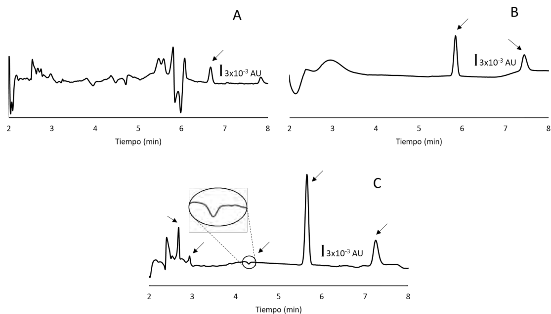
Figura 12. Electroferogramas obtenidos mediante el uso de ES de \text{Na}_2\text{B}_4\text{O}_7 25 \text{mmol L}^{-1} ajustados pH 9.0, a \lambda=215 nm y 18 kV. A) biftalato de potasio 5 \text{mmol L}^{-1} , B) ácido pícrico 5 \text{mmol L}^{-1} y C) benzoato de sodio 5 \text{mmol L}^{-1} .
