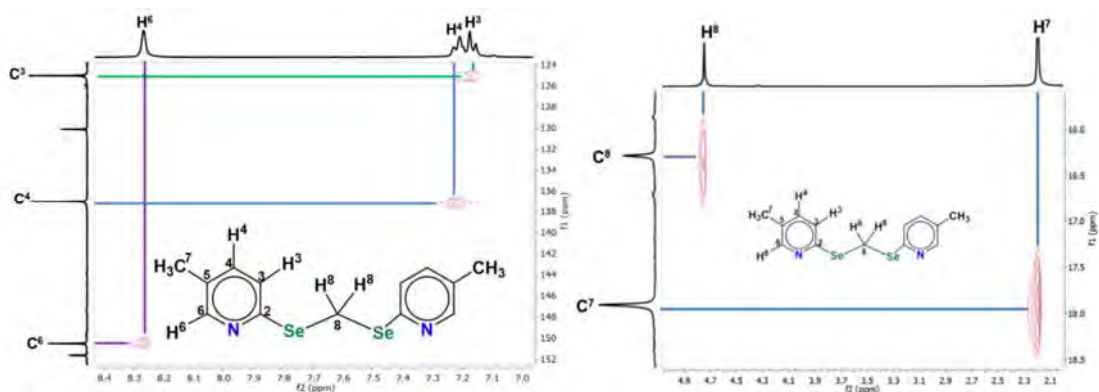
Figura 3.31 Espectro gHSQCAD del compuesto DML5 en \text{CDCl}_3 a 25 °C.
