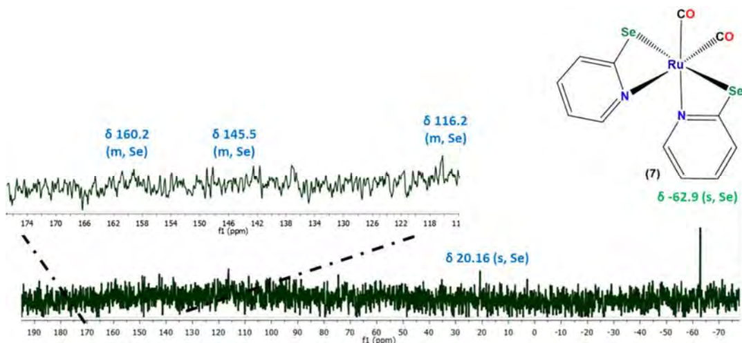
Figura 4.8. Espectro de RMN de ^{77}\text{Se}\{^1\text{H}\} de la mezcla de reacción en \text{CDCl}_3 a 25\text{ }^\circ\text{C} .
