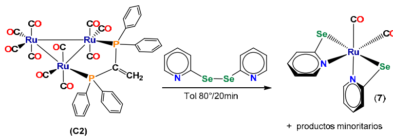
Esquema 4.4. Reacción de (C1) con el 2,2'-dipiridildiselenuro (DL3) en condiciones drásticas de reacción.
