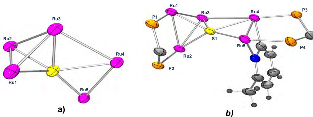
Figura 2.10. a) Geometría BPT distorsionada alrededor del átomo de azufre o bipirámide pentagonal disminuida en dos centros metálicos en términos de la nuclearidad del cúmulo; b) Esqueleto del compuesto 3a.
