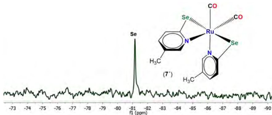
Figura 4.15. Espectro de RMN de 77 Se{ 1 H} del complejo [Ru(pySe) 2 (CO) 2 ] (7), en CDCl 3 a 25 °C.
