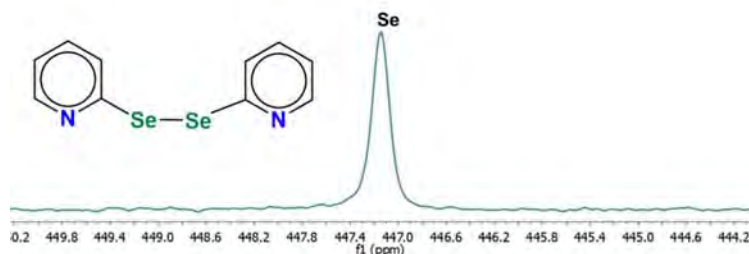
Figura 3.6. Espectro de RMN de ^{77}\text{Se}\{^1\text{H}\} del compuesto DL3 en \text{CDCl}_3 a 25 °C.
