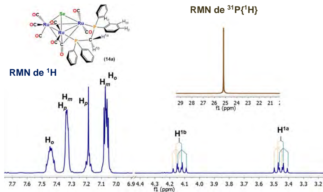
Figura 4.30. Espectros de RMN de ^1\text{H} y ^{31}\text{P}\{^1\text{H}\} del compuesto 14a . en CDCl 3 a 25 °C.
