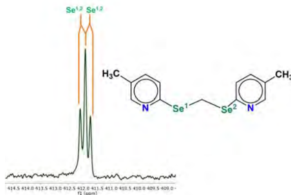
Figura 3.32. Espectro de RMN de ^{77}\text{Se}\{^1\text{H}\} del compuesto DML5 en \text{CDCl}_3 a 25 °C.
