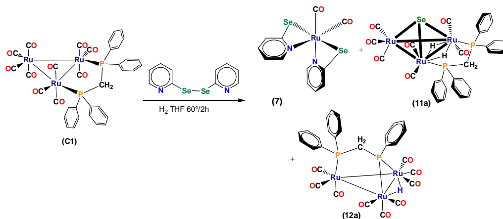
Esquema 4.5. Hidrogenación del cúmulo C1 con el ligante DL3 .
