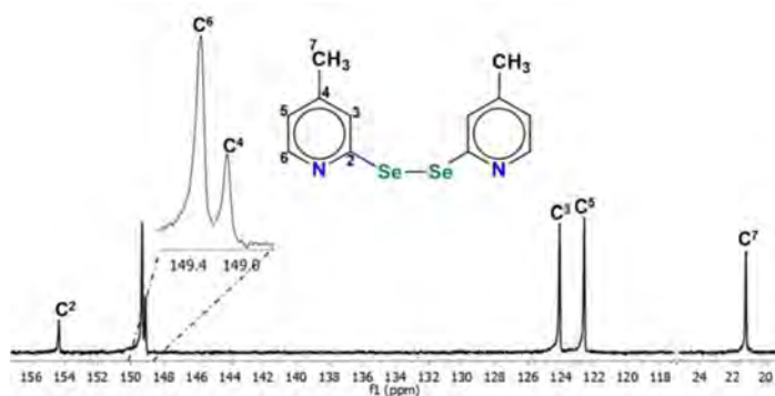
Figura 3.9. Espectro de RMN de ^{13}\text{C}\{^1\text{H}\} del compuesto DL4 en \text{CDCl}_3 a 25^\circ\text{C} .
