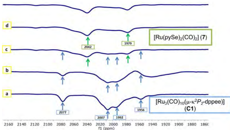
Figura 4.5. Espectro de infrarrojo en la zona de carbonilos terminales de la reacción del C1 y el ligante LNa3 al inicio de la reacción a) , 15 min. b) , 45min. c) y 60 min d) .
