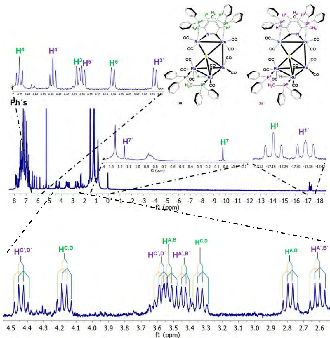
Figura 2.3. Espectro de RMN de ^1\text{H} de los compuestos isoméricos 3a y 3a' en \text{CDCl}_3 a 25^\circ\text{C} .
