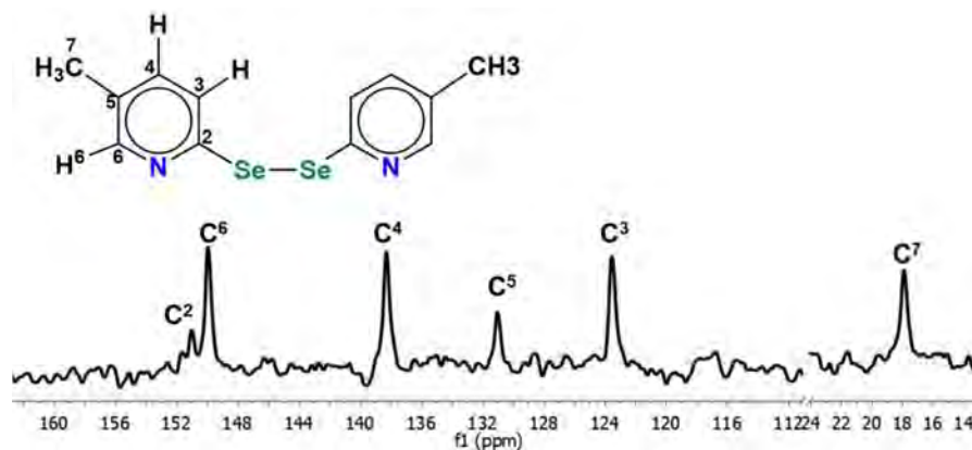
Figura 3.16. Espectro de RMN de ^{13}\text{C}\{^1\text{H}\} del compuesto DL5 .
