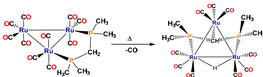
Esquema 1.13. Reacción para la síntesis del compuesto [\text{Ru}_3(\text{CO})_9\{\mu_3\text{-}\kappa^3\text{-P}_2\text{-C-P}(\text{CH}_3)_2\text{PCHP}(\text{CH}_3)_2\}] .
