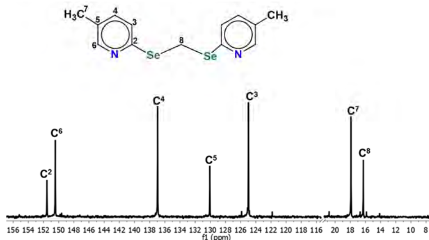
Figura 3.30 Espectro de RMN de ^{13}\text{C}\{^1\text{H}\} del compuesto DML5 en \text{CDCl}_3 a 25 °C.
