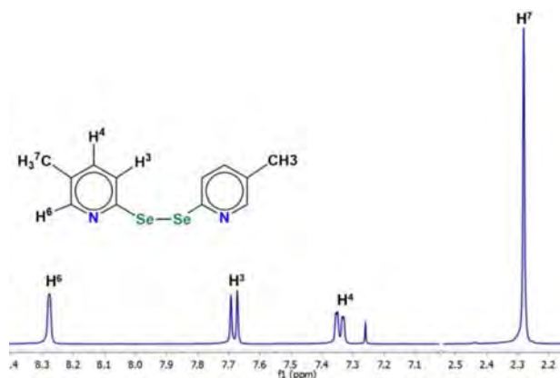
Figura 3.14. Espectro de RMN de ^1\text{H} del compuesto DL5.
