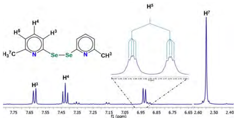
Figura 3.20. Espectro de RMN de ^1\text{H} del compuesto DL6 en \text{CDCl}_3 a 25 °C.
