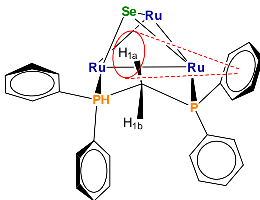
Figura 4.31. Efecto anisotrópico en el compuesto 14a .
