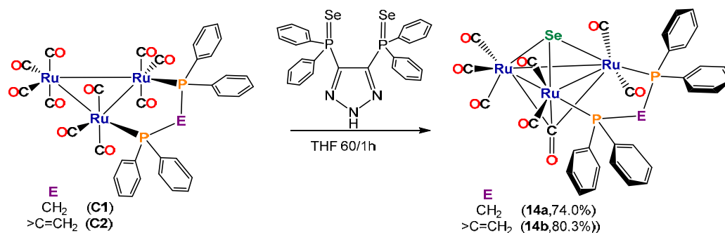
Esquema 4.9. Reactividad del cúmulo C1 y C2 frente al ligante bis(selenodifenilfosfinoil)-1,2,3-triazol (L7) .
