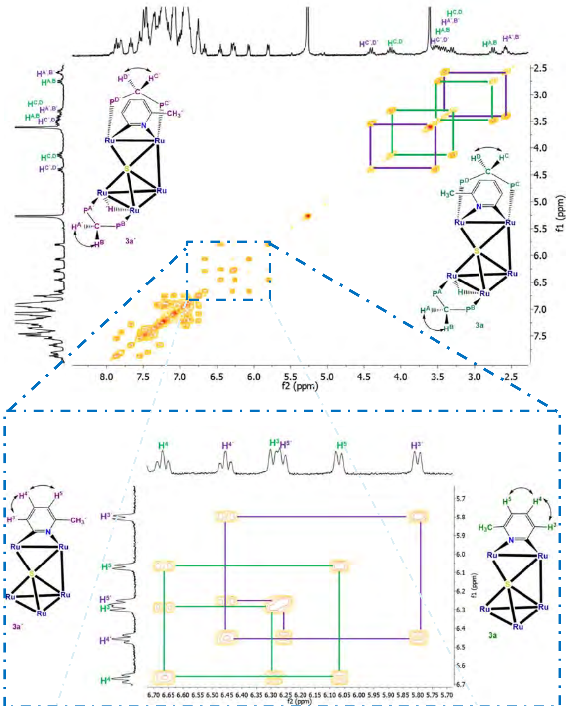
Figura 2.7. Espectro de dos dimensiones gCOSY ^1\text{H} - ^1\text{H} del compuesto 3a y 3a' en \text{CDCl}_3 a 25 °C.
