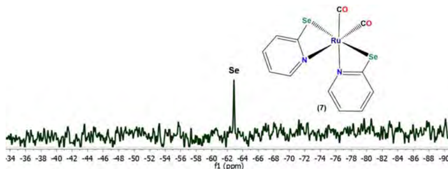
Figura 4.17. Espectro de RMN de ^{77}\text{Se}\{^1\text{H}\} de la reacción de C2 con DL3 . en acetona- \text{d}_6 a 25^\circ\text{C} .
