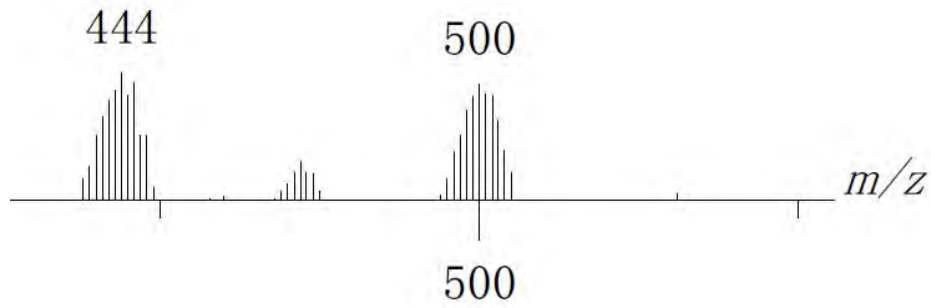
Espectro de masas del compuesto 7'.
