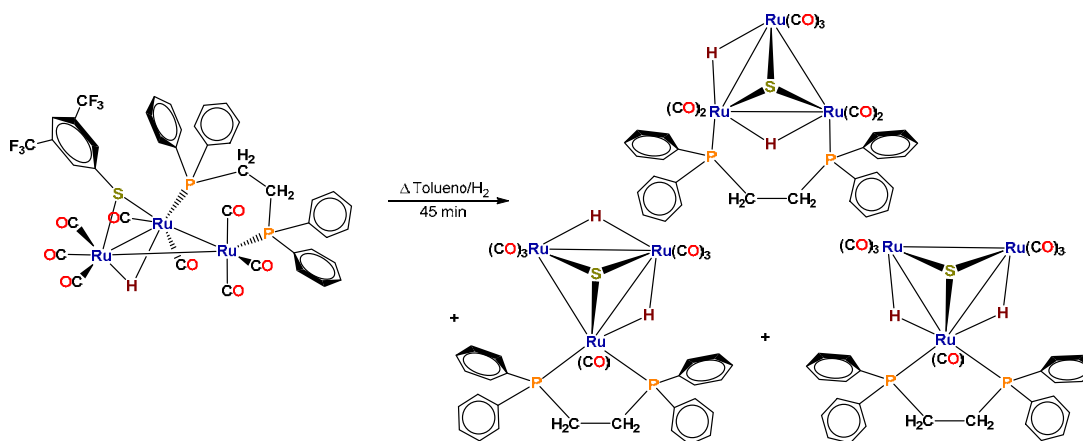
Esquema 1.16. Reacción para la síntesis de los cúmulos de fórmula general [Ru_3(\mu-H)_2(\mu_3-S)(\mu-dppe)(CO)_7] .
