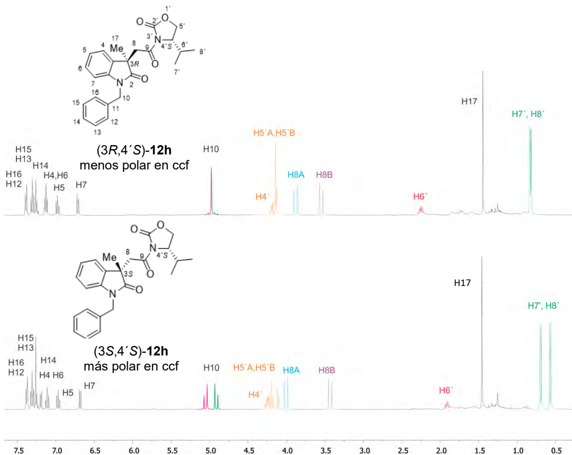
Figura 24. Espectros de RMN de ^1\text{H} a 400 MHz en \text{CDCl}_3 de las imidas diastereoisoméricas (3 R ,4' S )- y (3 S ,4' S )- 12h .
