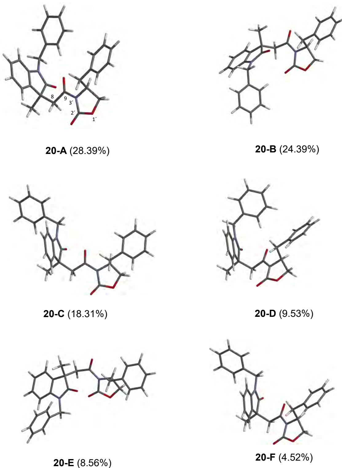
Figura 27. Estructuras de los 8 conformeros de menor energía del diastereoisómero (3 S ,4' S )- 20 obtenidos mediante cálculos DFT a un nivel de teoría B3LYP/DGDZVP.
