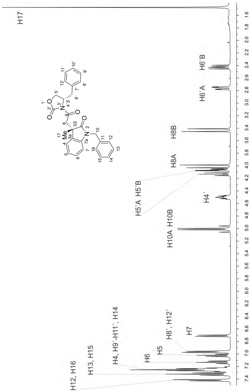
Figura 32. Espectro de RMN de ^1\text{H} de (3 S ,4' S )- 20 en \text{CDCl}_3 a 400 MHz.
