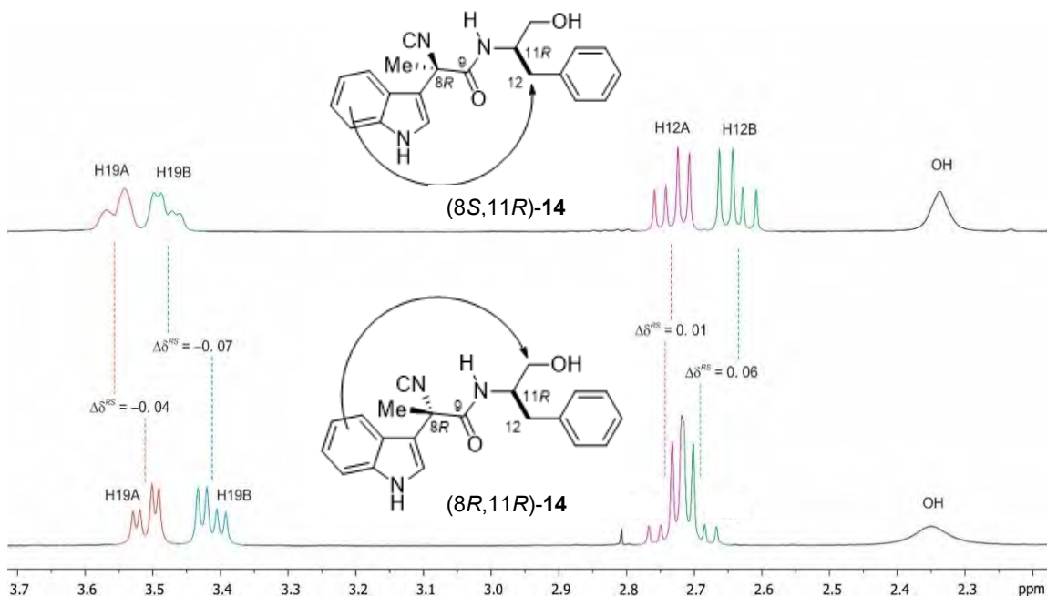
Figura 15. Espectros de RMN de ^1\text{H} de las amidas (8R,11R) - y (8S,11R) - 14 .
