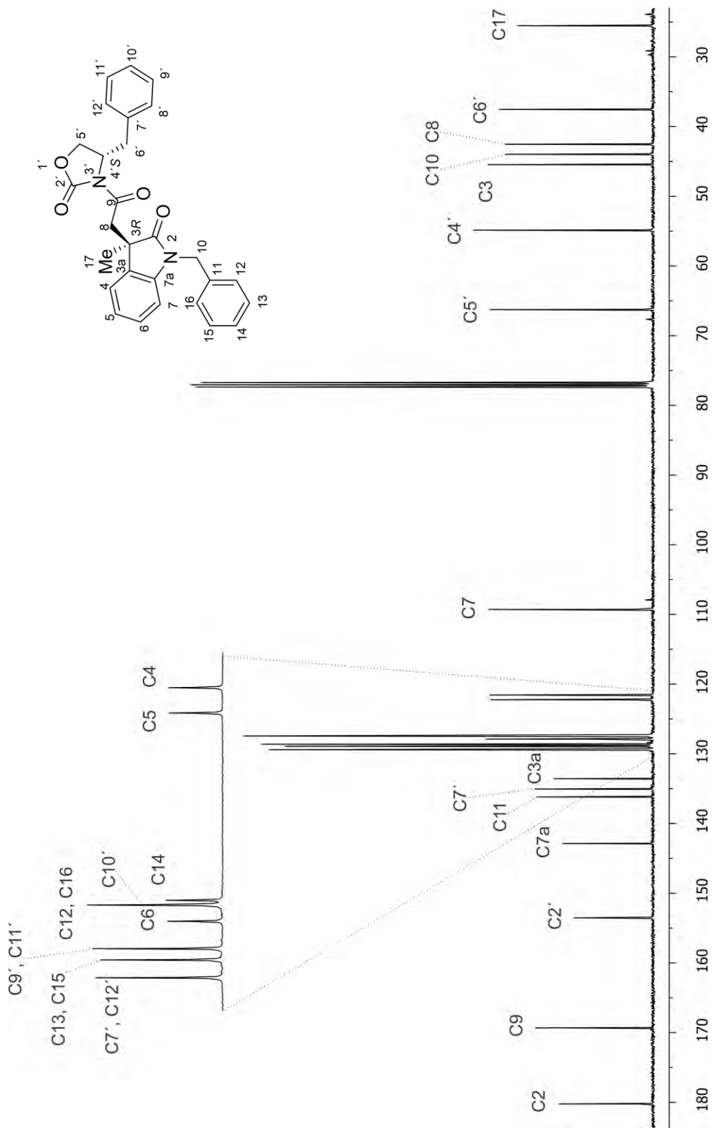
Figura 31. Espectro de RMN de ^{13}\text{C} de (3R,4'S)-20 en \text{CDCl}_3 a 100 MHz.
