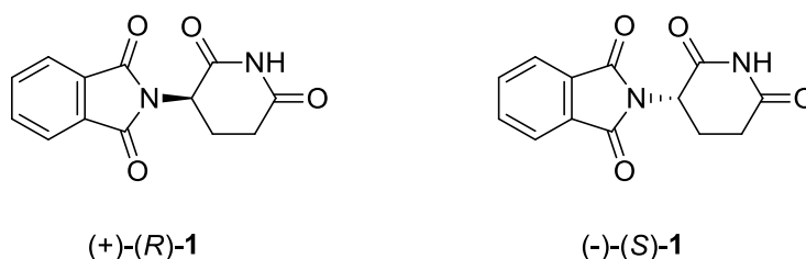
Figura 1. Enantiómeros de la ( \pm )-talidomida.
