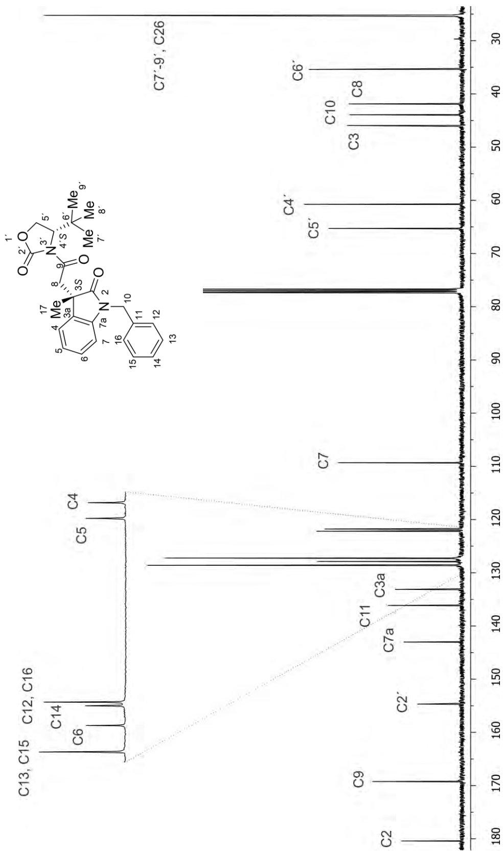
Figura 45. Espectro de RMN de ^{13}\text{C} de (3S,4'S)-23 en \text{CDCl}_3 a 100 MHz.
