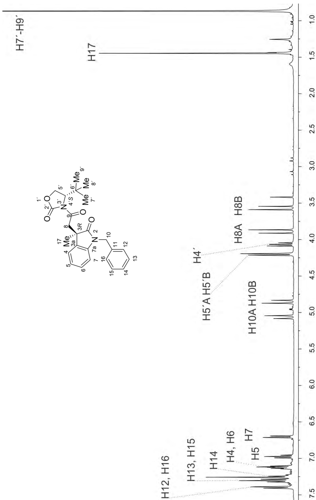
Figura 42. Espectro de RMN de 1 H de (3 R ,4' S )- 23 en CDCl 3 a 400 MHz.
