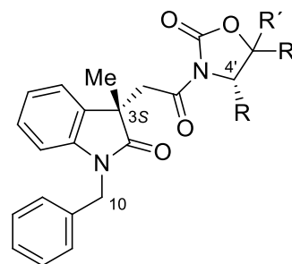
(3S,4'S)-20-24 más polar en ccf
