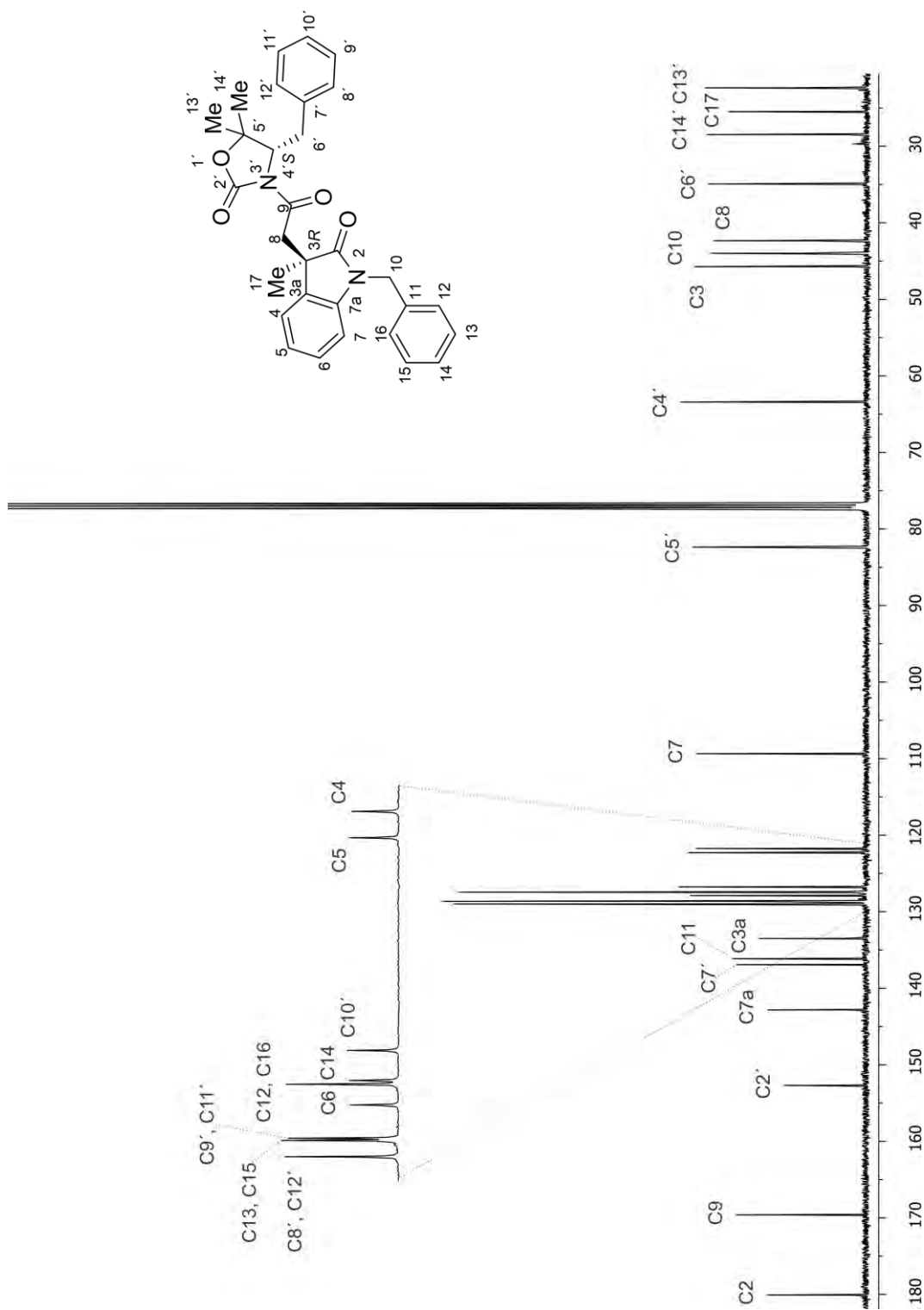
Figura 35. Espectro de RMN de ^{13}\text{C} de (3R,4'S)-21 en \text{CDCl}_3 a 100 MHz.
