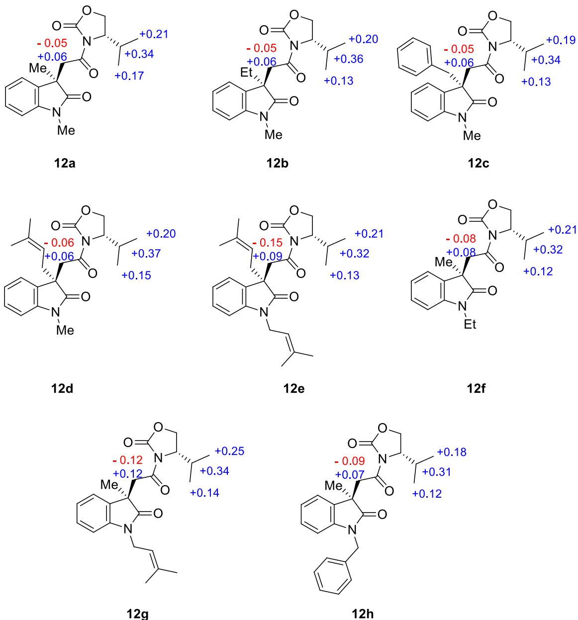
Figura 10. Diferencias de desplazamiento químico \Delta\delta^{RS} de las imidas (3 R ,4' S )- y (3 S ,4' S )- 12a-h
