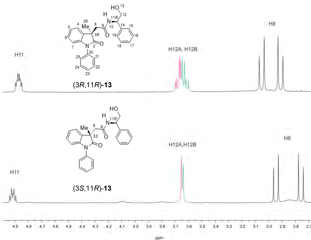
Figura 14. Espectros de RMN de ^1\text{H} de las amidas (3R,11R) - y (3S,11R) - 13 .
