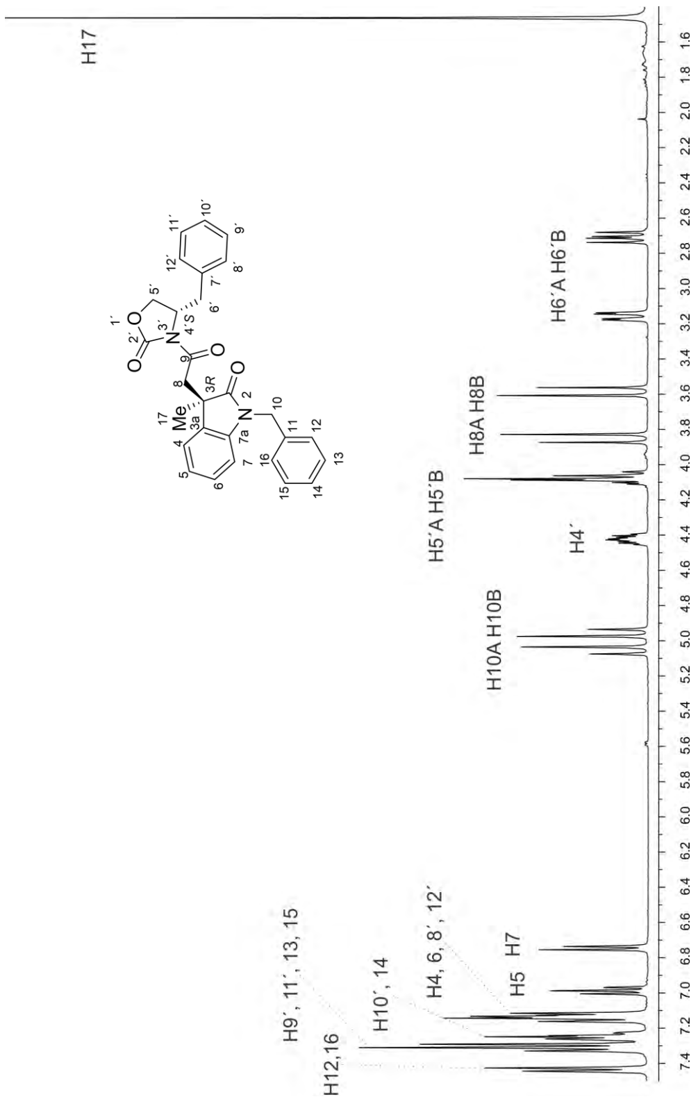
Figura 30. Espectro de RMN de ^1\text{H} de (3 R ,4' S )- 20 en \text{CDCl}_3 a 400 MHz.
