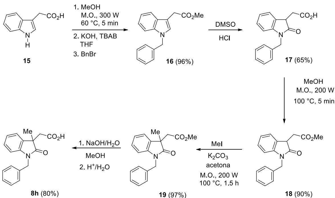
Esquema 3. Síntesis del ácido oxindolilacético 8h .
