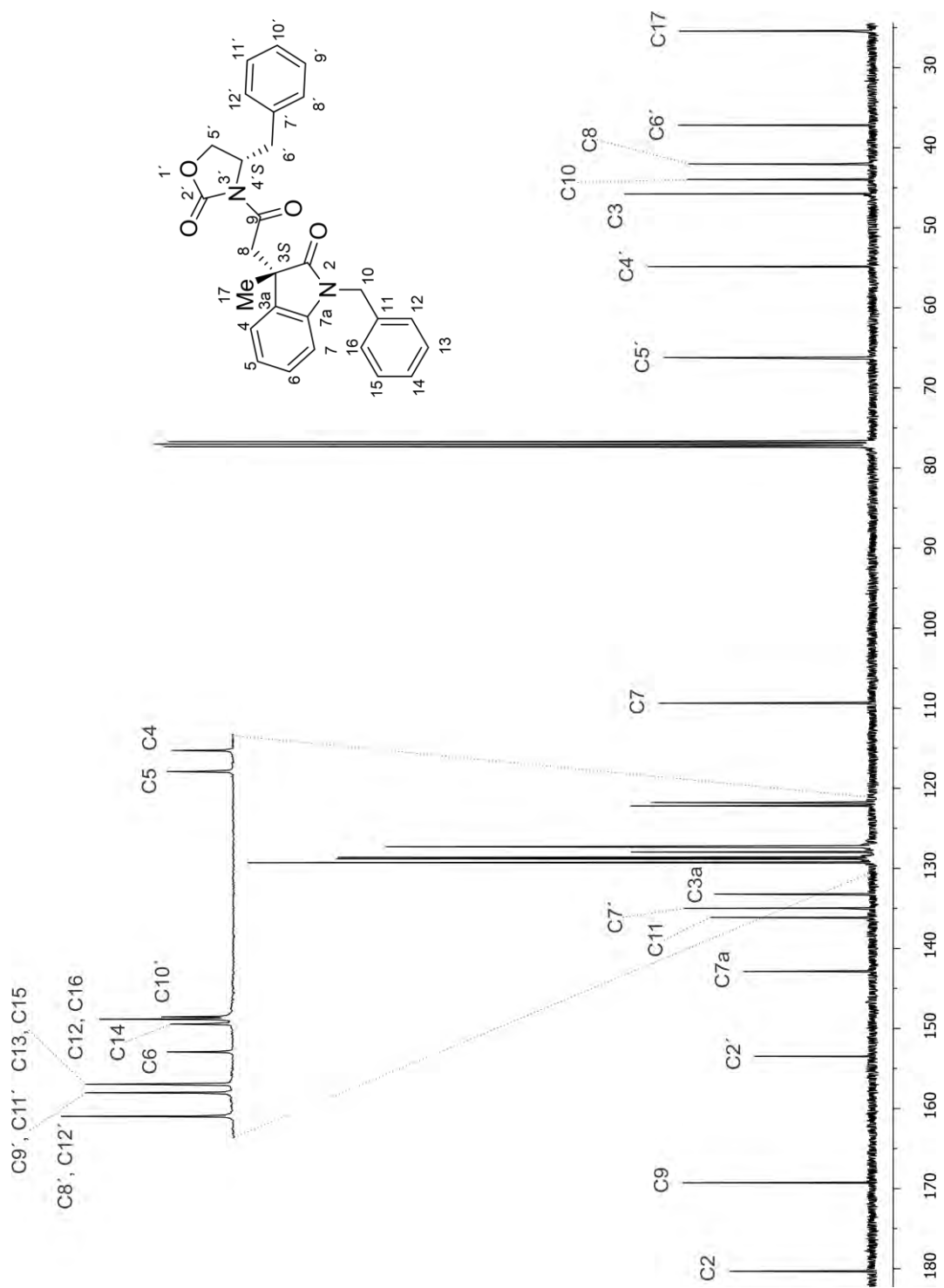
Figura 33. Espectro de RMN de 13 C de (3S,4'S)-20 en CDCl 3 a 100 MHz.
