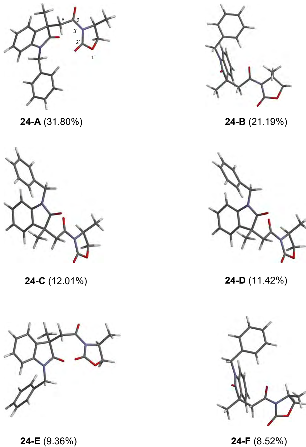
Figura 28. Estructuras de los 10 conformeros de menor energía del diastereoisómero (3 R ,4' S )- 24 obtenidos mediante cálculos DFT a un nivel de teoría B3LYP/DGDZVP.
