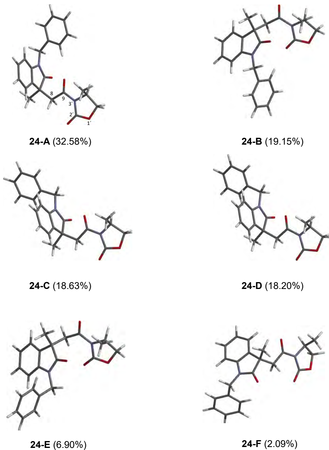
Figura 29. Estructuras de los 10 conformeros de menor energía del diastereoisómero (3S,4'S)- 24 obtenidos mediante cálculos DFT a un nivel de teoría B3LYP/DGDZVP.
