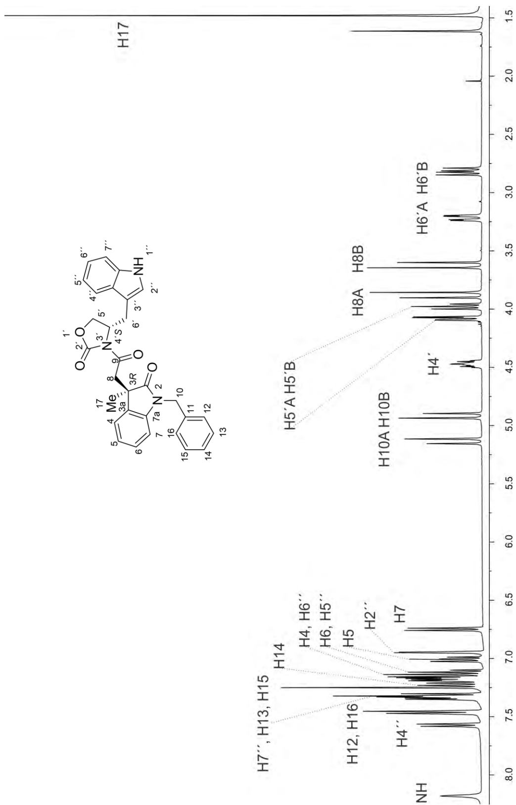
Figura 38. Espectro de RMN de ^1\text{H} de (3R,4'S)-22 en \text{CDCl}_3 a 400 MHz.
