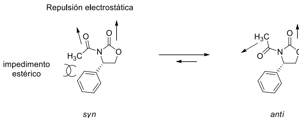
Esquema 5: Preferencia conformacional de oxazolidinonas N -carbonil sustituidas.
