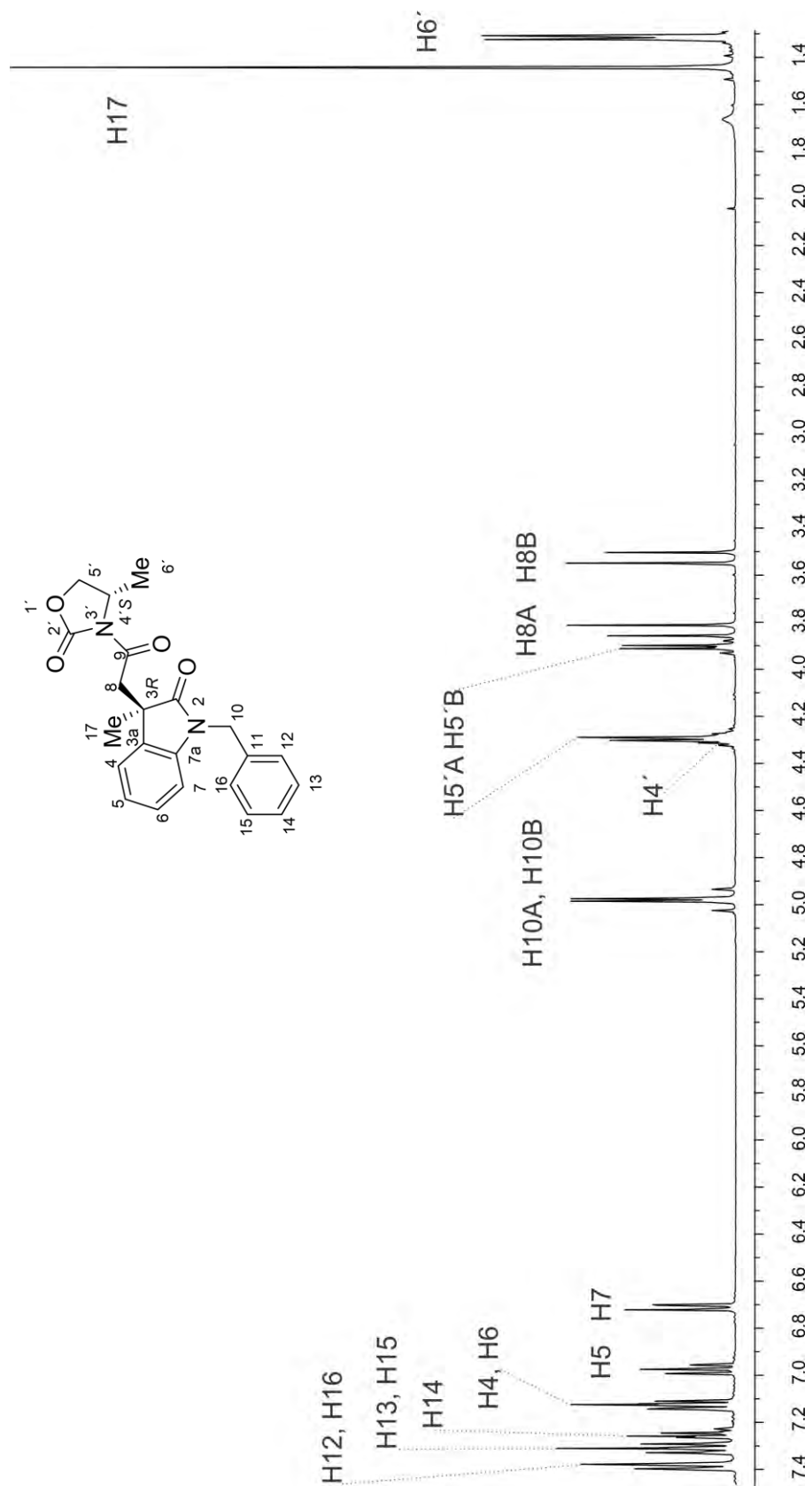
Figura 46. Espectro de RMN de ^1\text{H} de (3R,4'S)-24 en \text{CDCl}_3 a 400 MHz.
