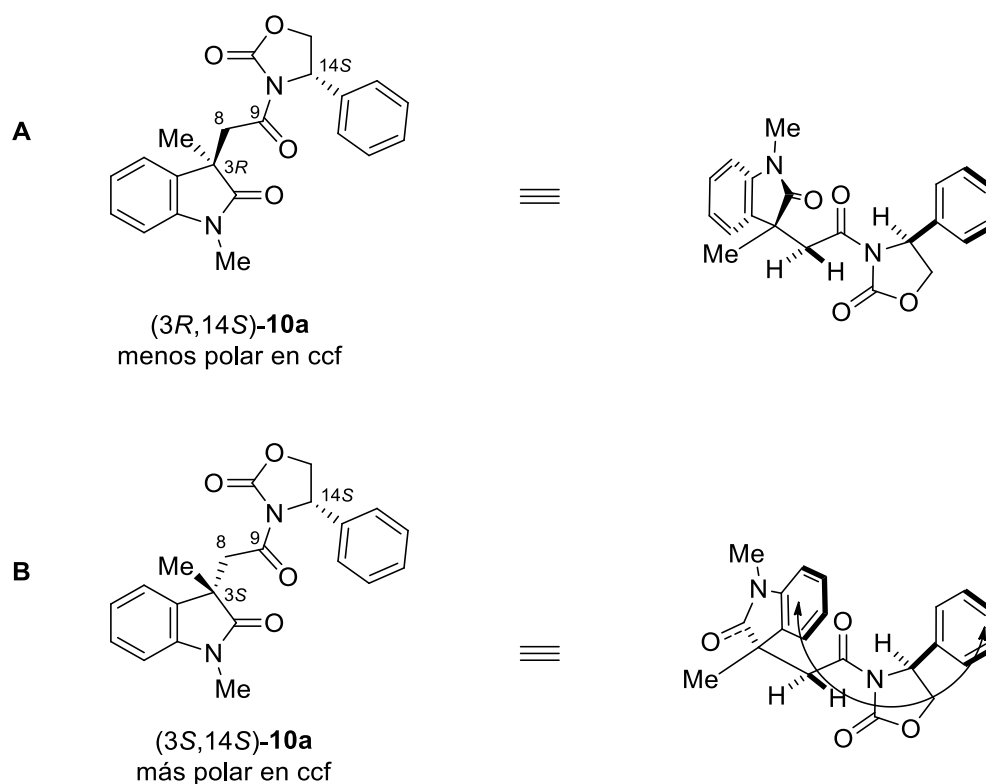
Figura 8. Modelo conformacional empírico propuesto para las imidas (3R,14S)- y (3S,14S)- 10a .
