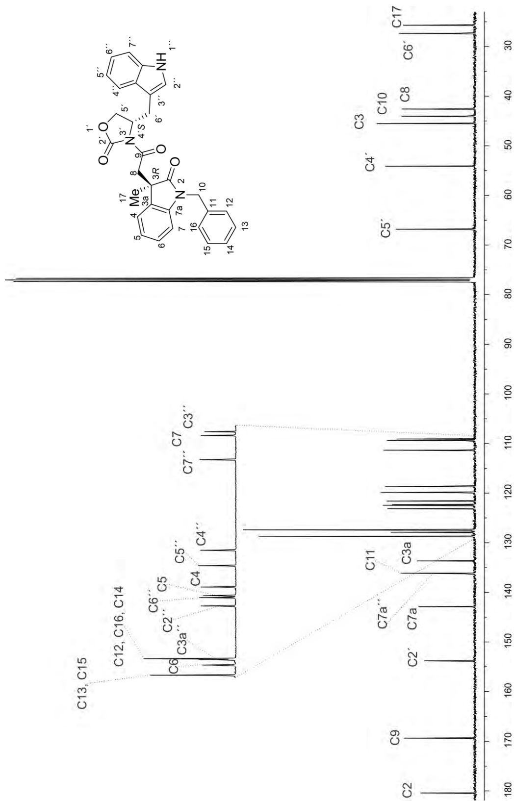
Figura 39. Espectro de RMN de ^{13}\text{C} de (3R,4'S)-22 en \text{CDCl}_3 a 100 MHz.
