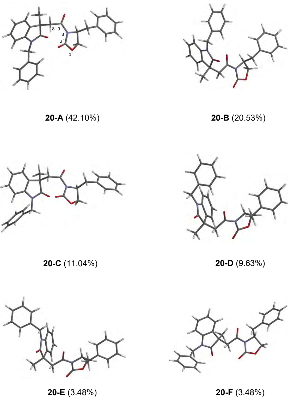
Figura 26. Estructuras de los 10 conformeros de menor energía del diastereoisómero (3 R ,4' S )- 20 obtenidos mediante cálculos DFT a un nivel de teoría B3LYP/DGDZVP.
