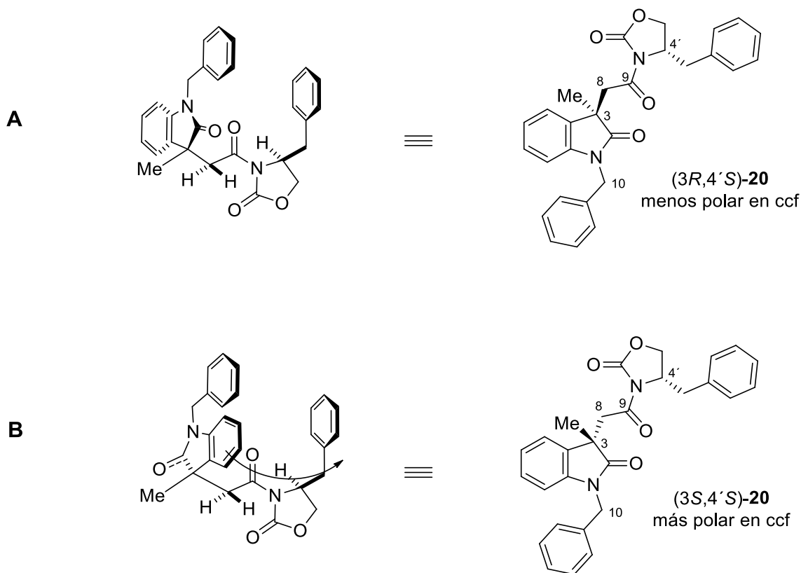
Figura 23. Modelos conformacionales empíricos propuestos para las imidas (3 R ,4' S )- y (3 S ,4' S )- 20 .
