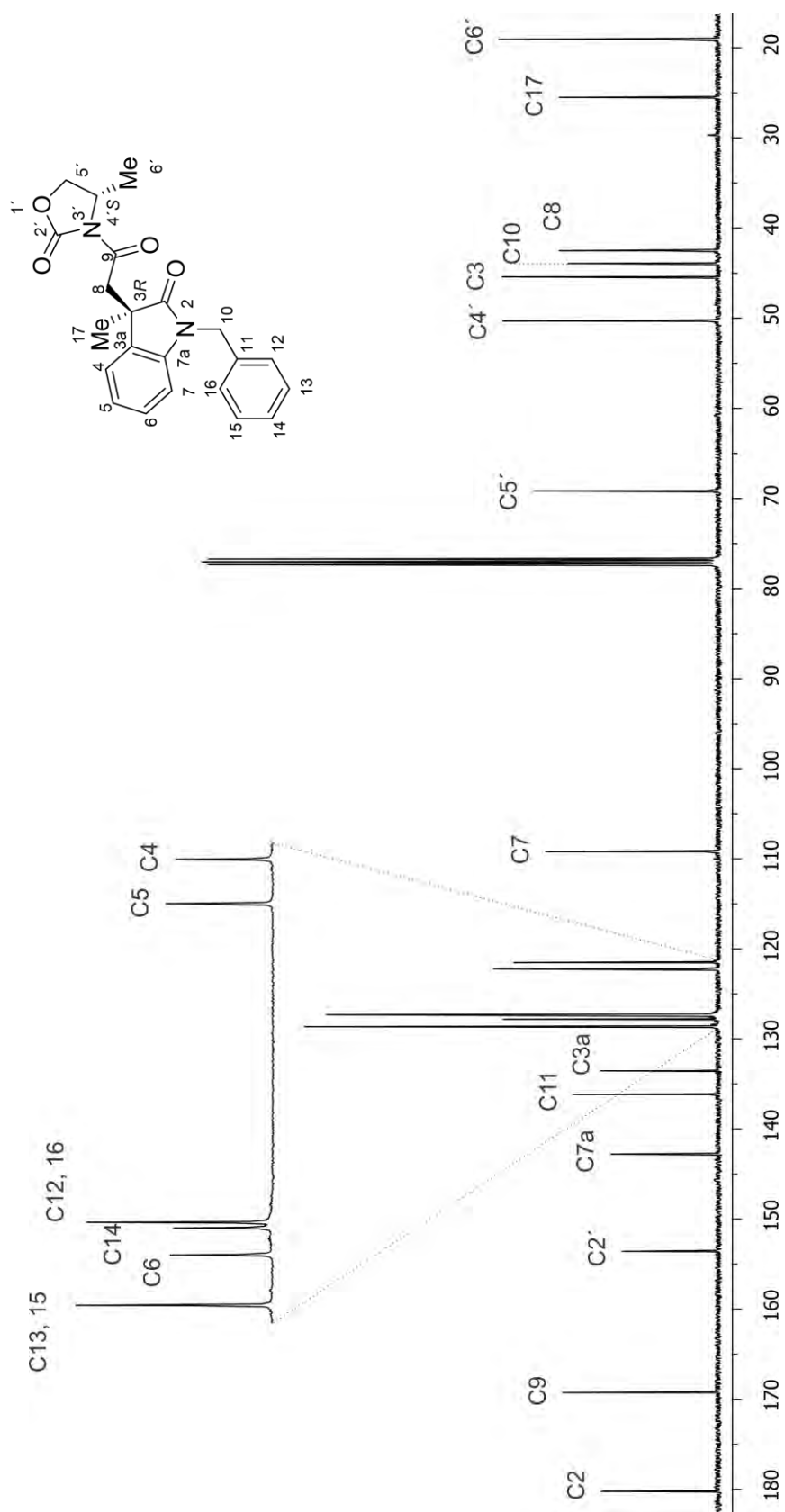
Figura 47. Espectro de RMN de ^{13}\text{C} de (3R,4'S)-24 en \text{CDCl}_3 a 100 MHz.
