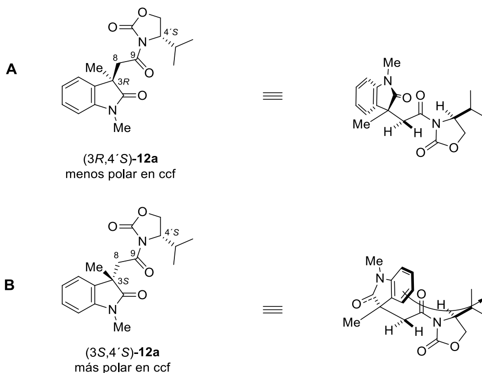
Figura 12. Modelo conformacional empírico propuesto para cada imida (3 R ,4' S )- y (3 S ,4' S )- 12a .
