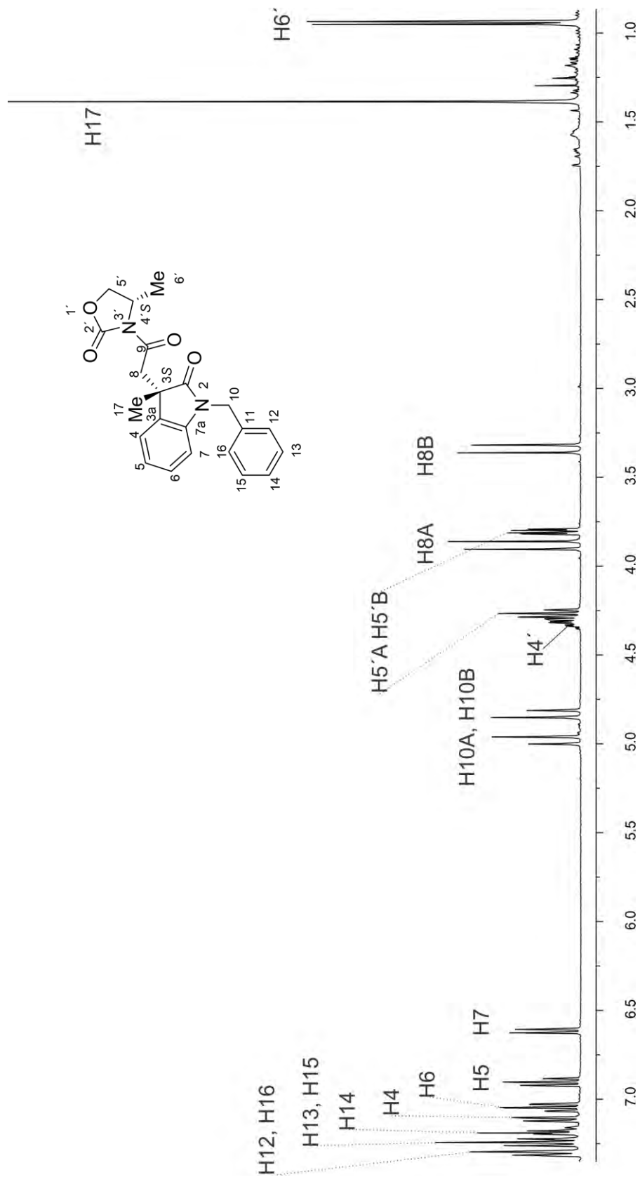
Figura 48. Espectro de RMN de ^1\text{H} de (3 S ,4' S )- 24 en \text{CDCl}_3 a 400 MHz.
