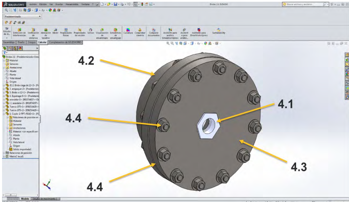
Fig. 71. Subensamle de bridas y accesorios.
