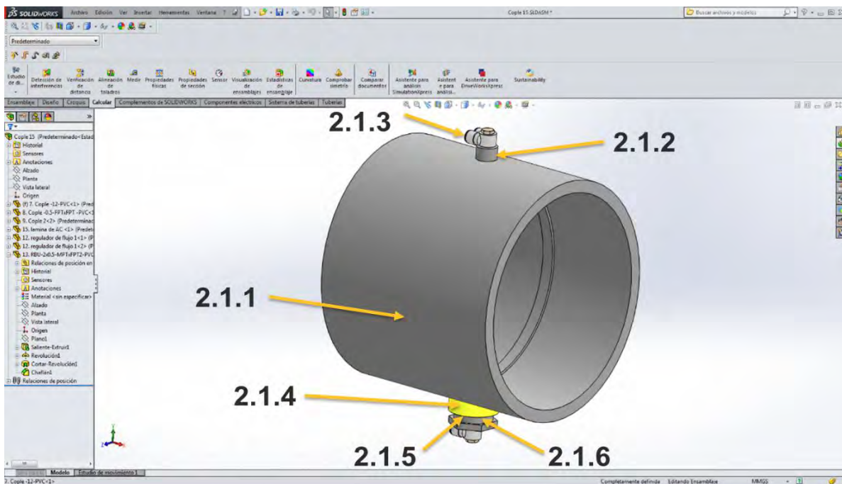
Fig. 68. Subensamble de coples y accesorios.
