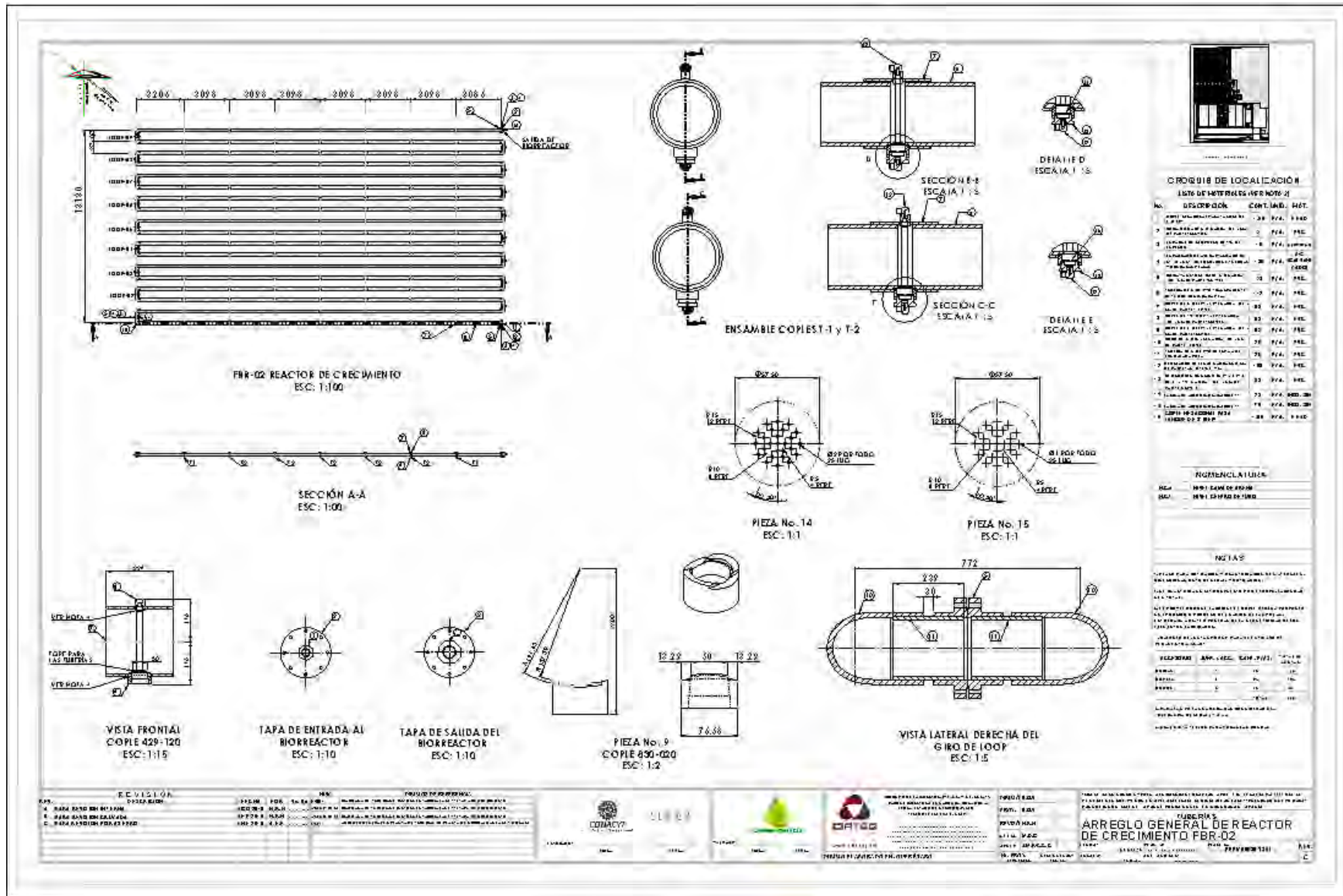
Fig. 87 Plano de construcción del fotobiorreactor de 8", con accesorios parametrizados.
