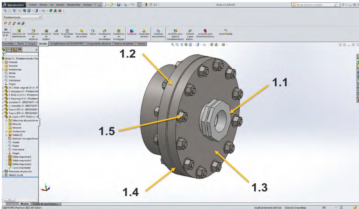
Fig. 67 Subensamble de bridas.
